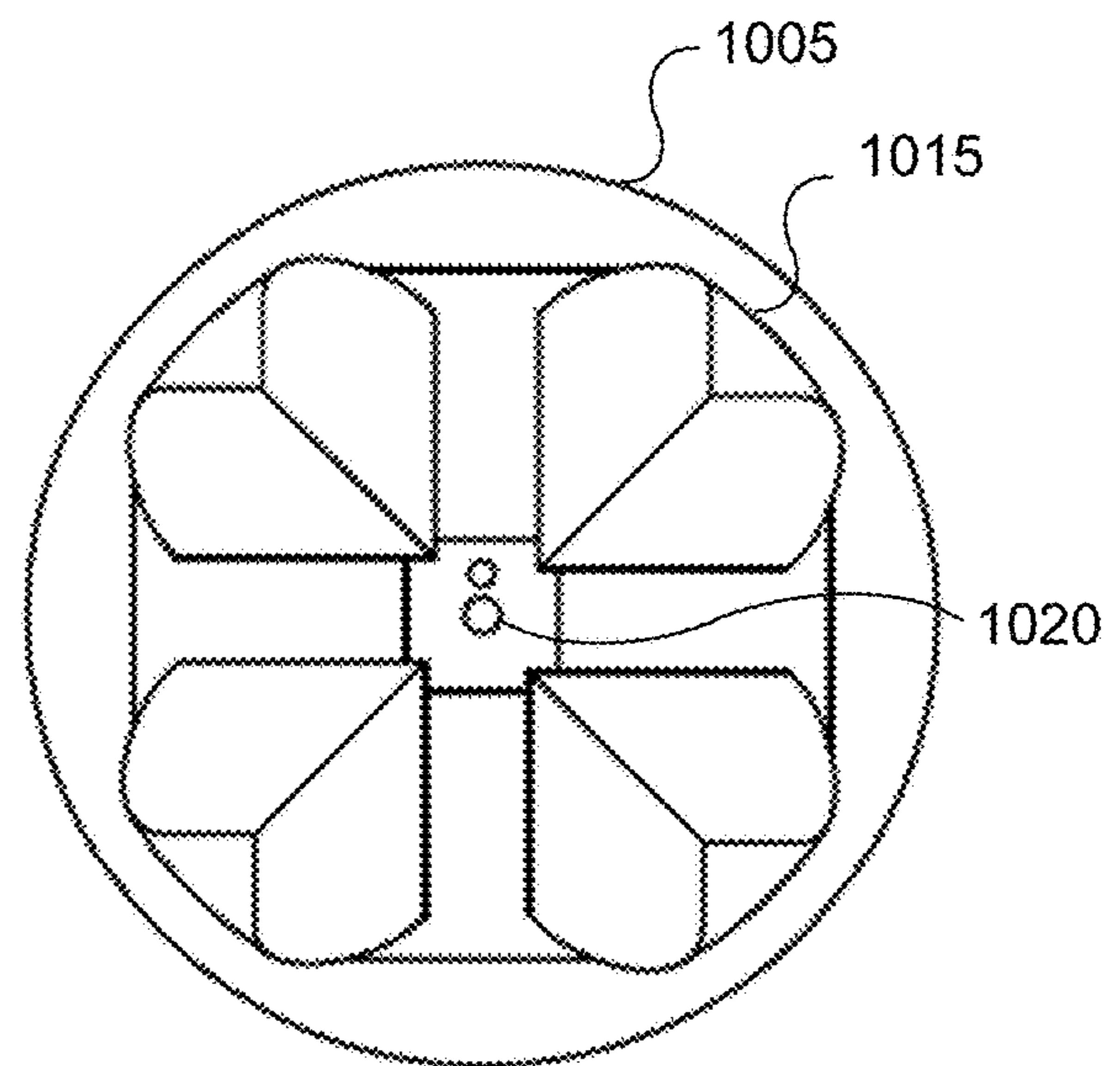
FIG. 10D
