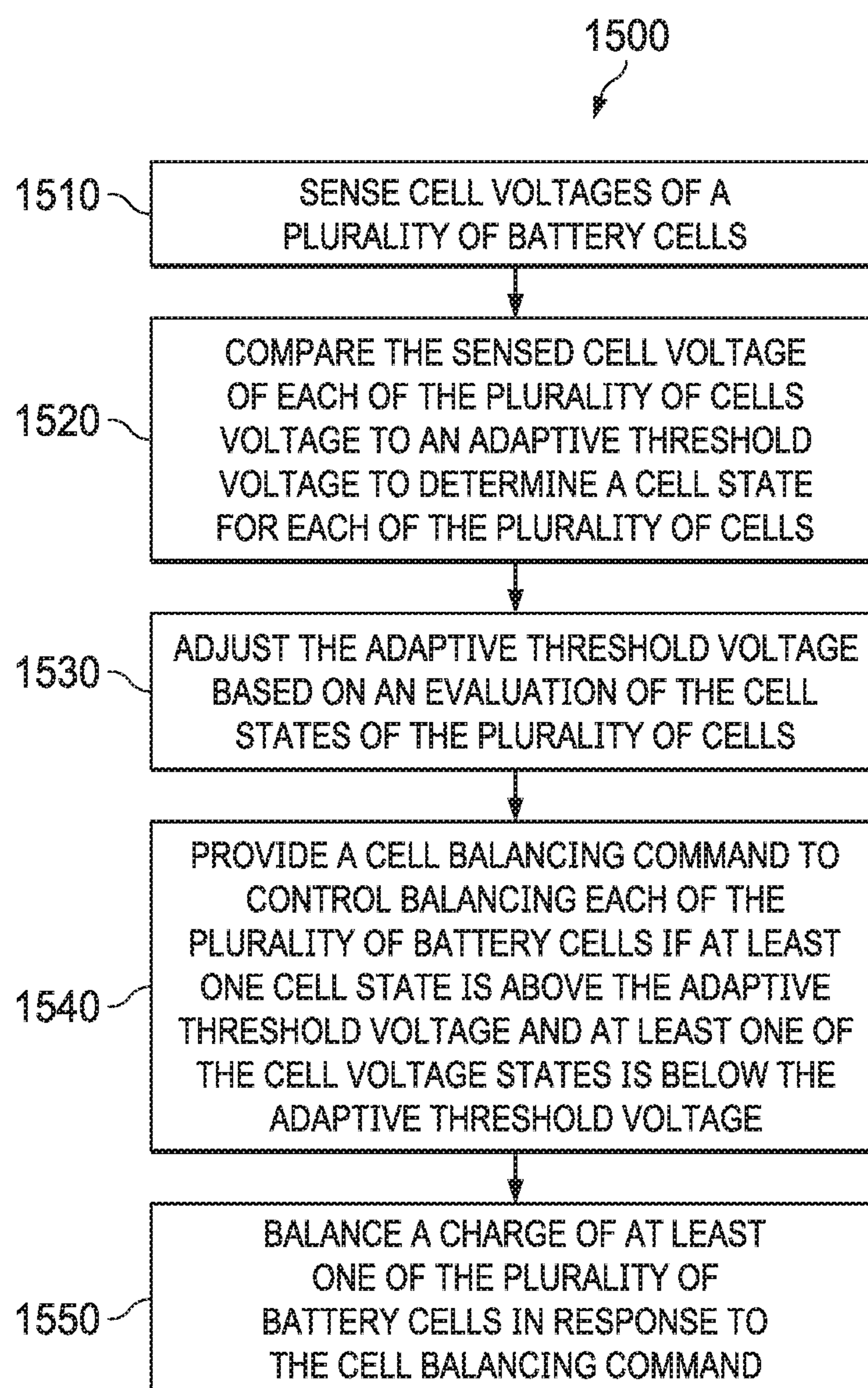
FIG. 15
