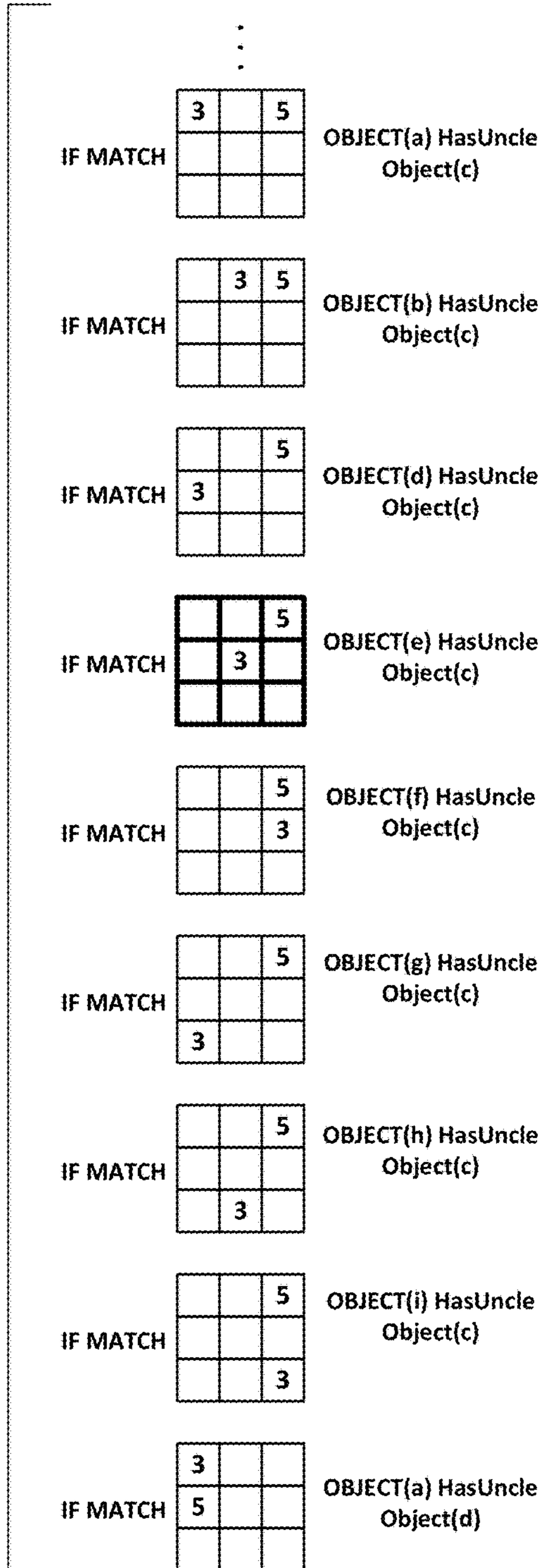
FIG. 26 – PREDICATE TEMPLATES
