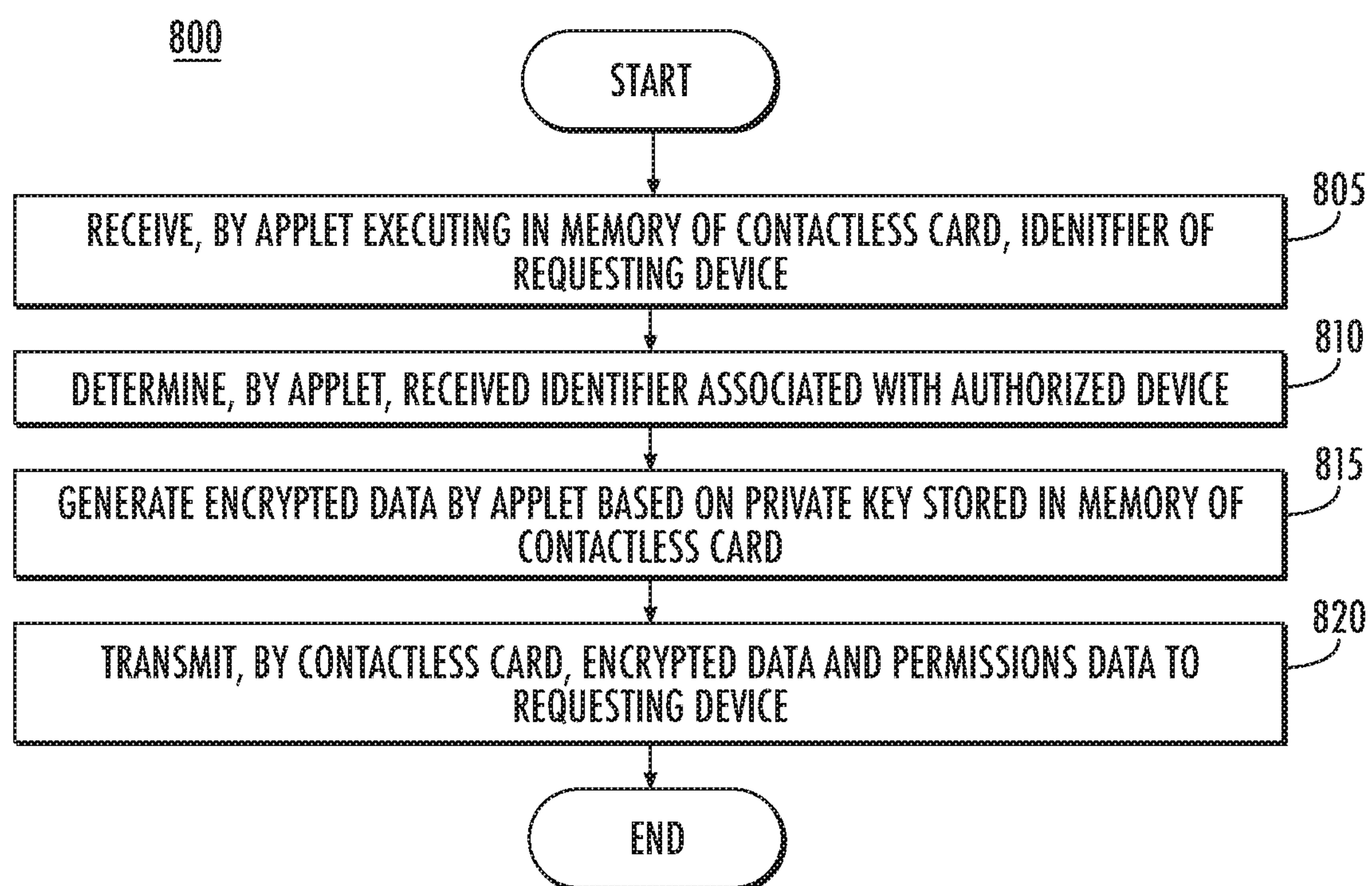
FIG. 8
