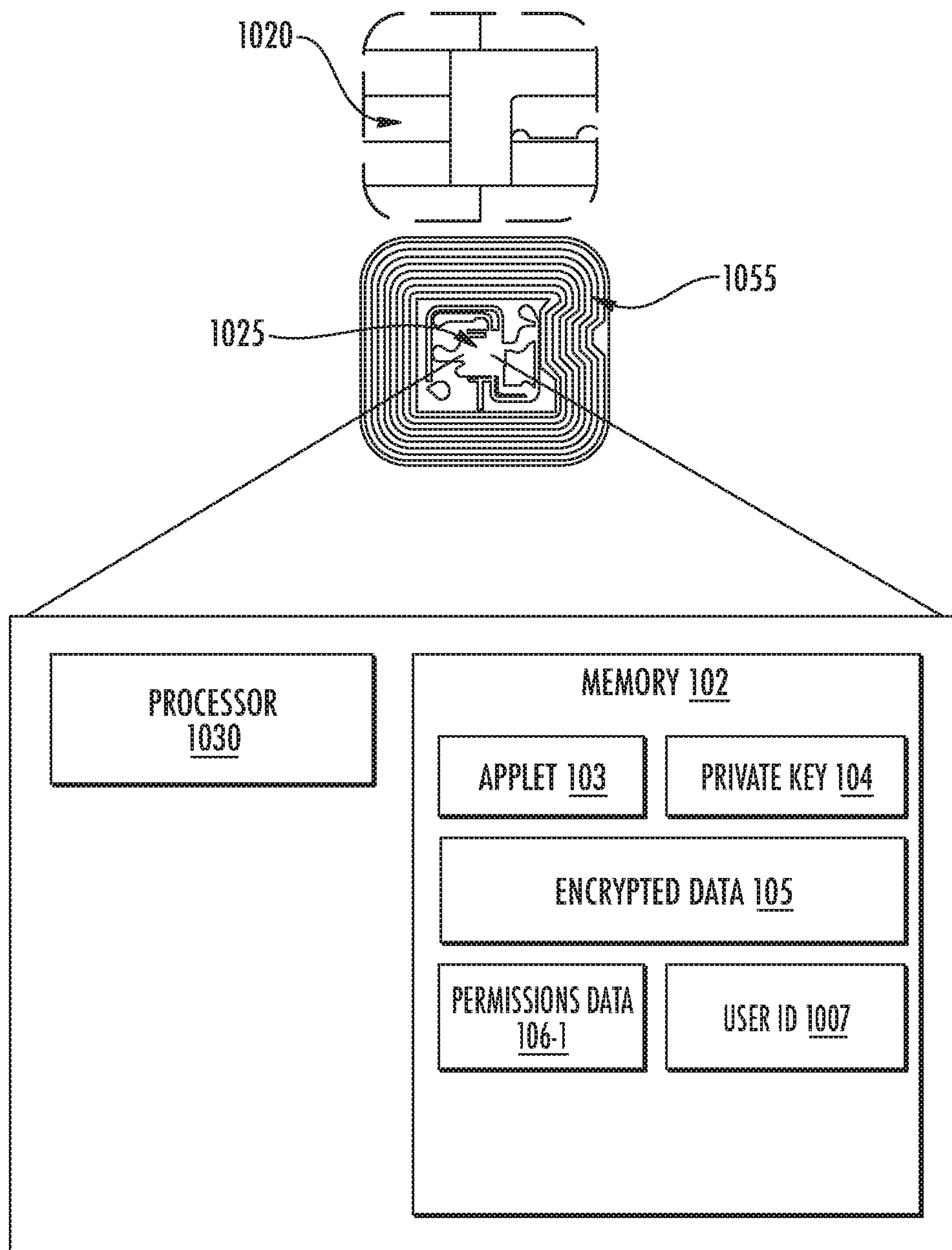
FIG. 10B
