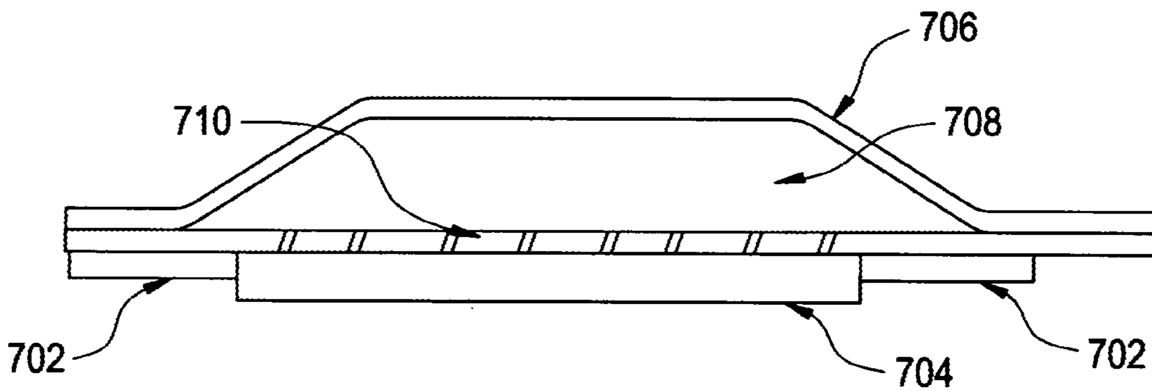
FIG. 7C Section A-A
