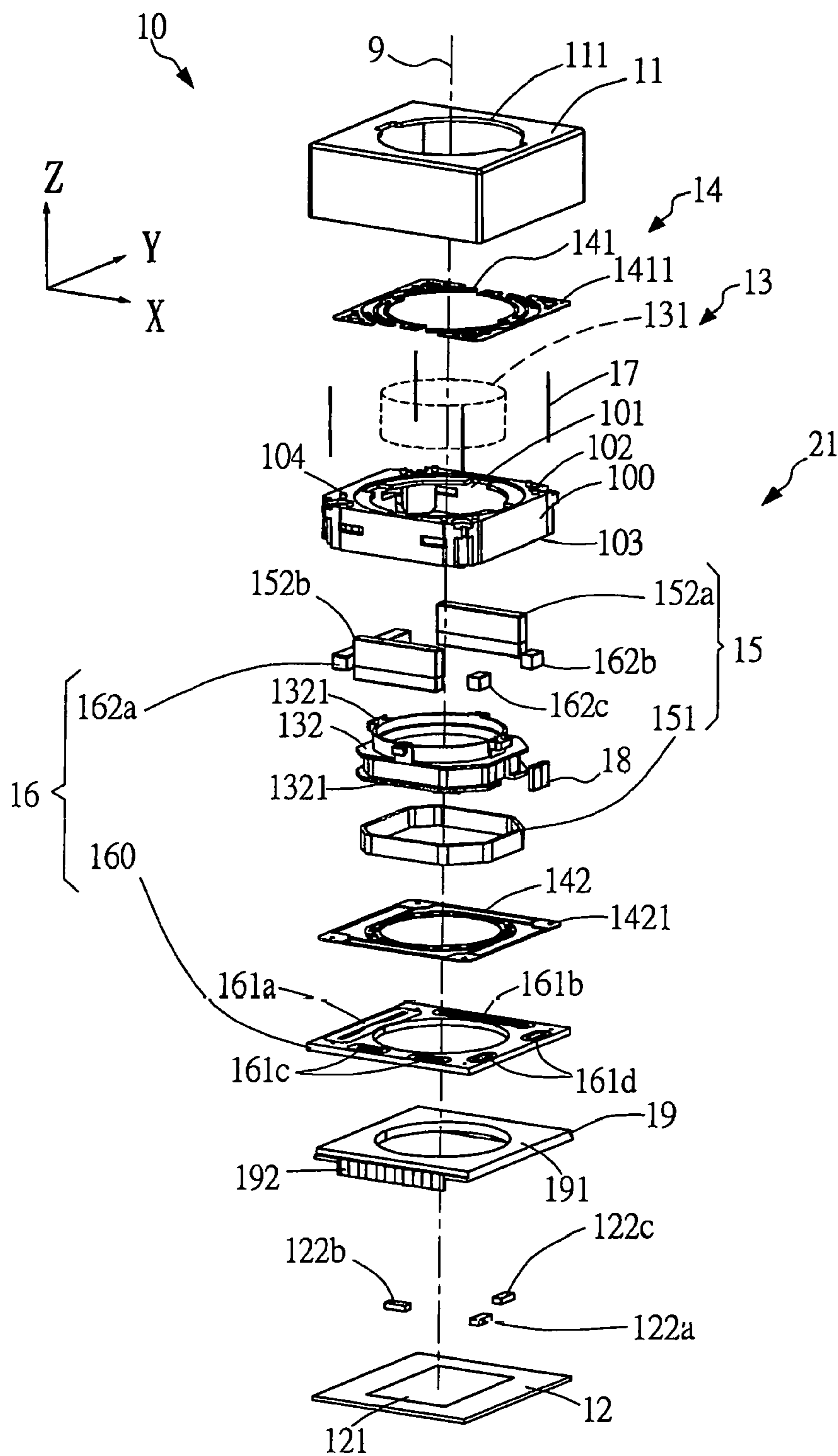
FIG.4A
