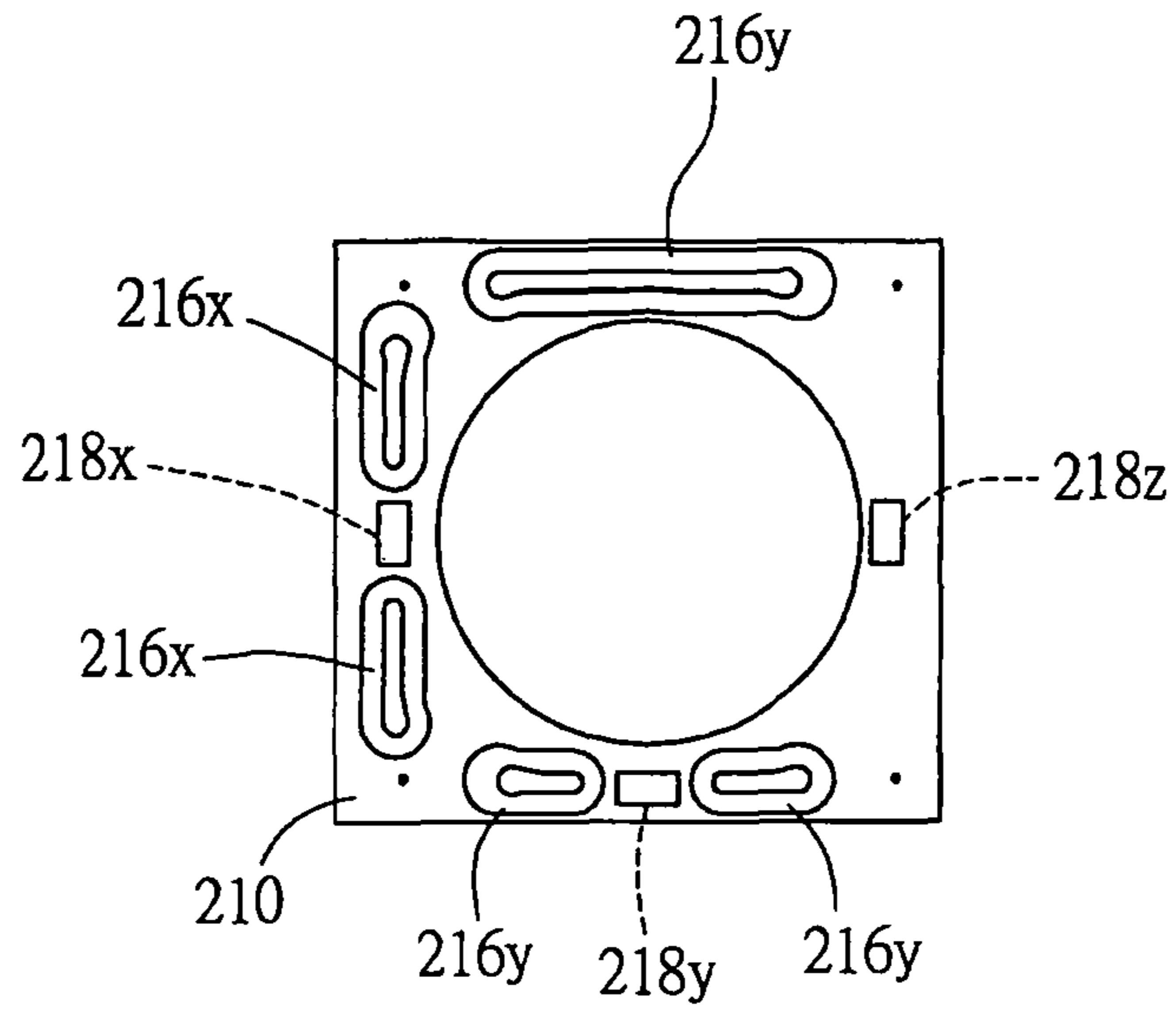
FIG.7A
