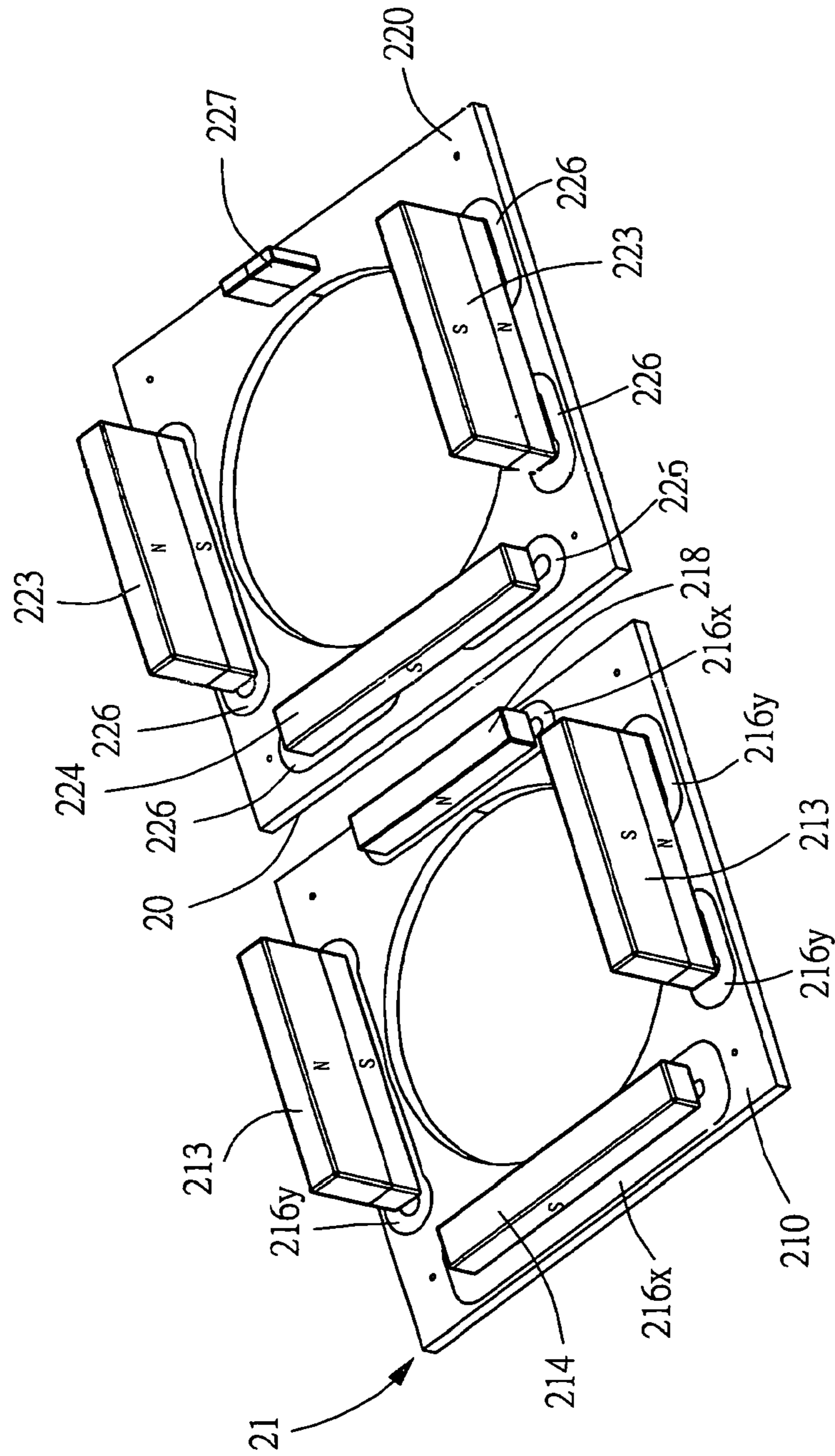
FIG.16
