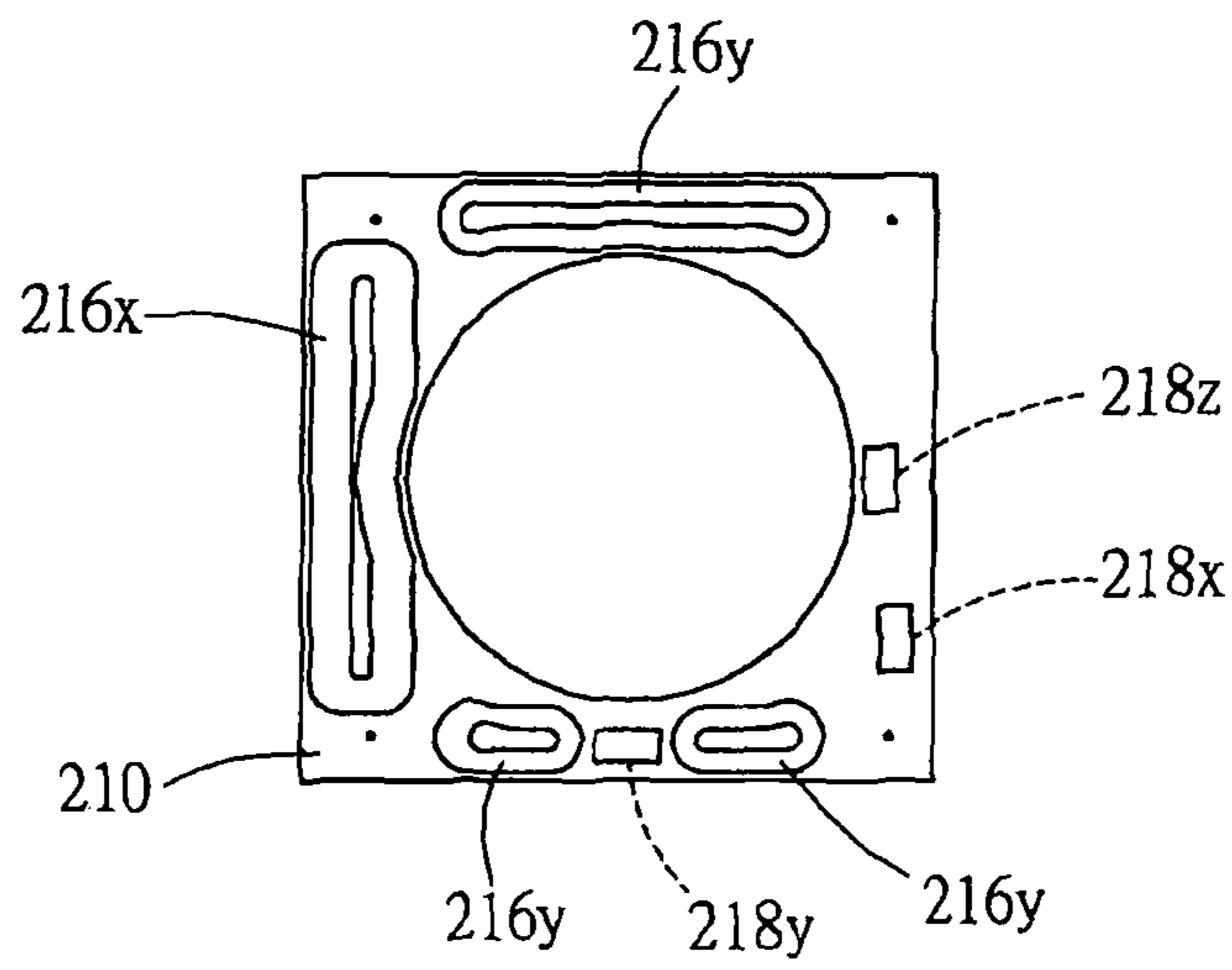
FIG. 11B
