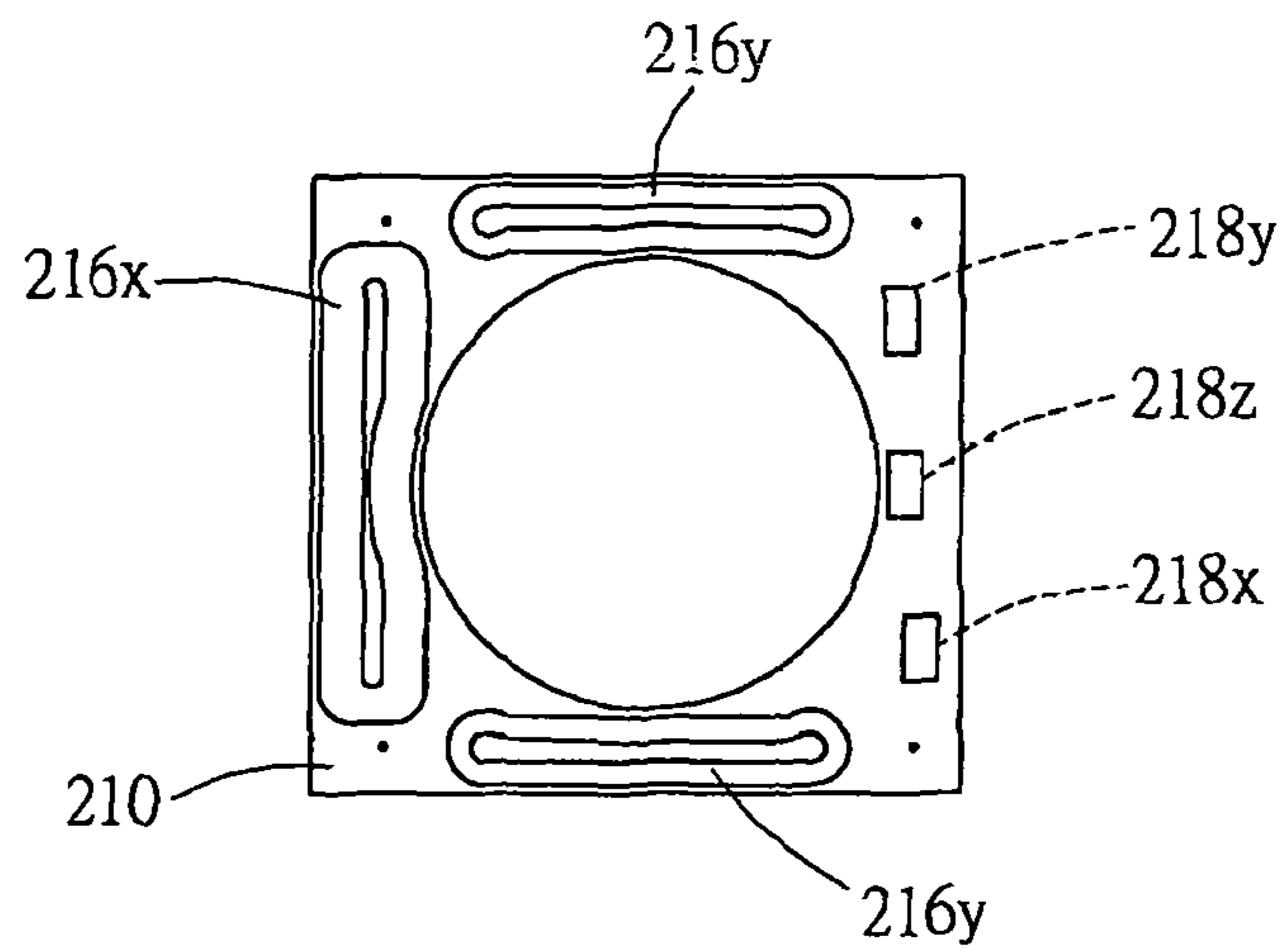
FIG. 11B
