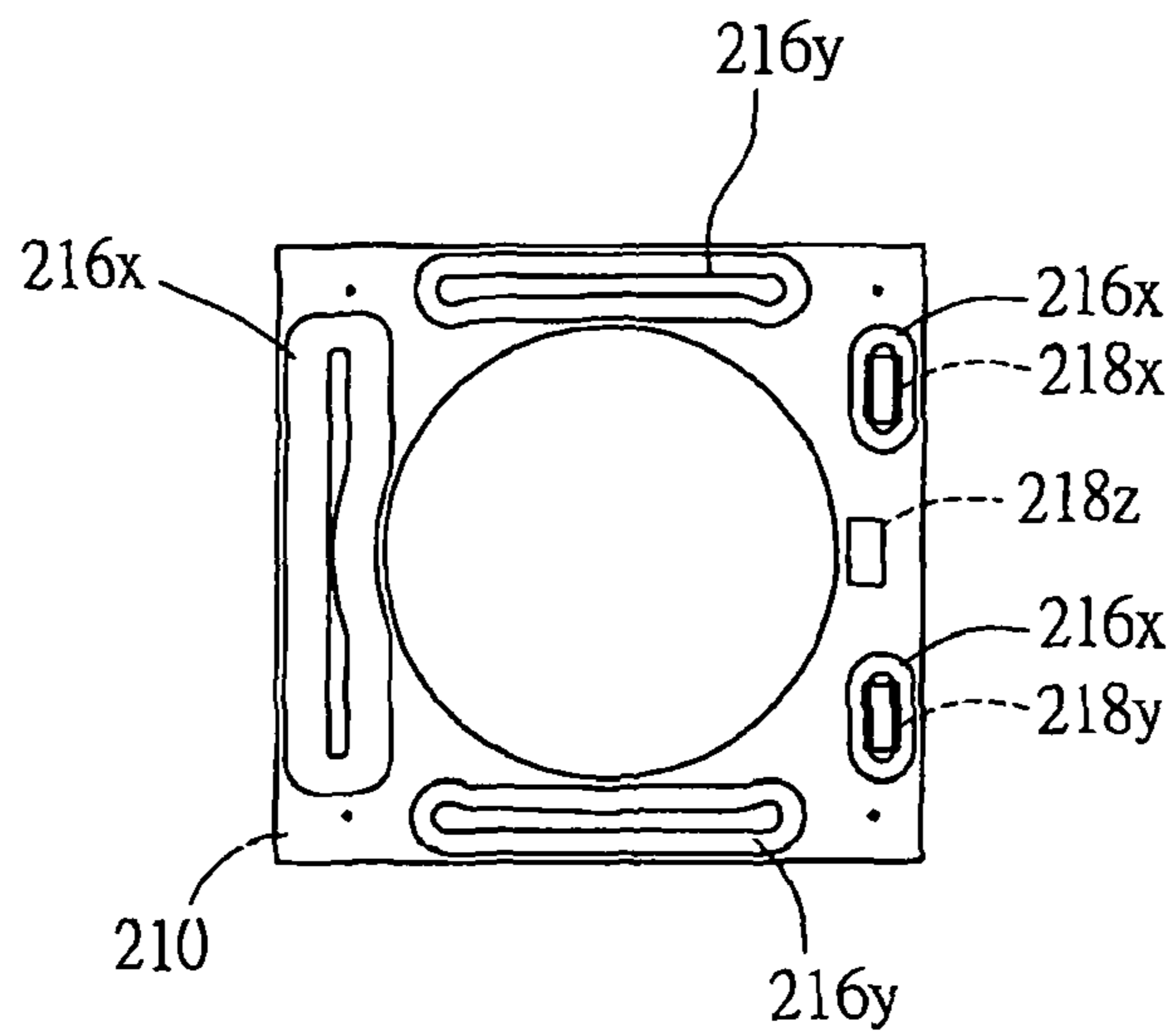
FIG. 7D
