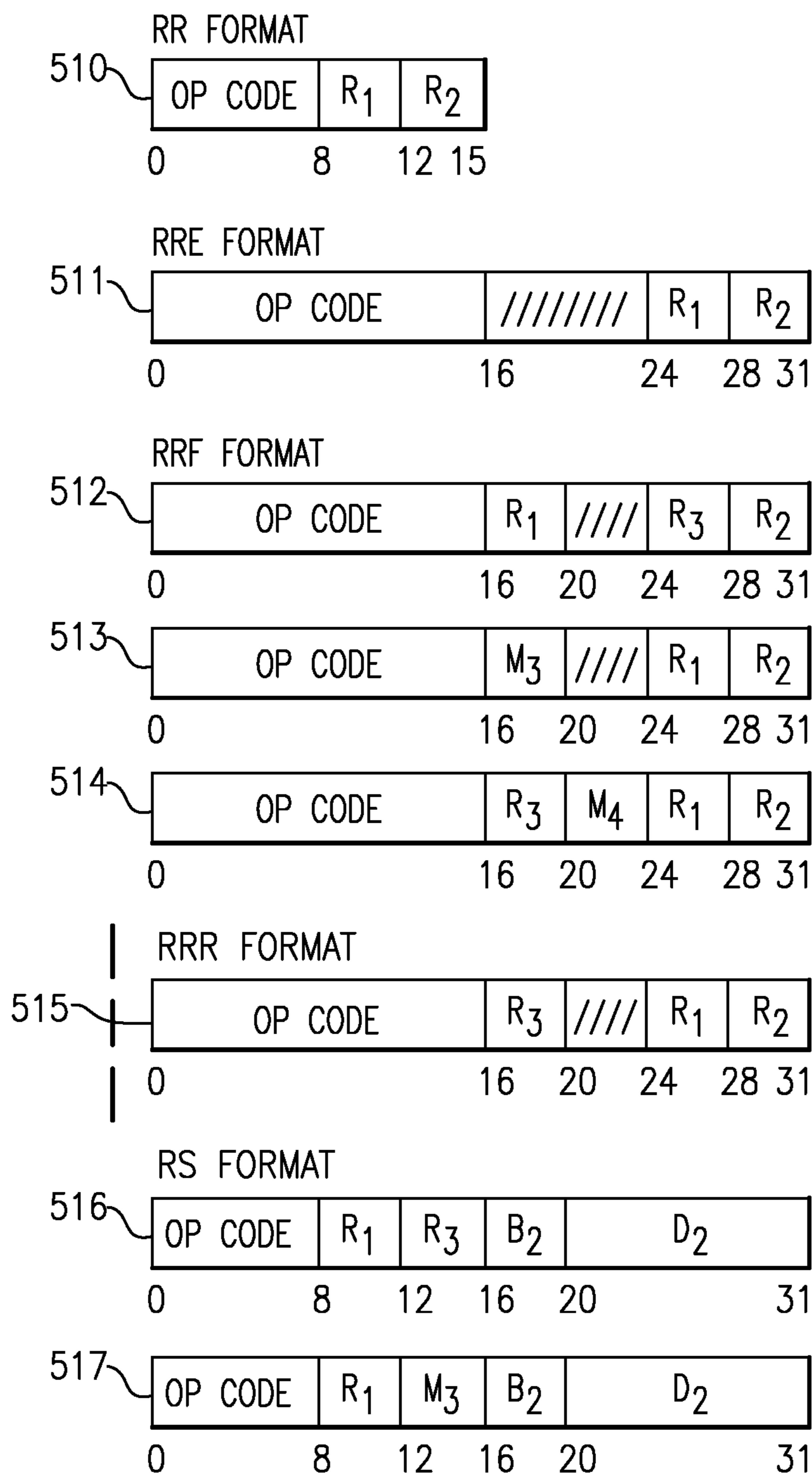
FIG.5B
