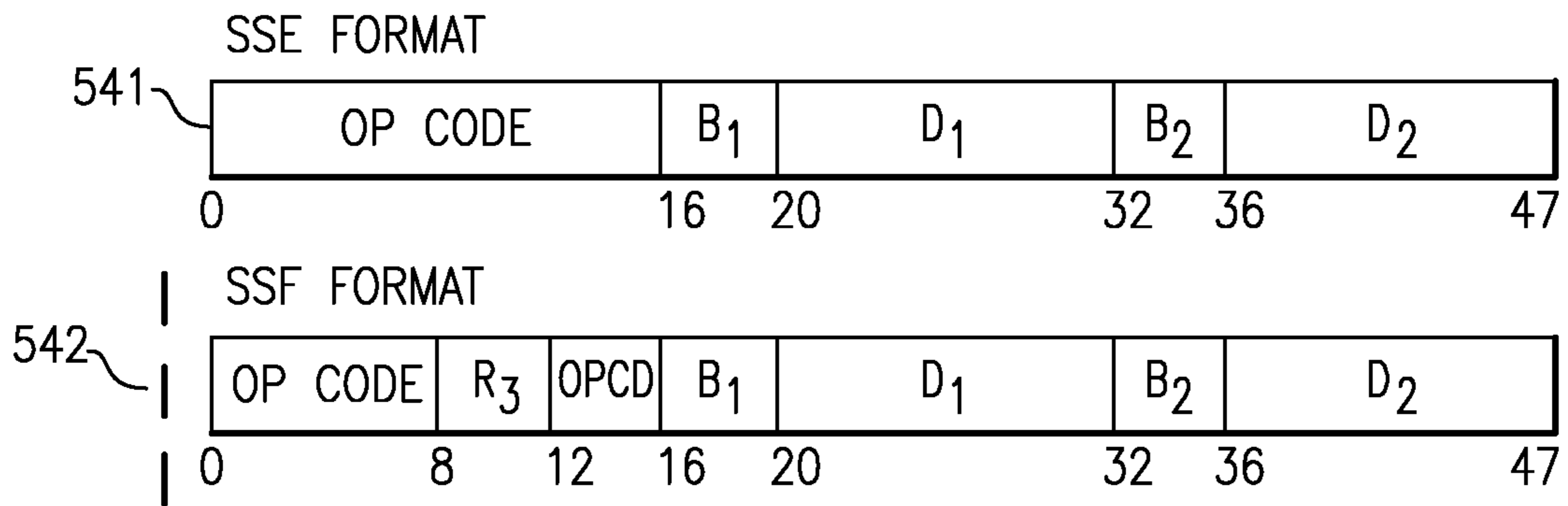
FIG.5E
