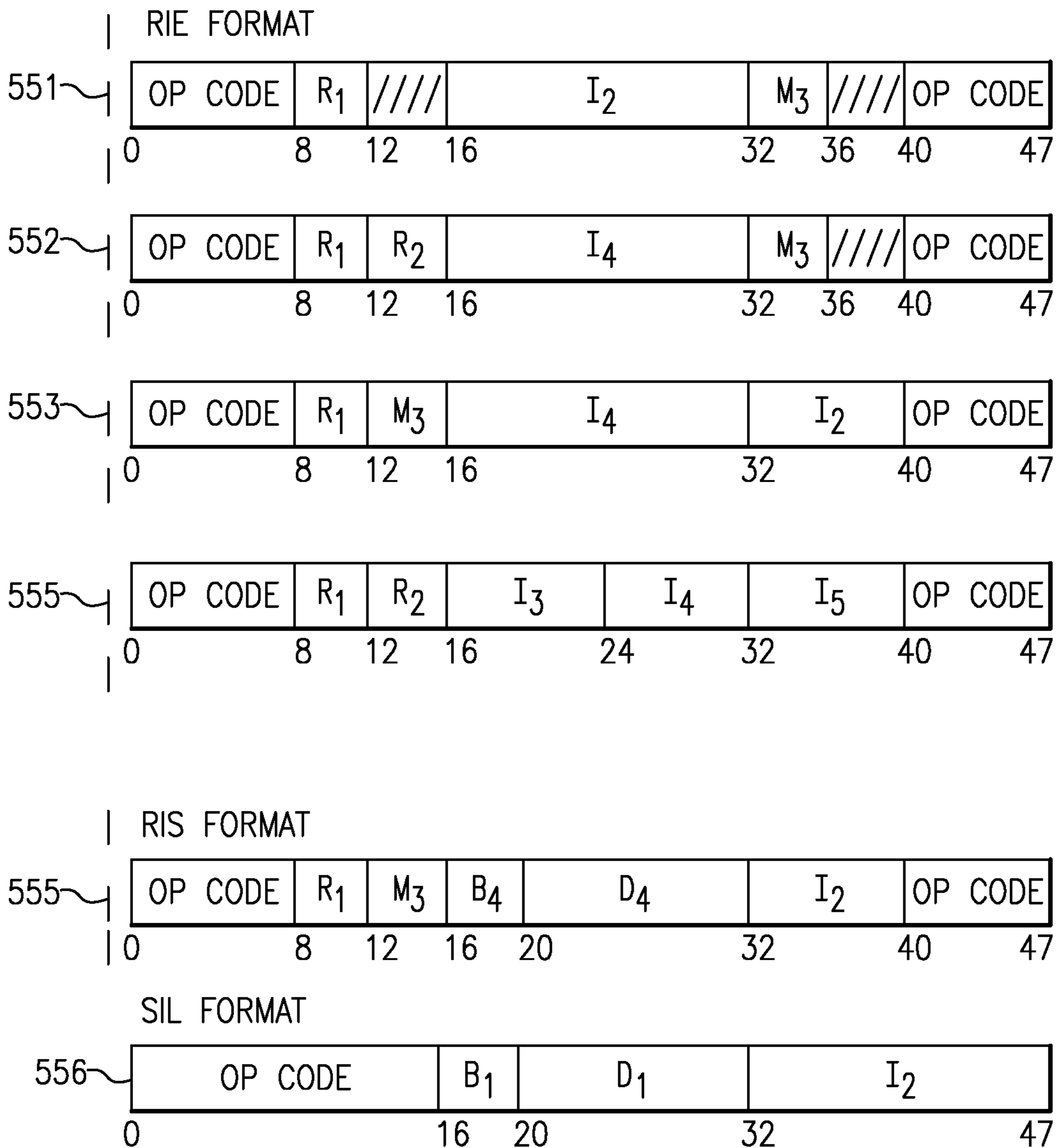
FIG.5F
