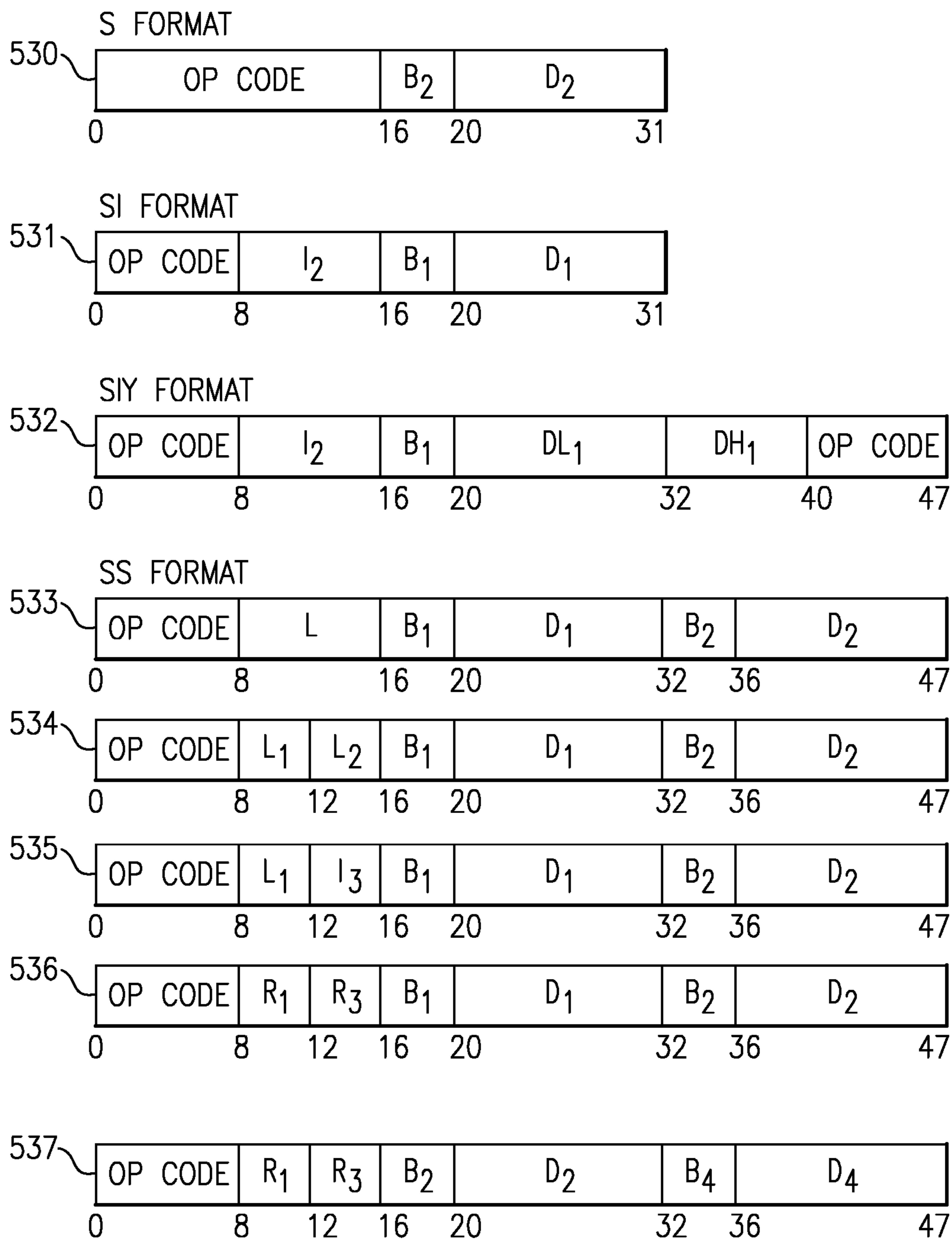
FIG.5D
