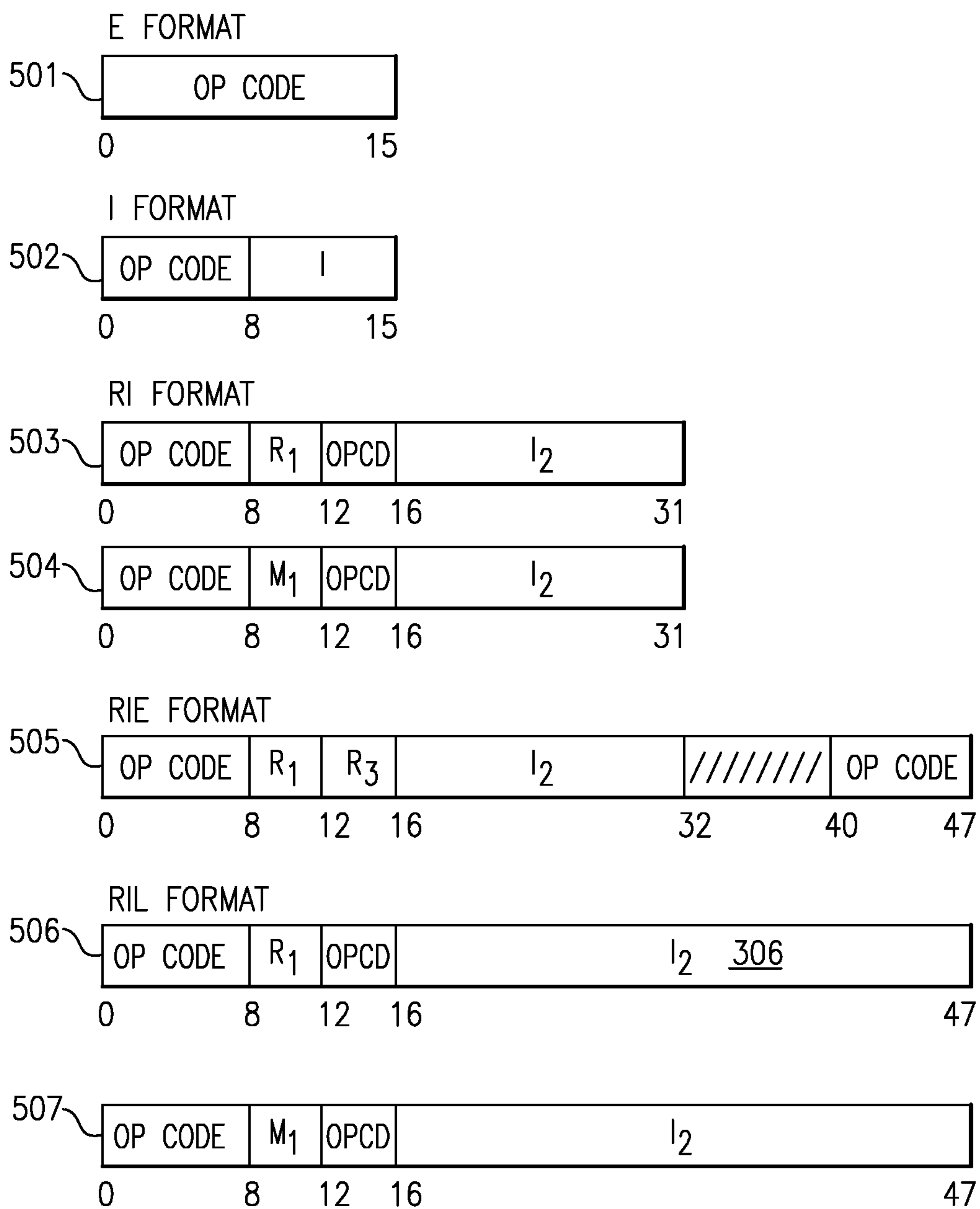
FIG.5A
