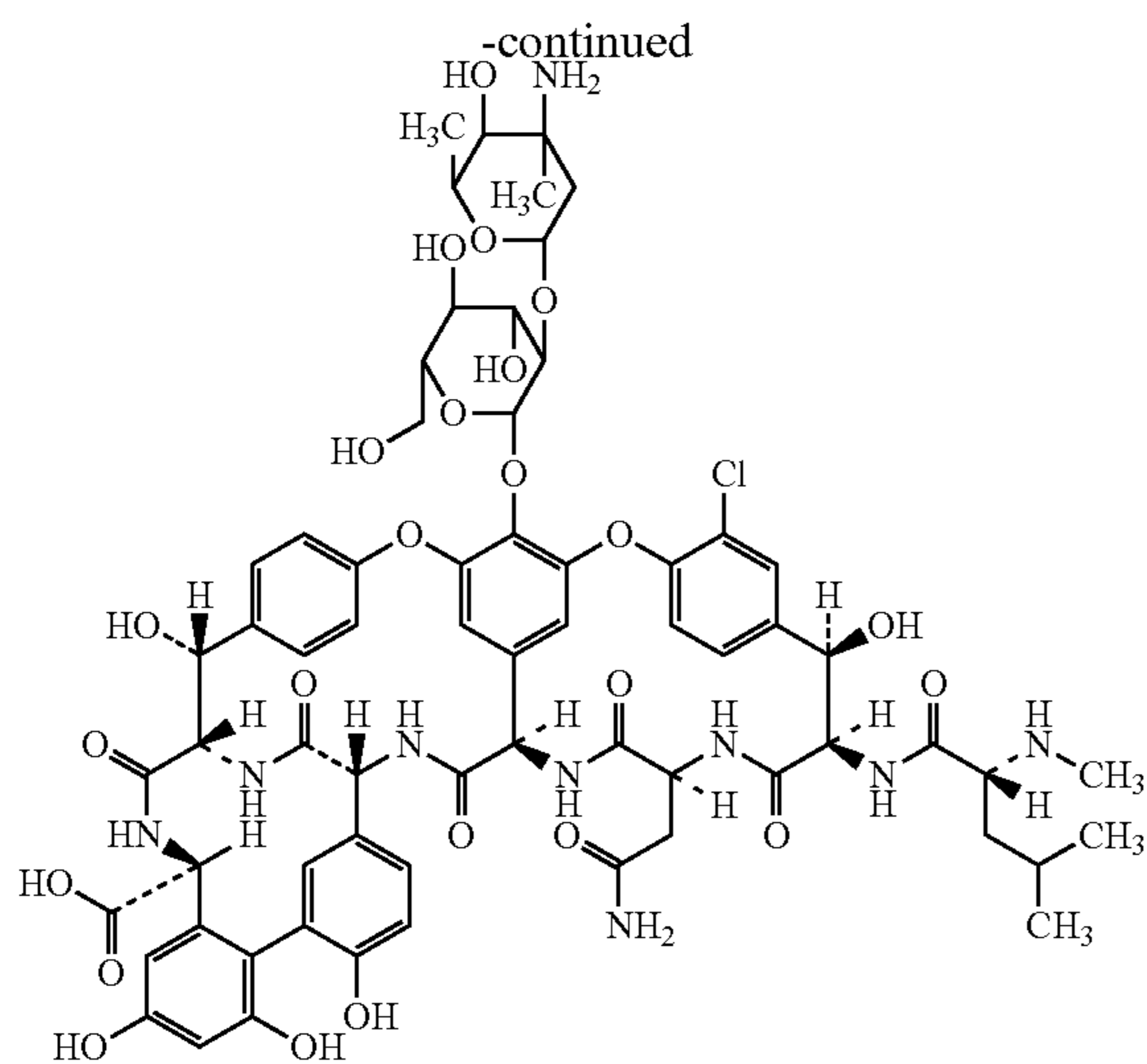
Monodechlorovancomycin
