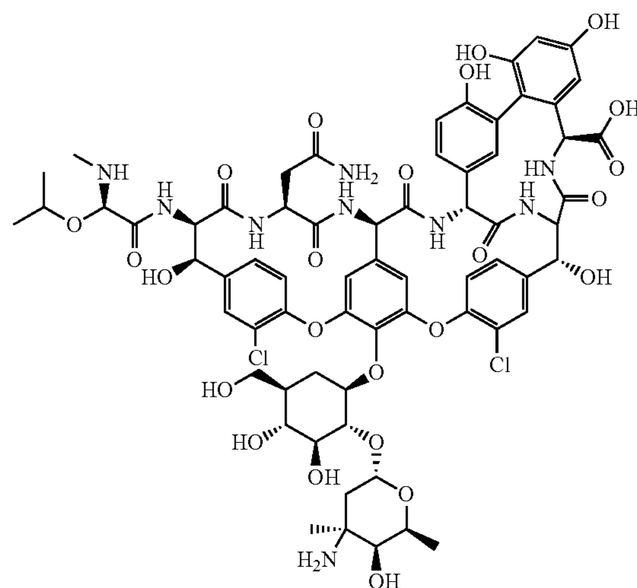
Vancomycin
