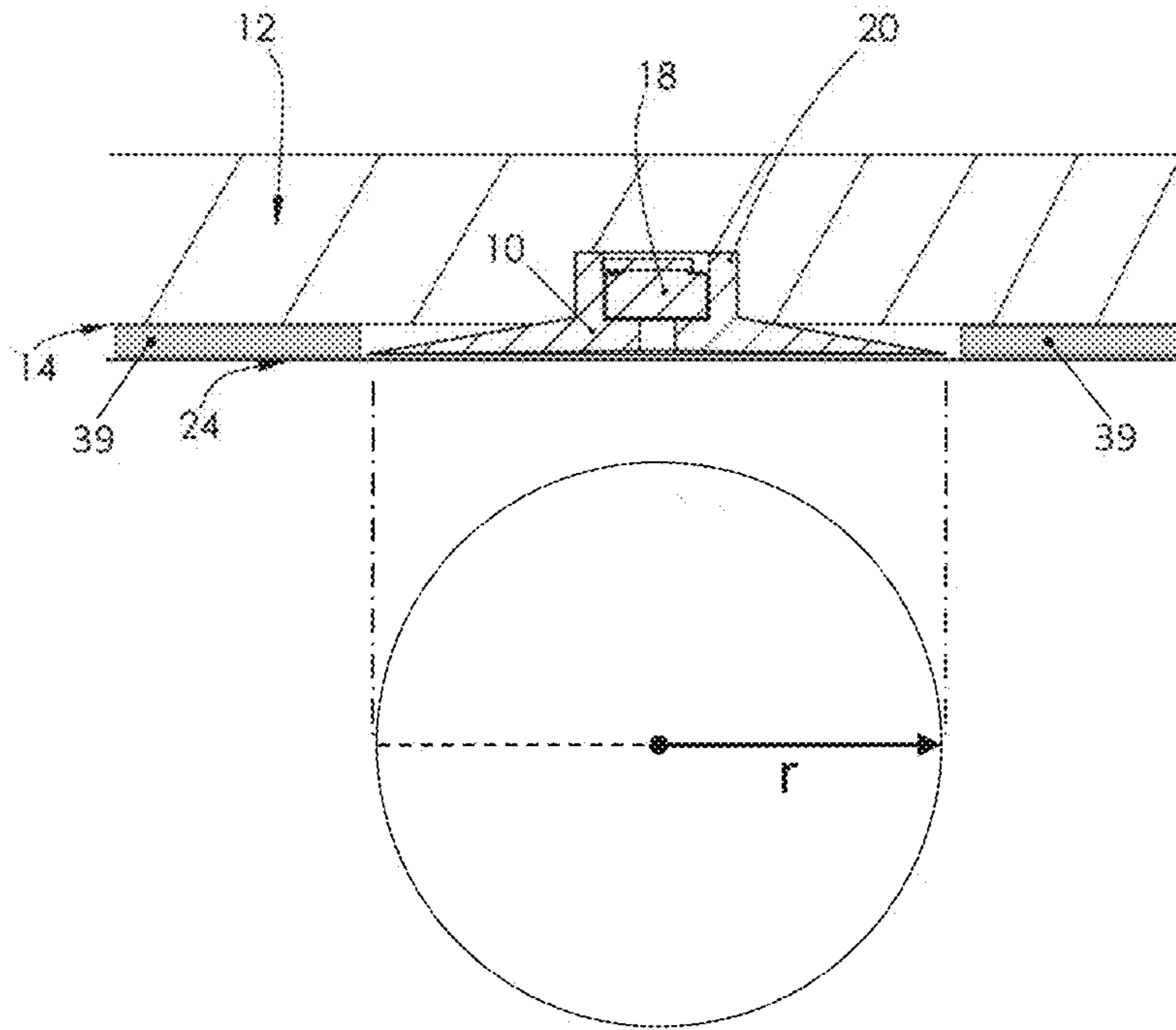
FIG. 8A
