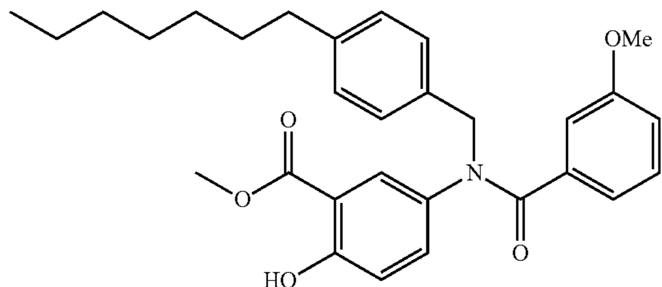
Methyl 5-(N-(4-heptylbenzyl)-3-methoxybenzamido)-2-hydroxybenzoate (19i)
