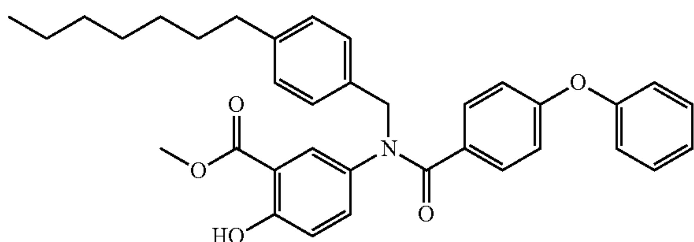
Methyl 5-(N-(4-heptylbenzyl)-4-phenoxybenzamido)-2-hydroxybenzoate (19f)
