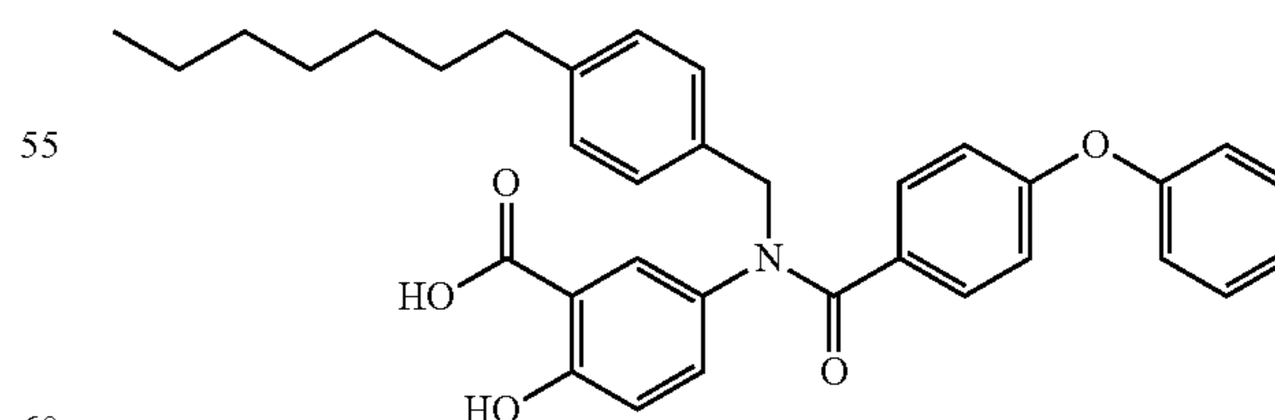
5-(N-(4-heptylbenzyl)-4-phenoxybenzamido)-2-hydroxybenzoic acid (20f)
