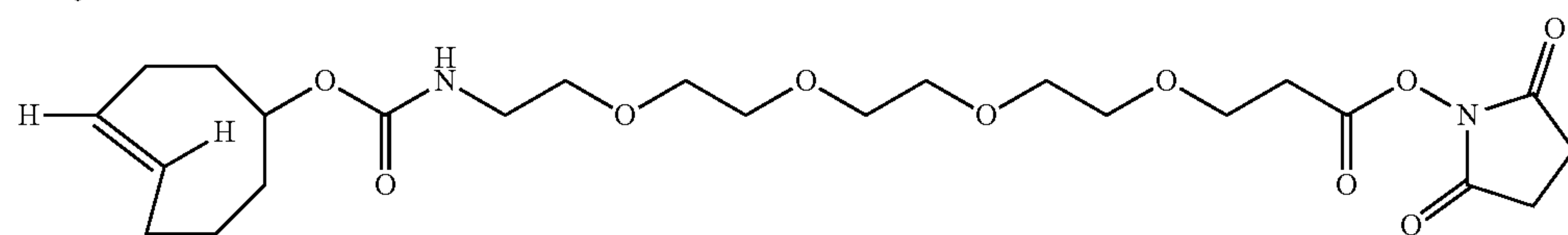
TCO-PEG4-NHS Ester 1
