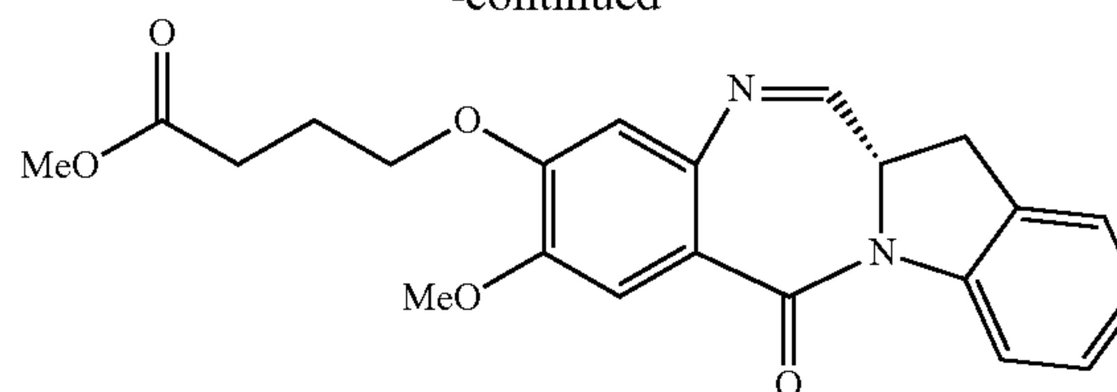
125
