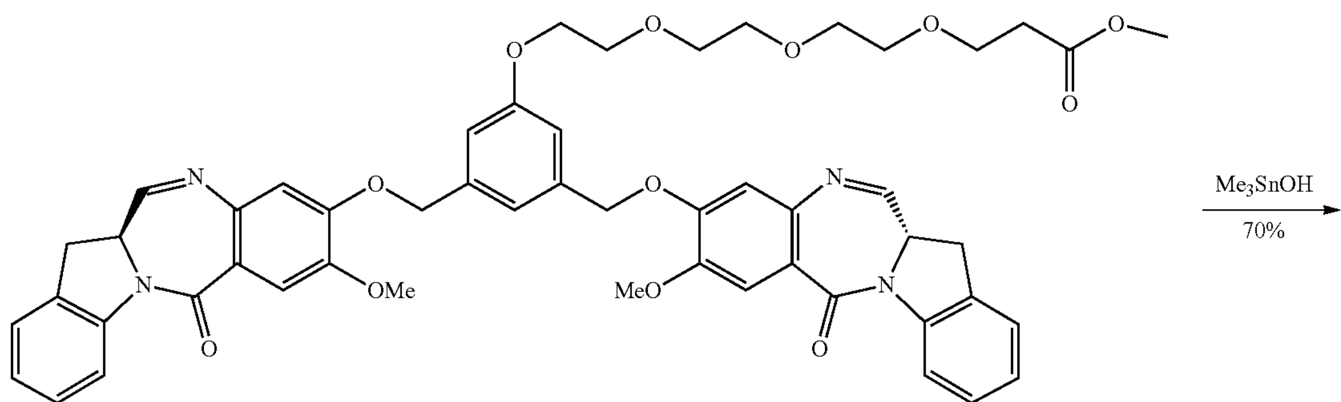
263c
