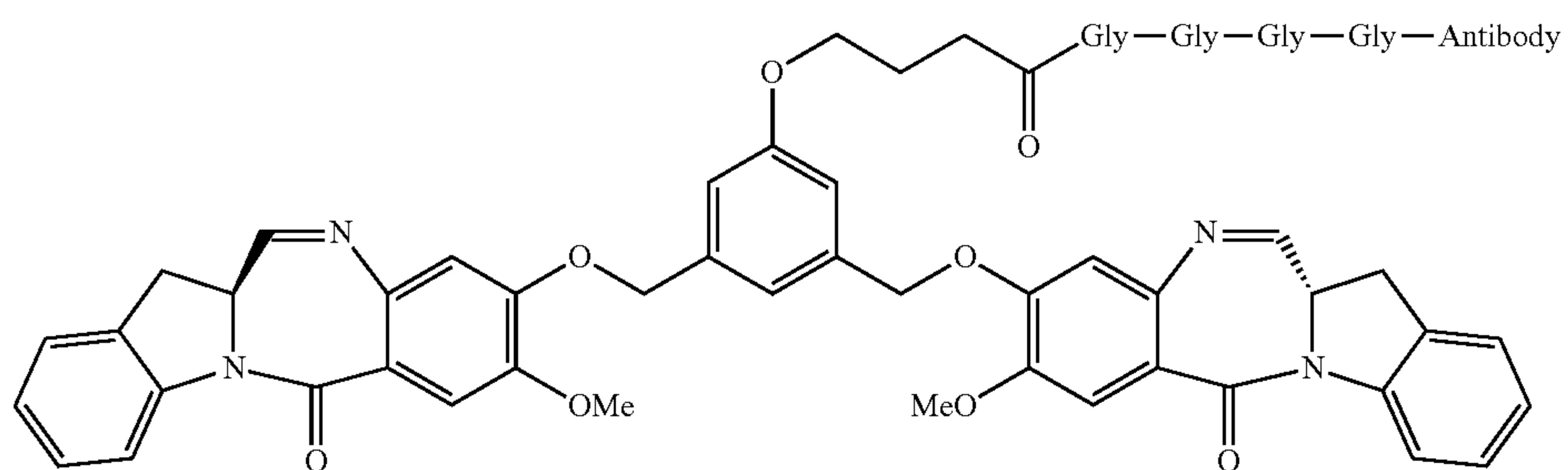
Dimer 1
