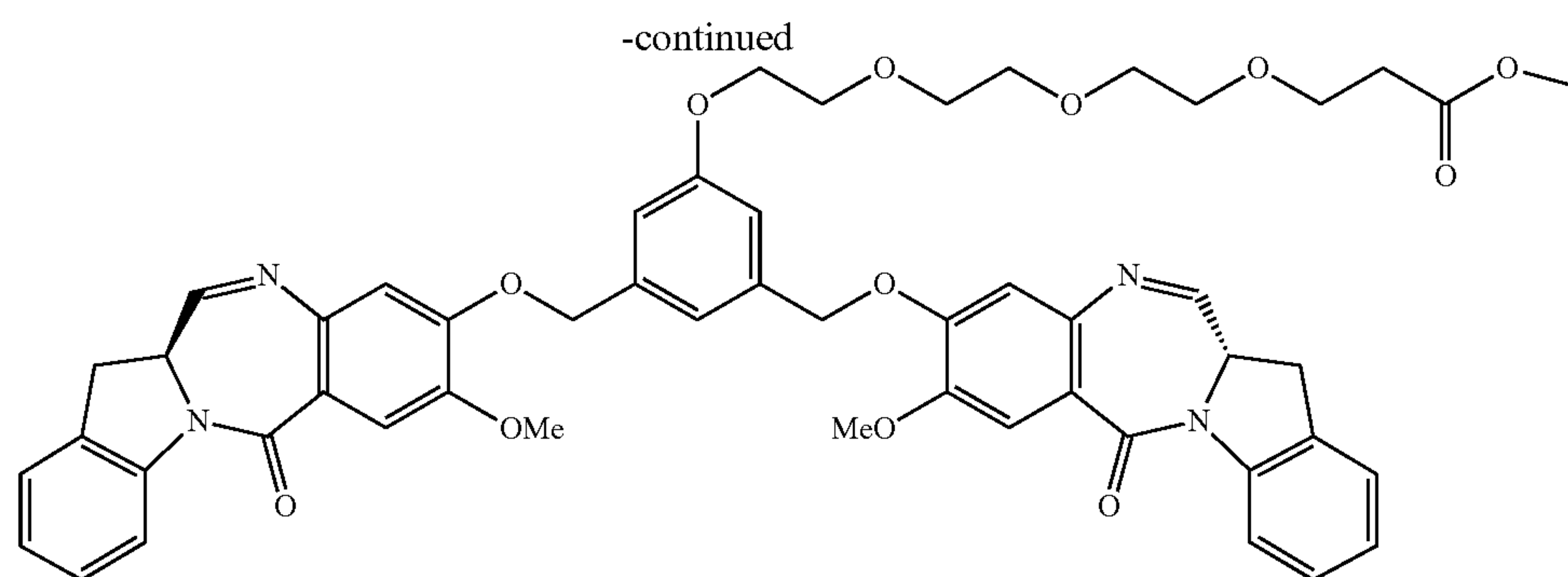
263c
