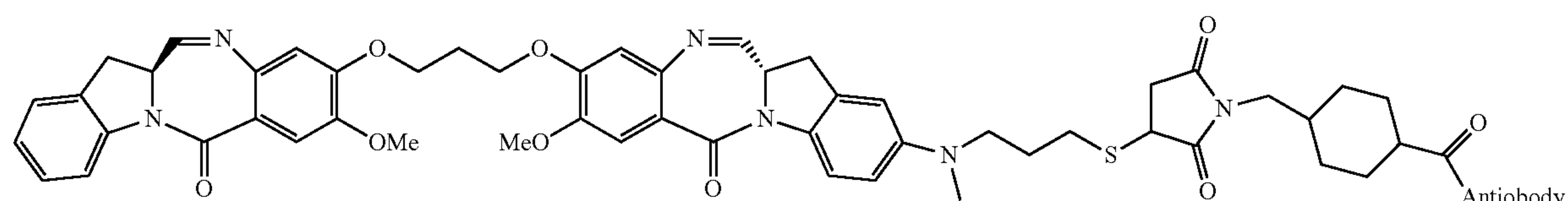
Dimer 8
