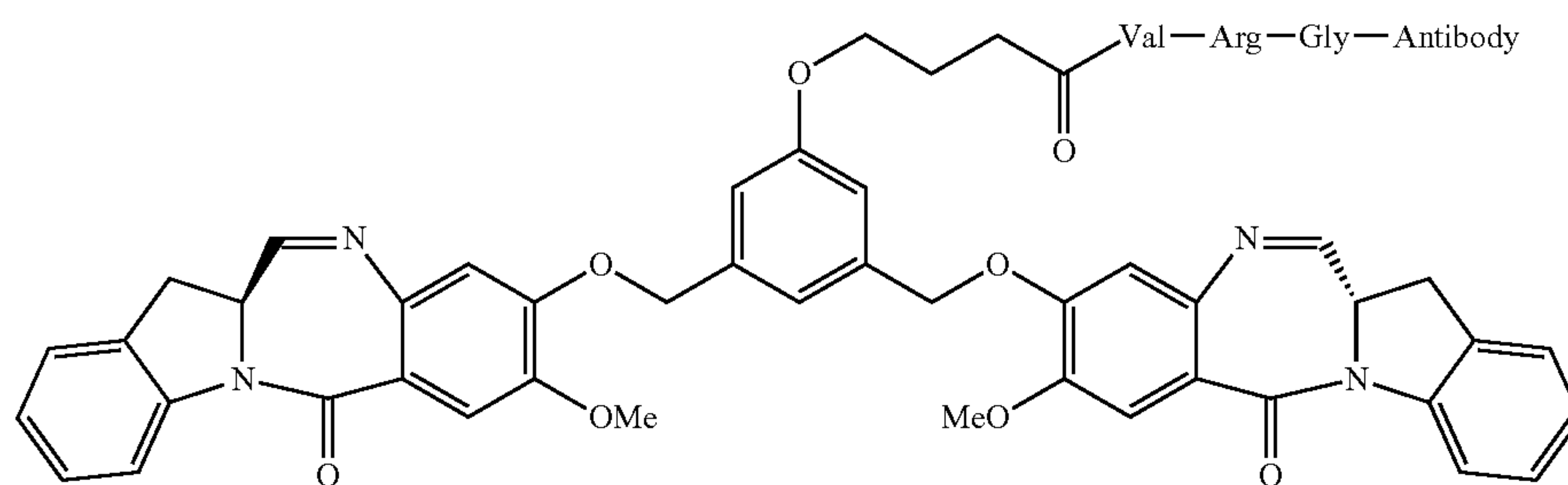
Dimer 2
