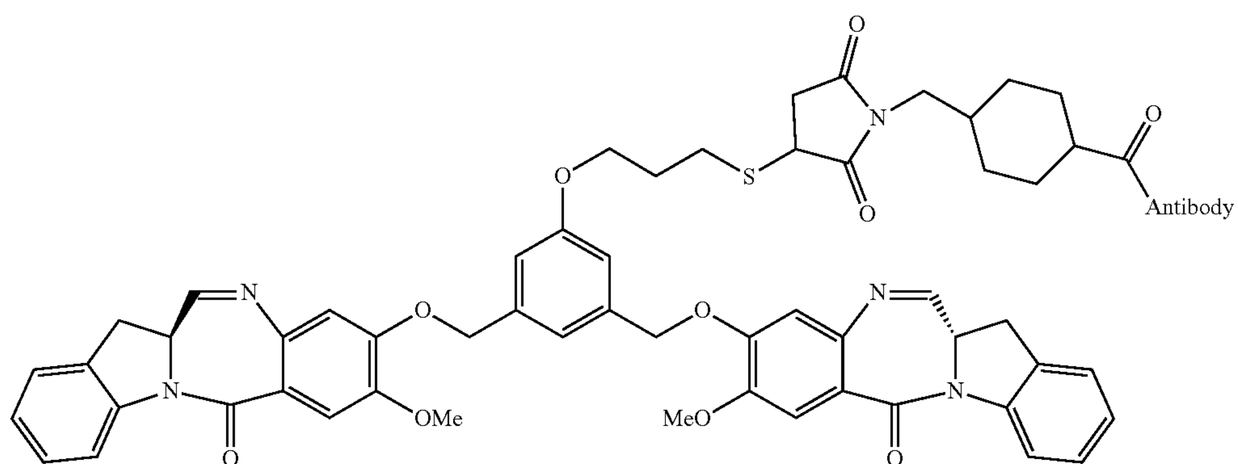
Dimer 3
