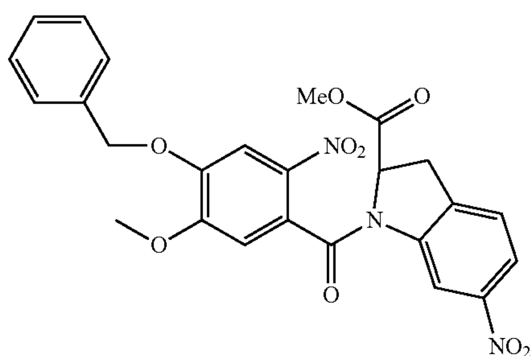
258b
