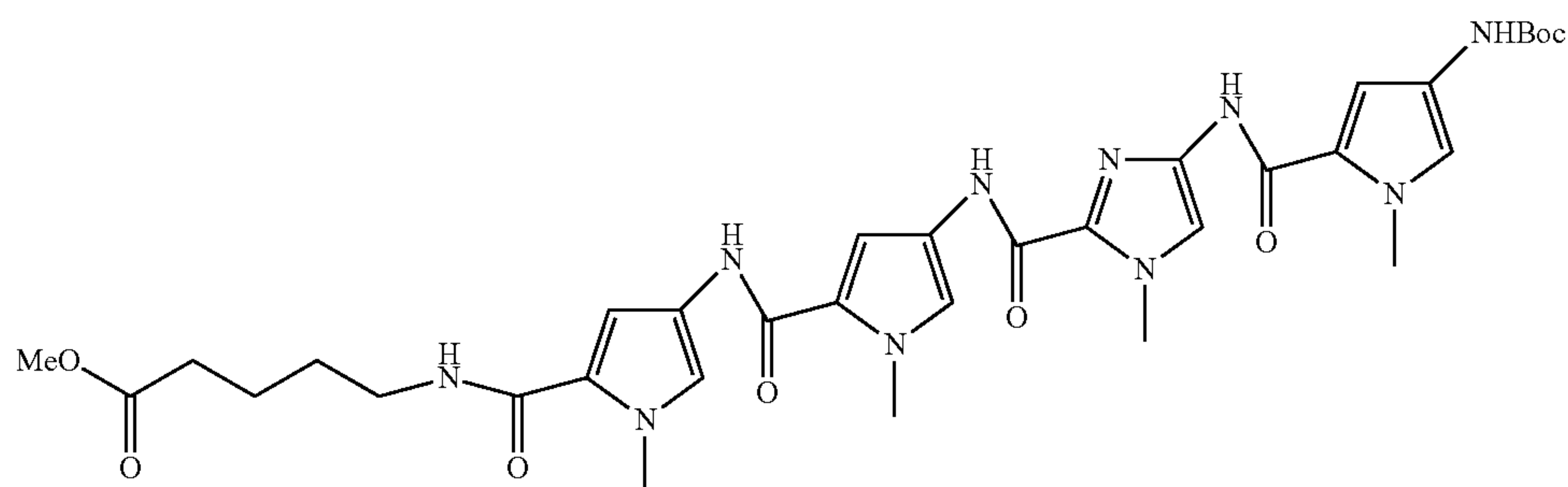
124
