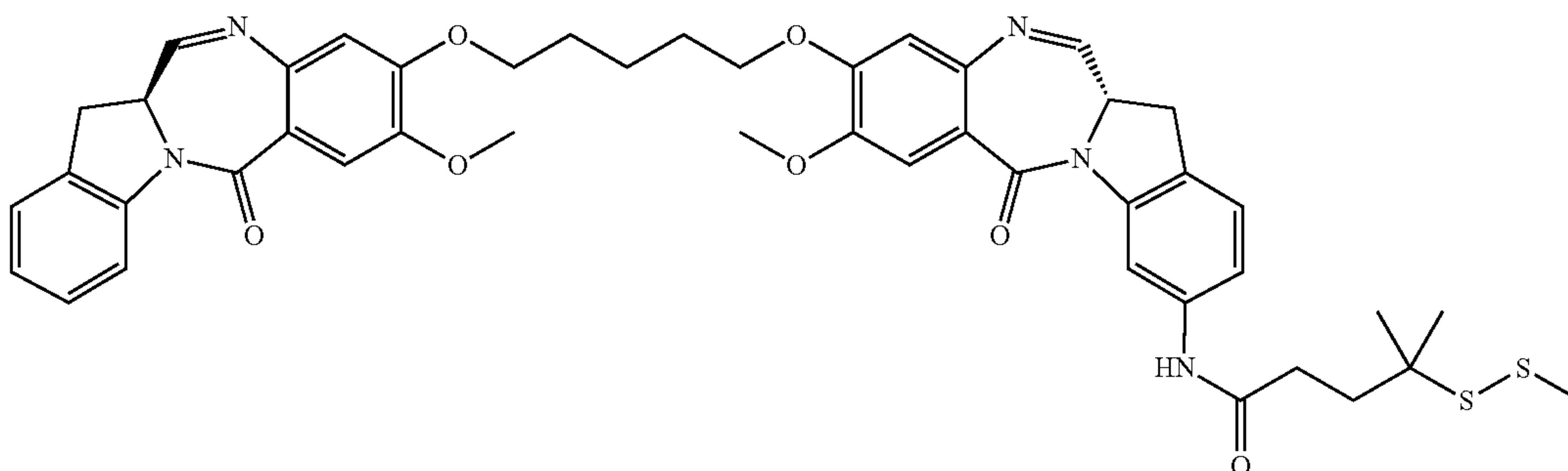
259b
