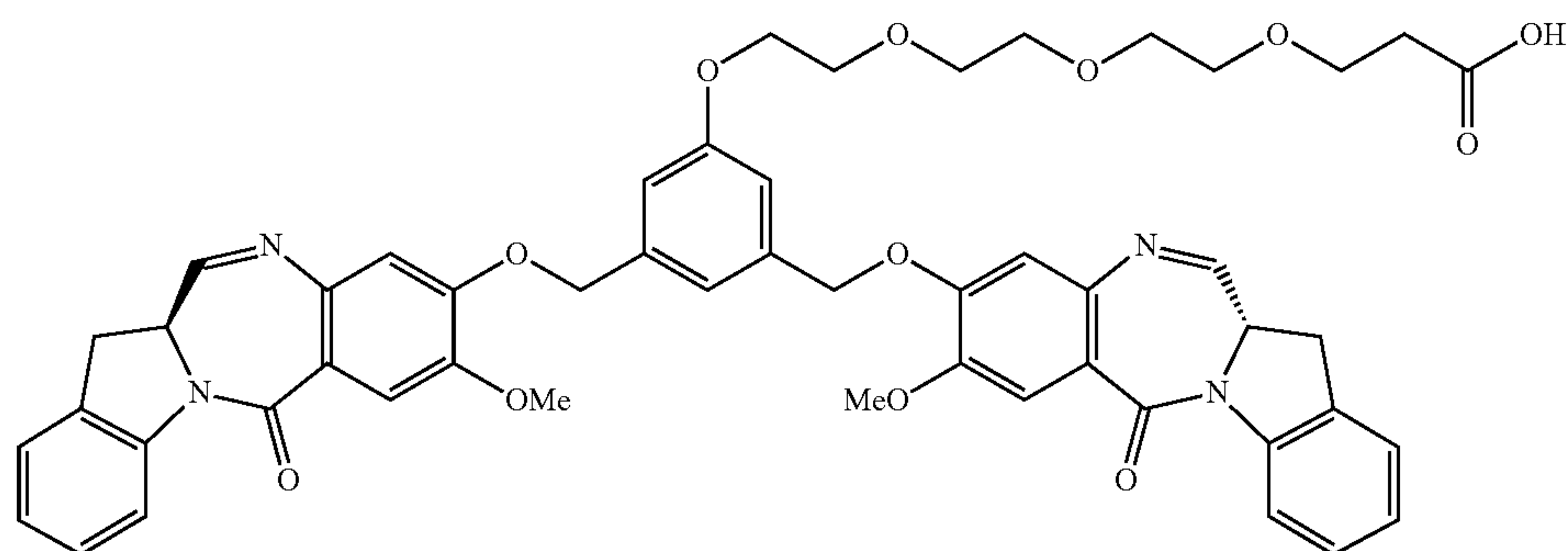
263d
