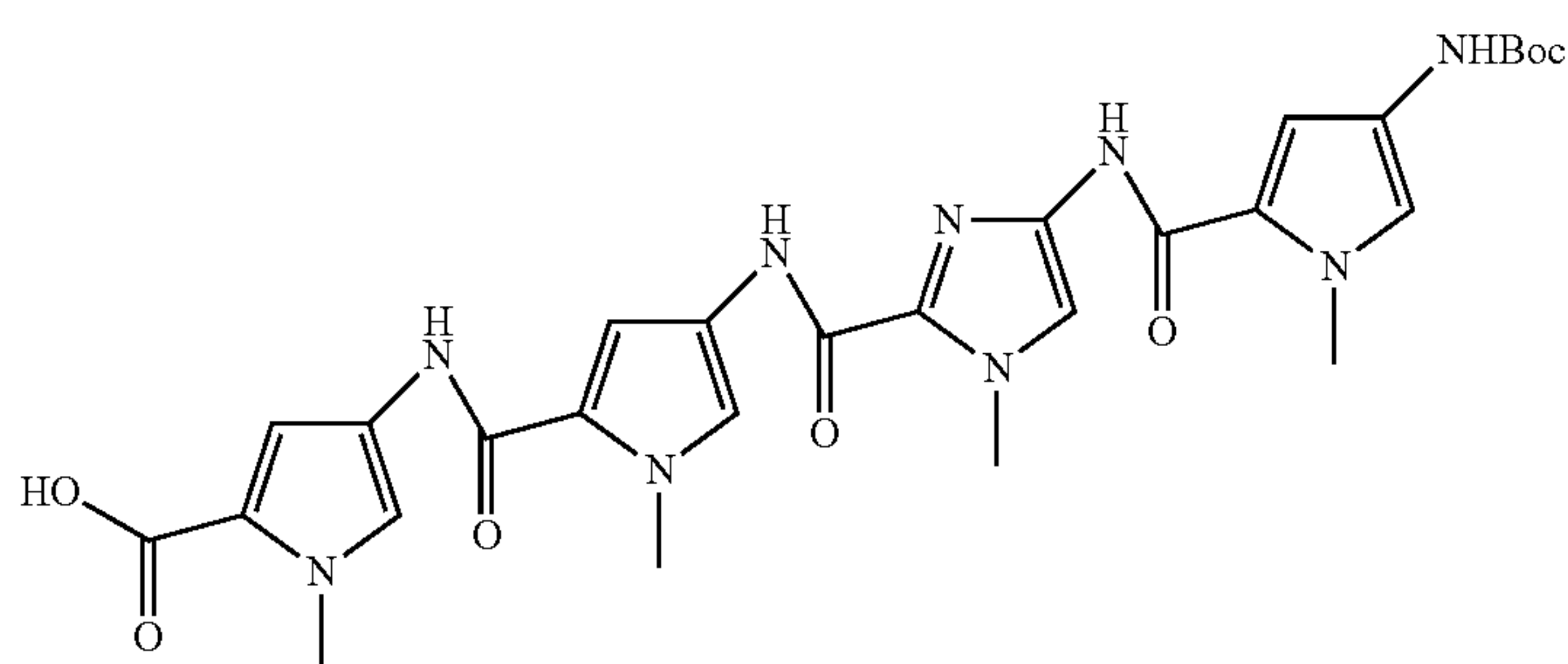
123
