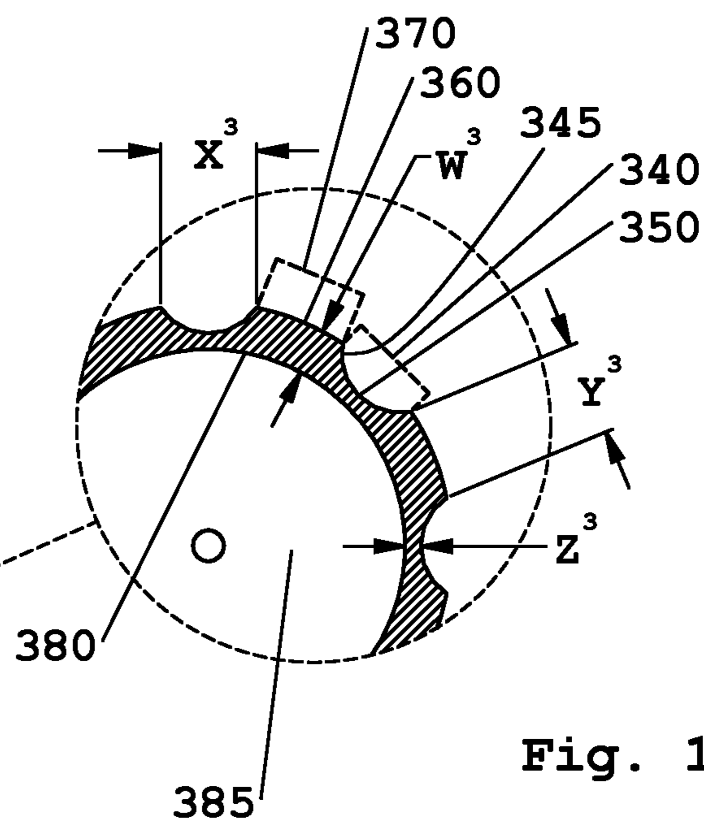
SECTION A3-A3
