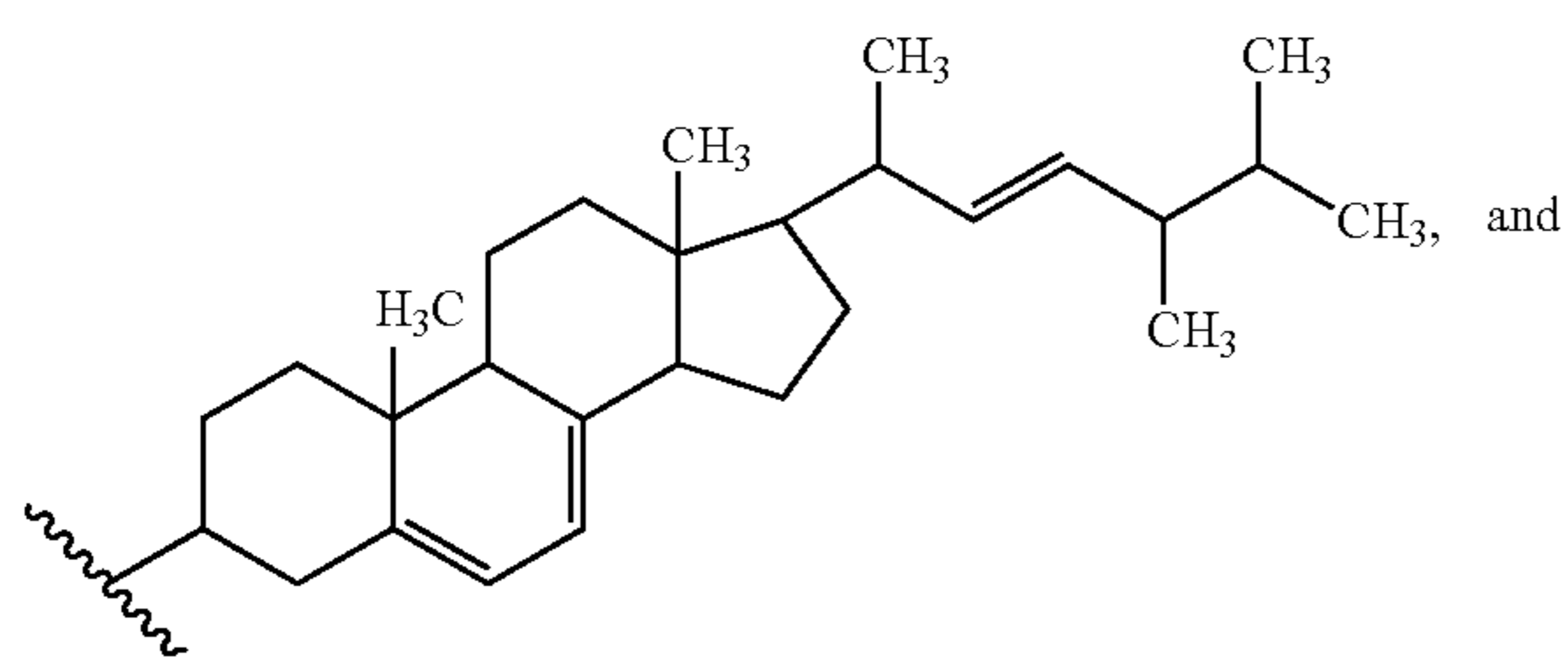
(ergosterol)
