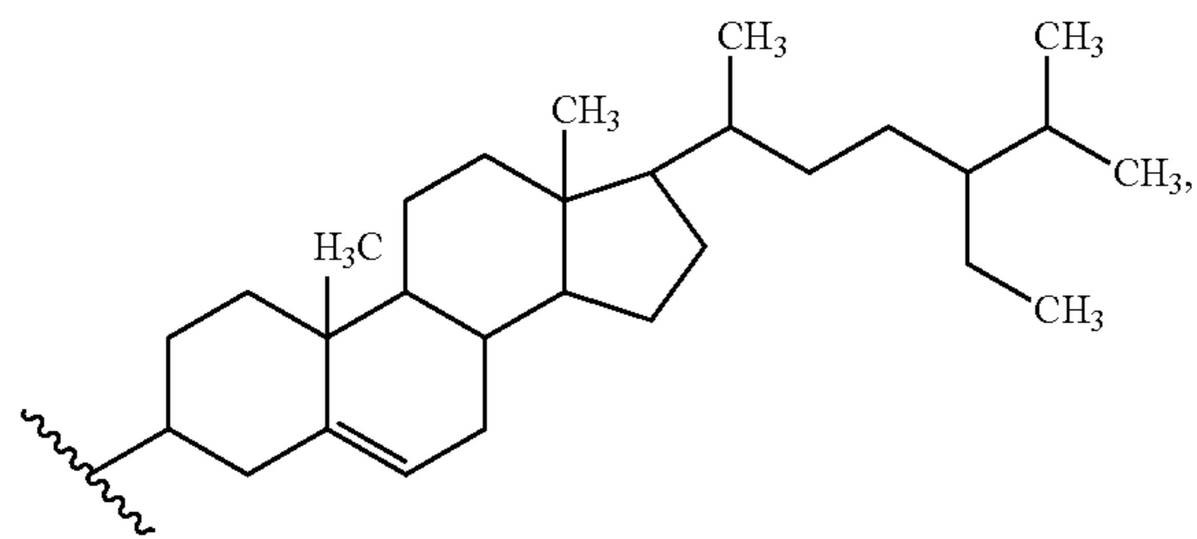
(sitosterol)
