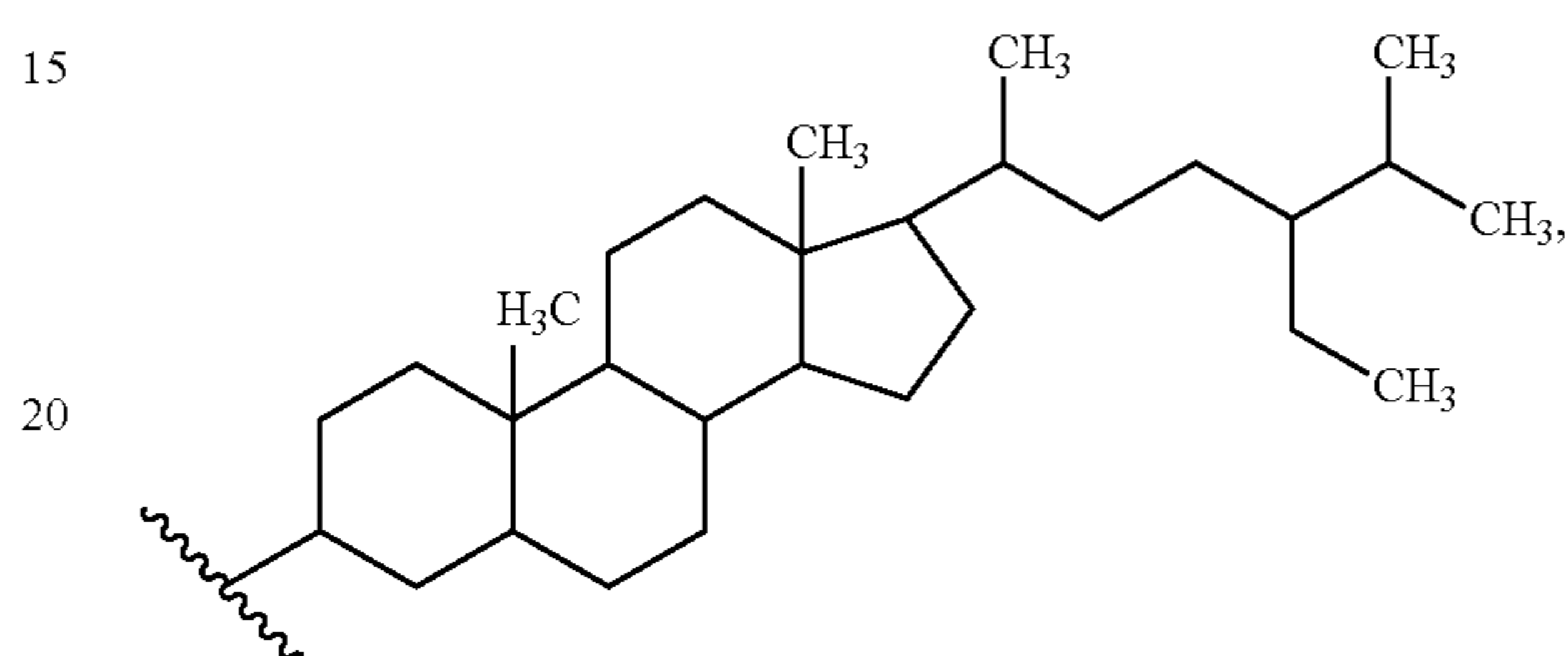
(stigmastanol)
