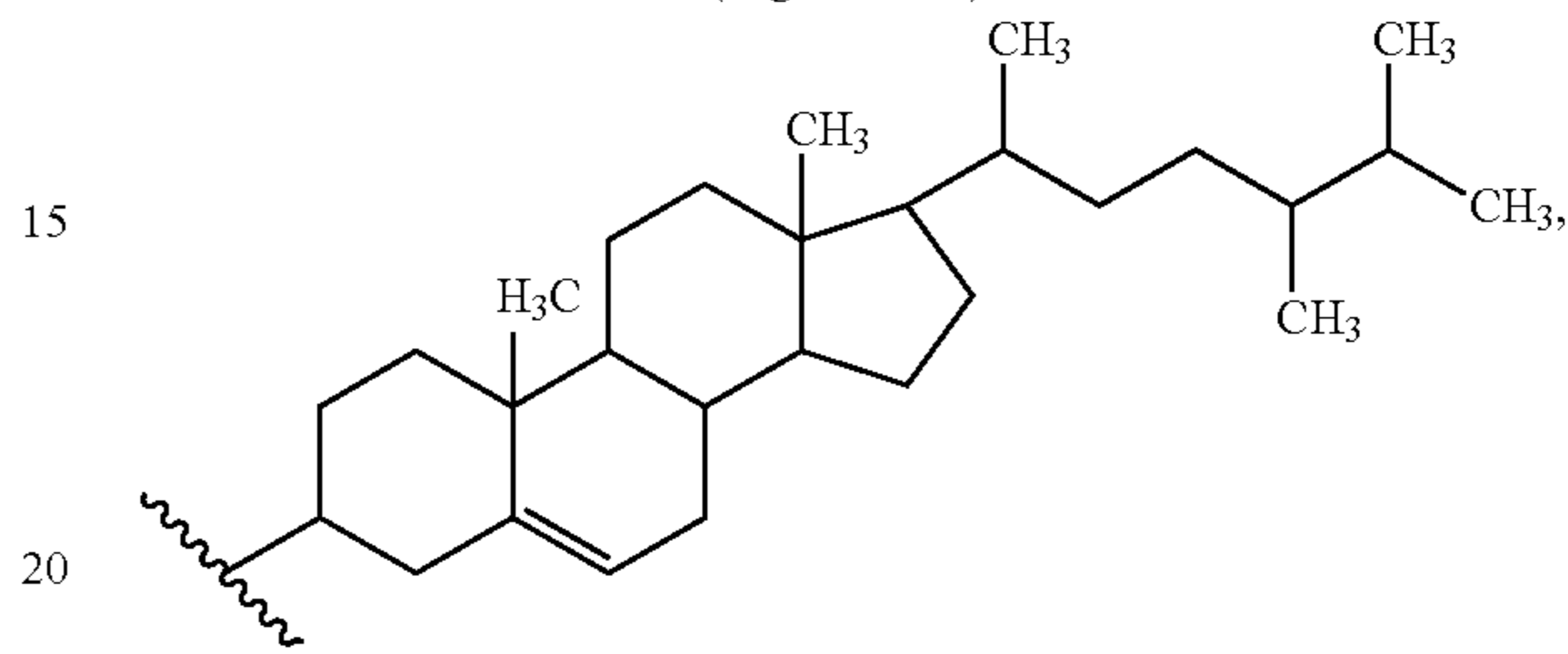
(campesterol)
