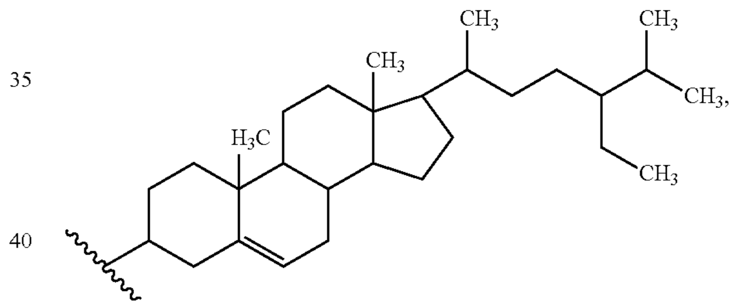
(sitosterol)
