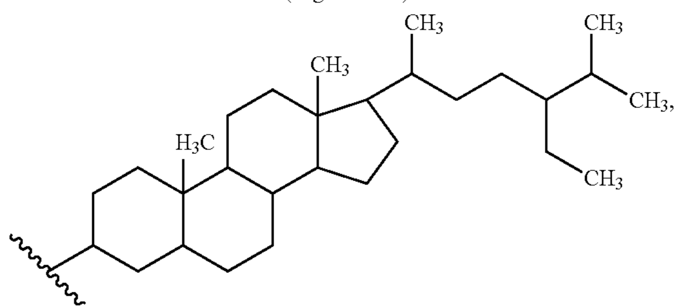
(stigmastanol)
