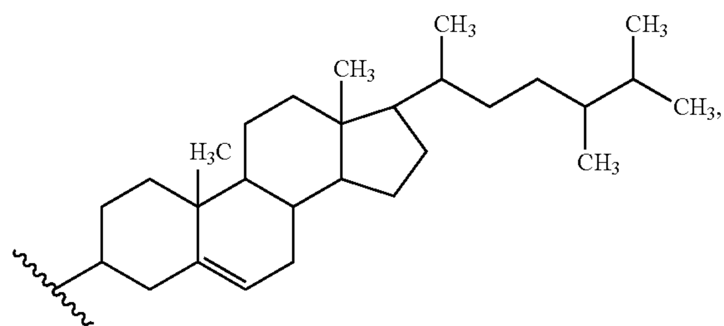
(campesterol)
