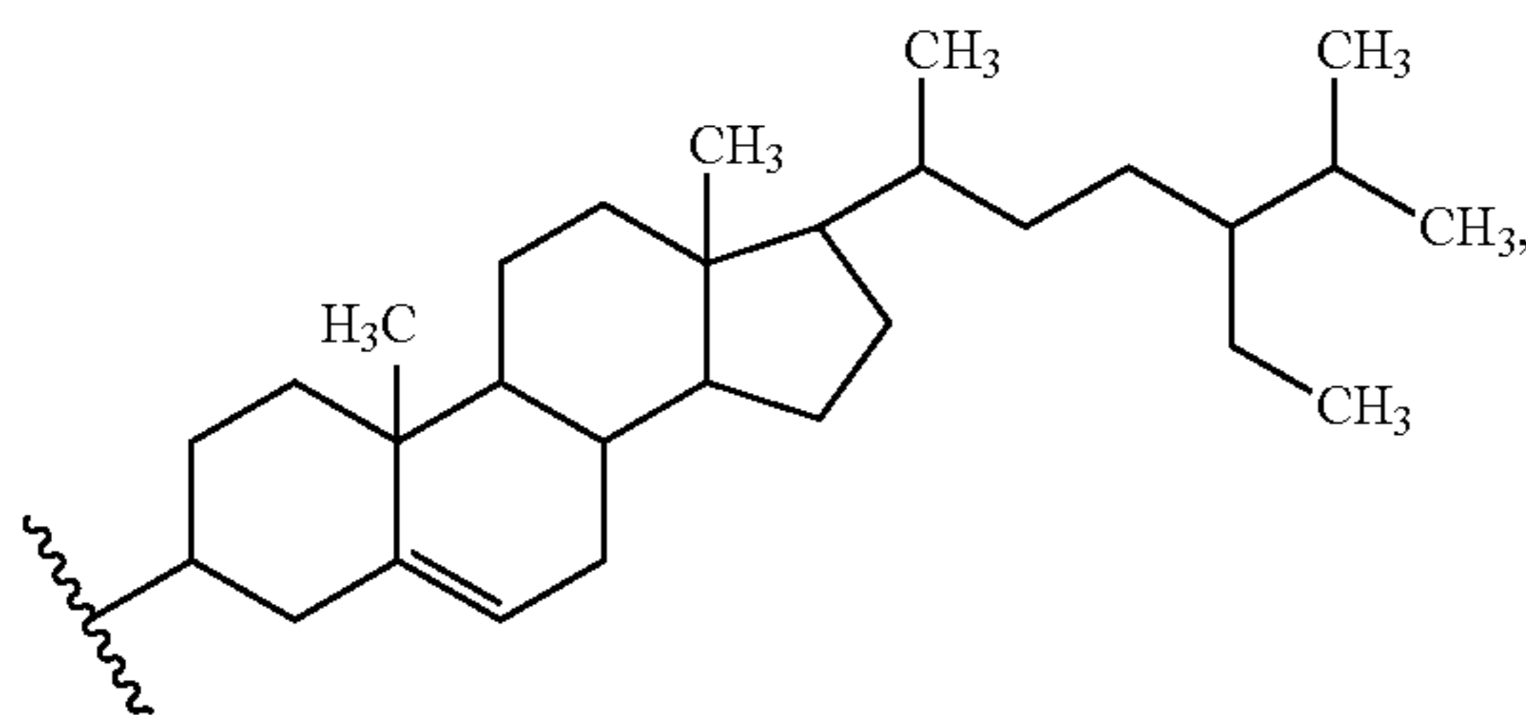
(sitosterol)
