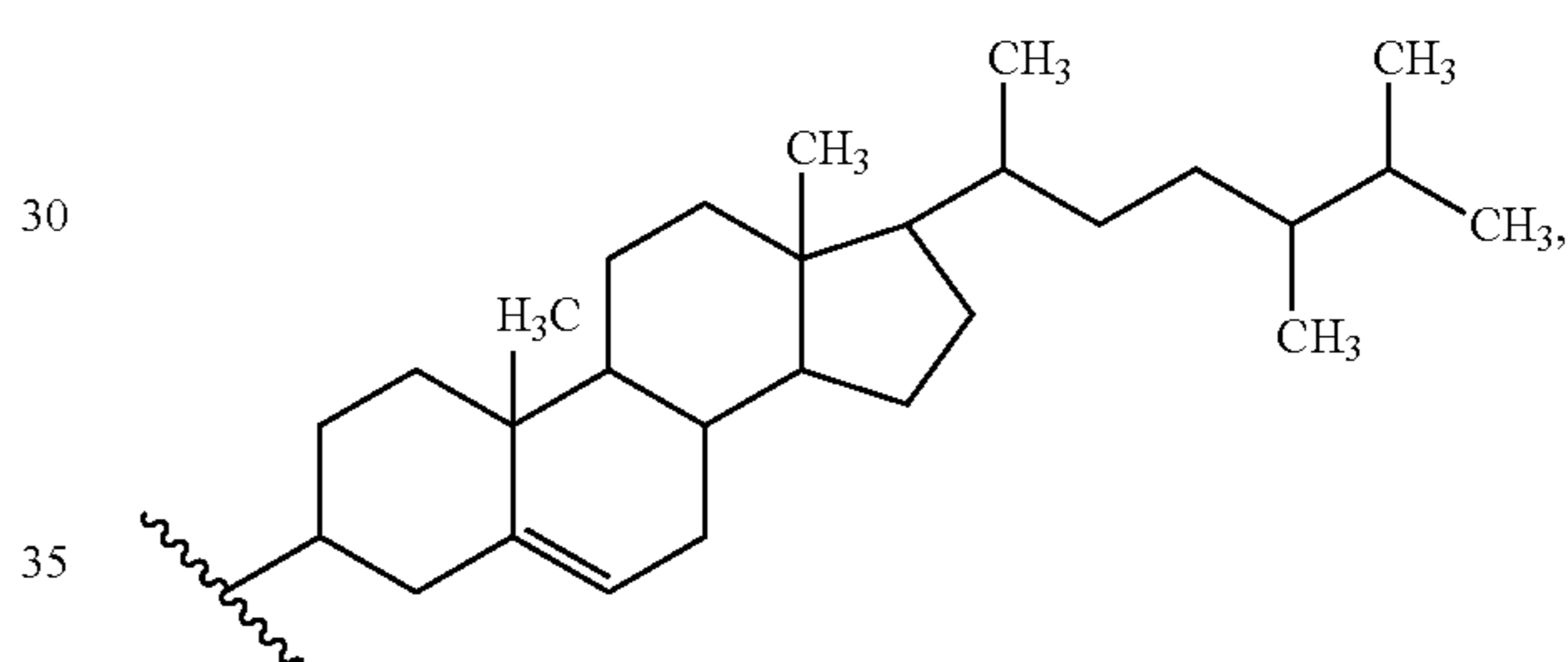
(campesterol)
