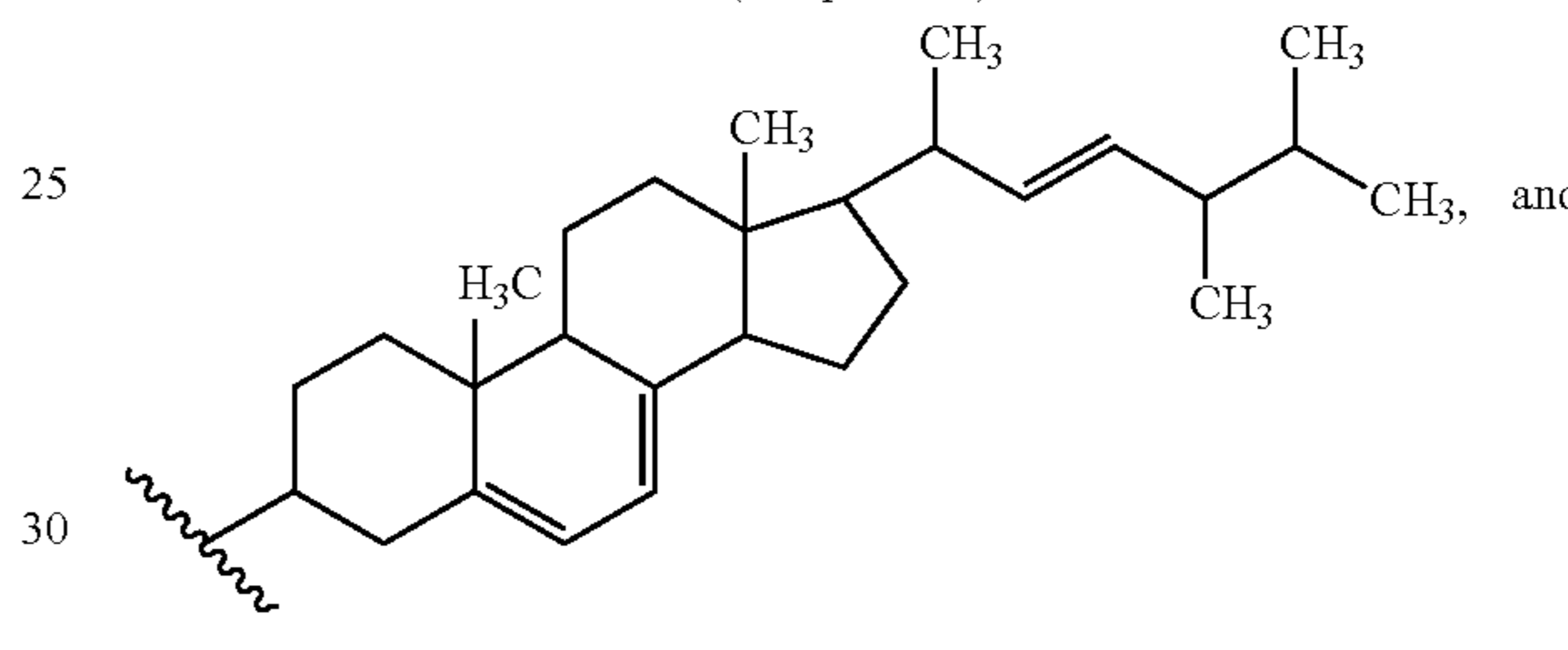
(ergosterol)
