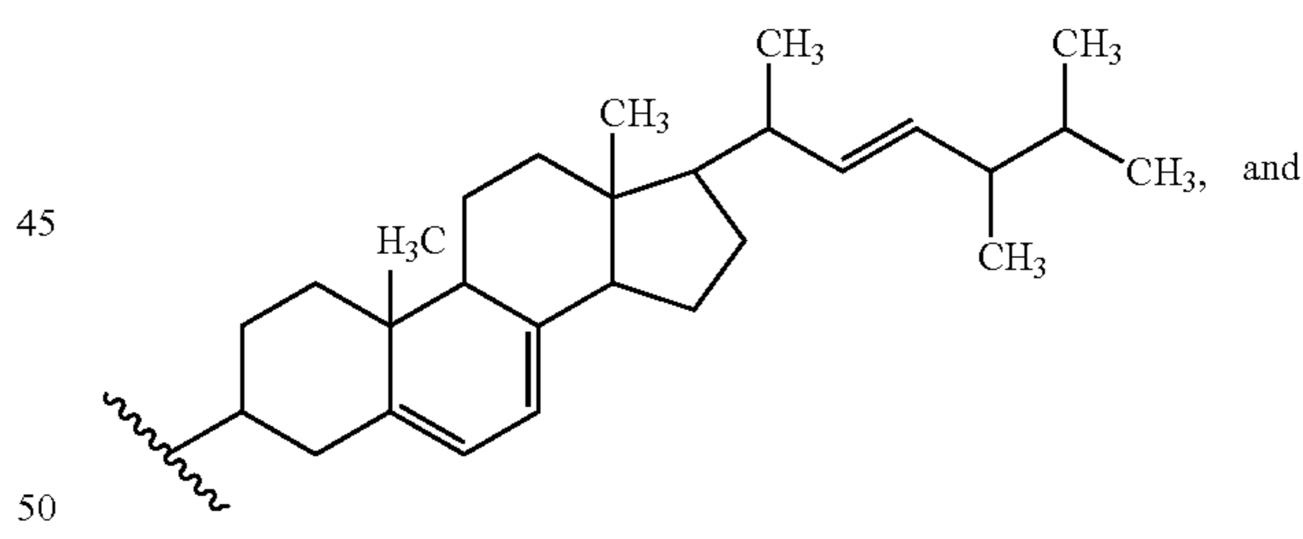
(ergosterol)
