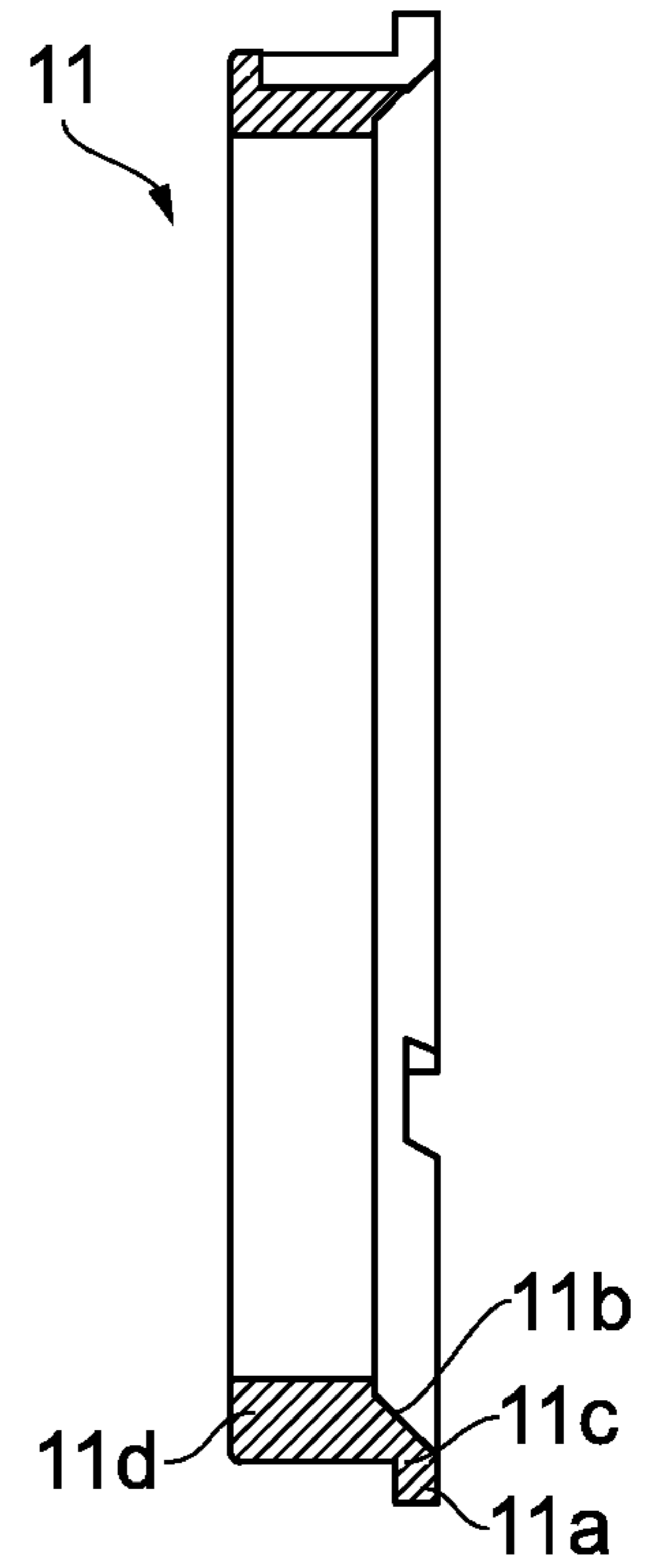
Section A-A FIG. 6B
