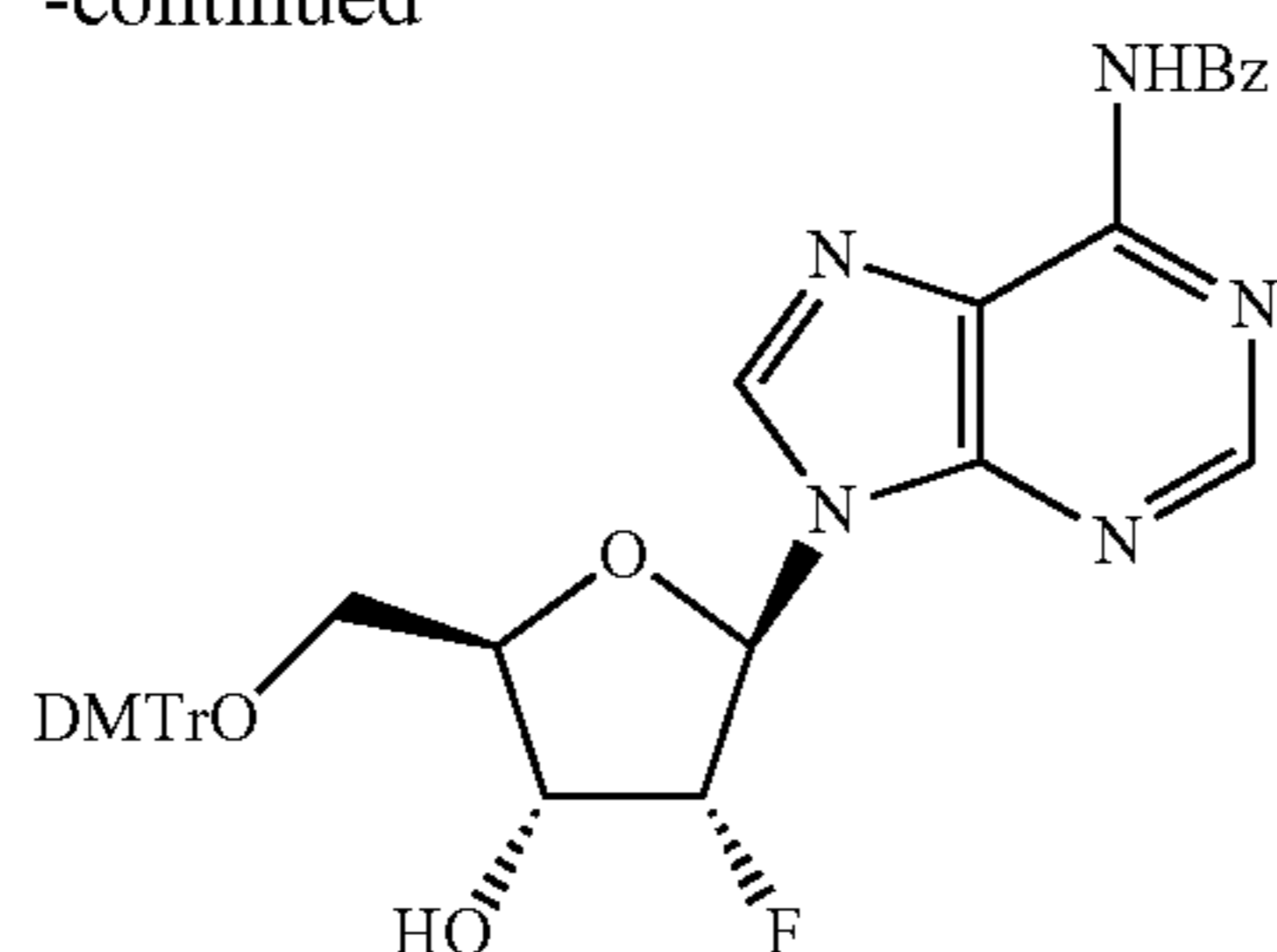
N-(9-((2R,3R,4R,5R)-5-((bis(4-methoxyphenyl)(phenyl)methoxy)methyl)-3-fluoro-4-hydroxytetrahydrofuran-2-yl)-9H-purin-6-yl)benzamide
