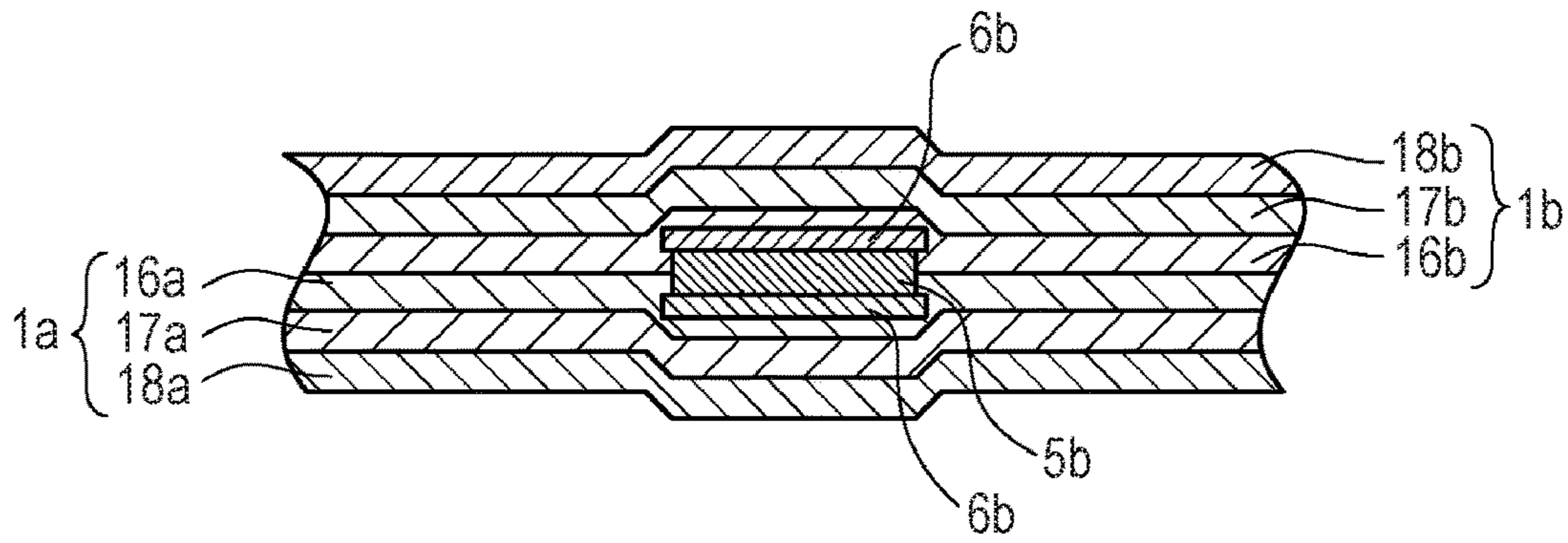
FIG. 10B
