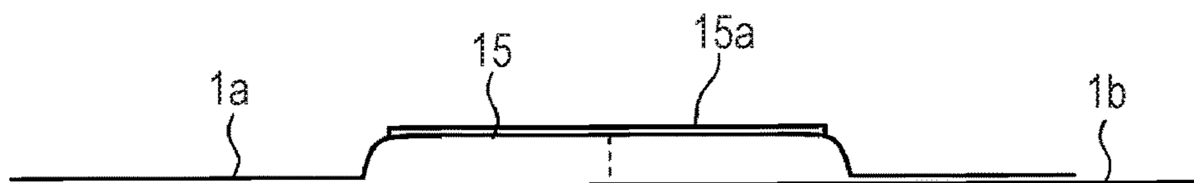
FIG. 7C
