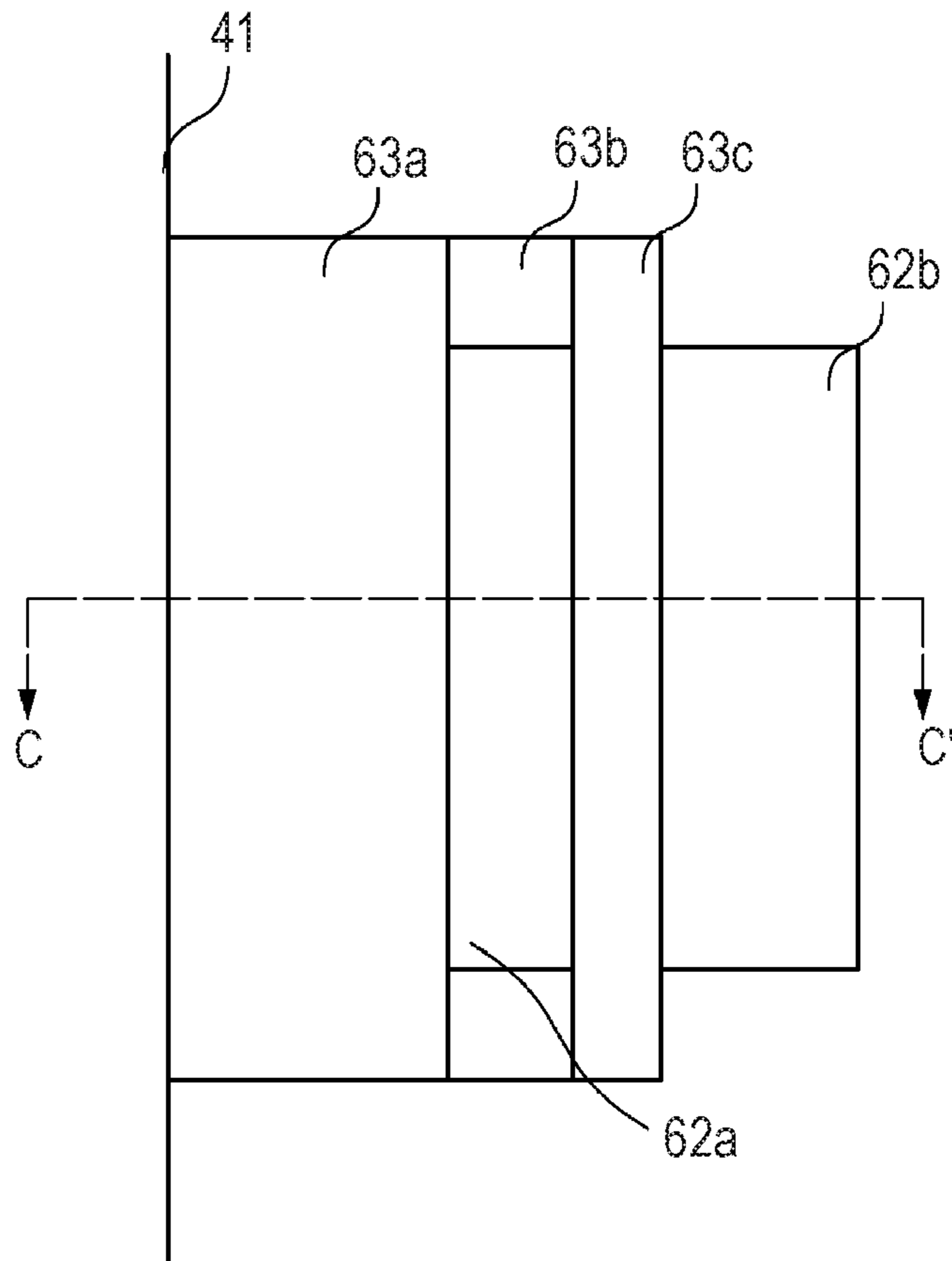
FIG. 20B
