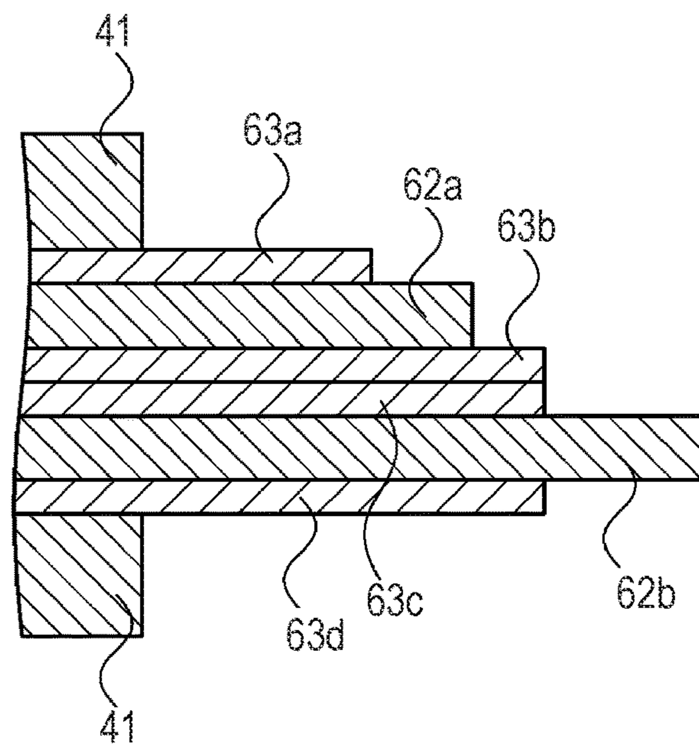
FIG.21B
