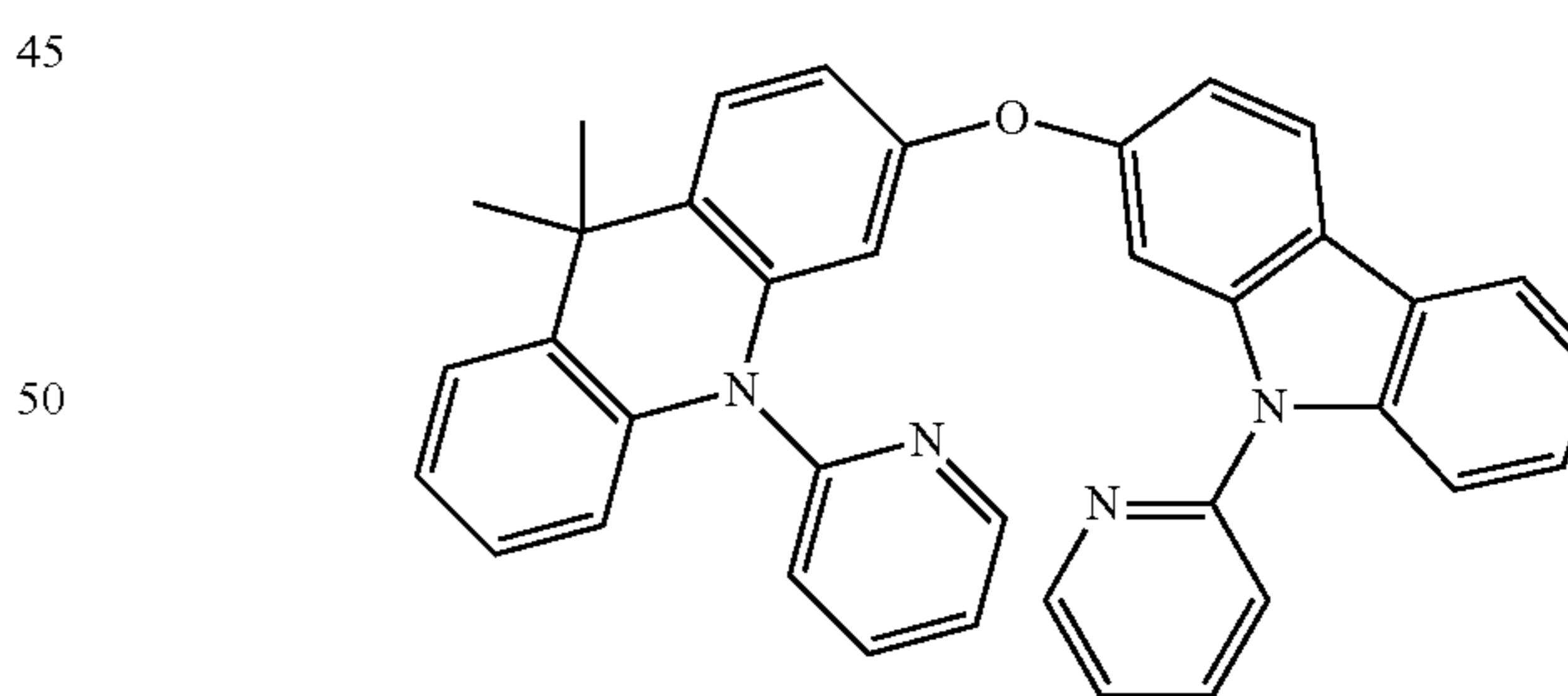
NON' Ligand
