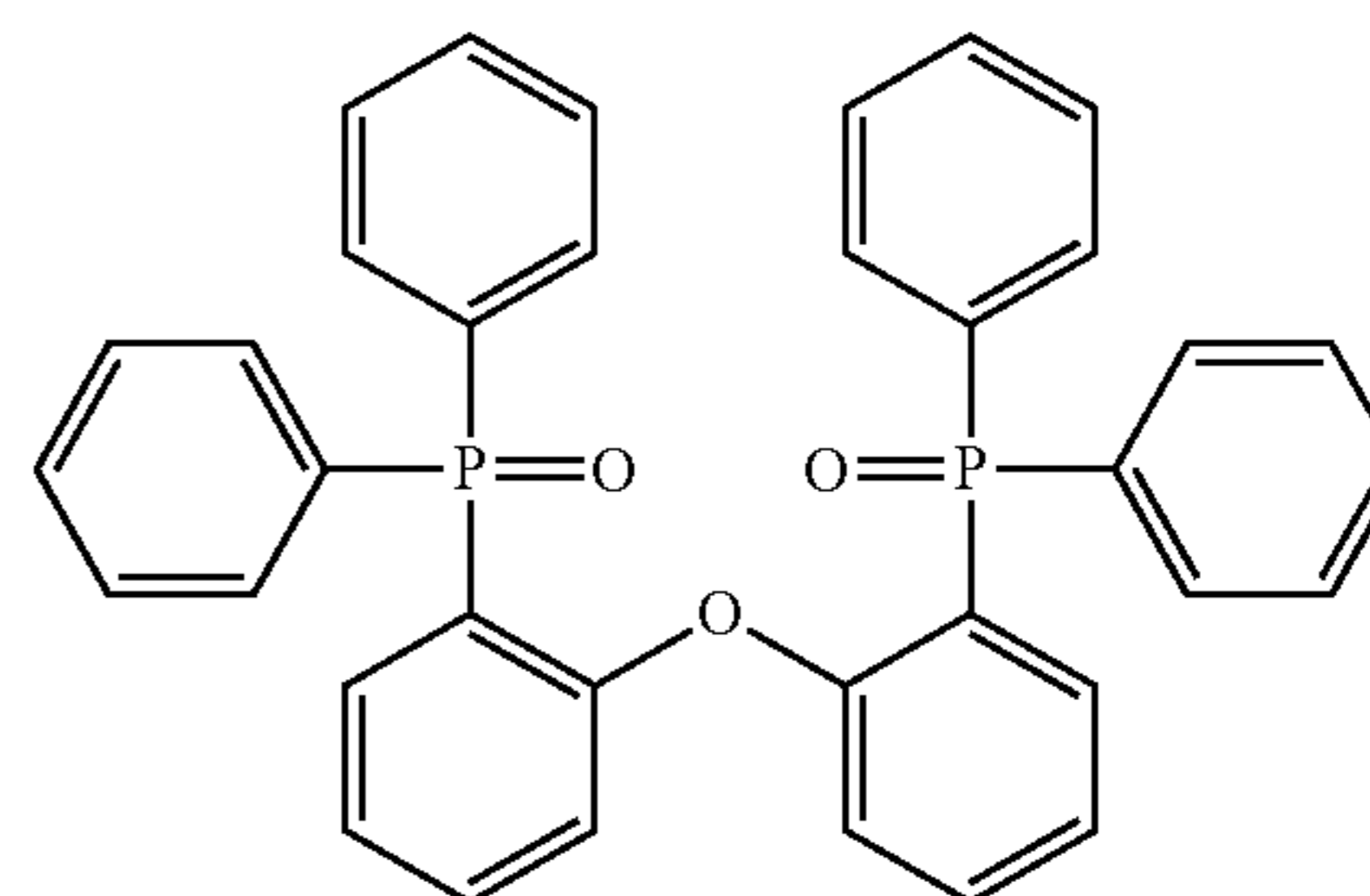
DPEPO
