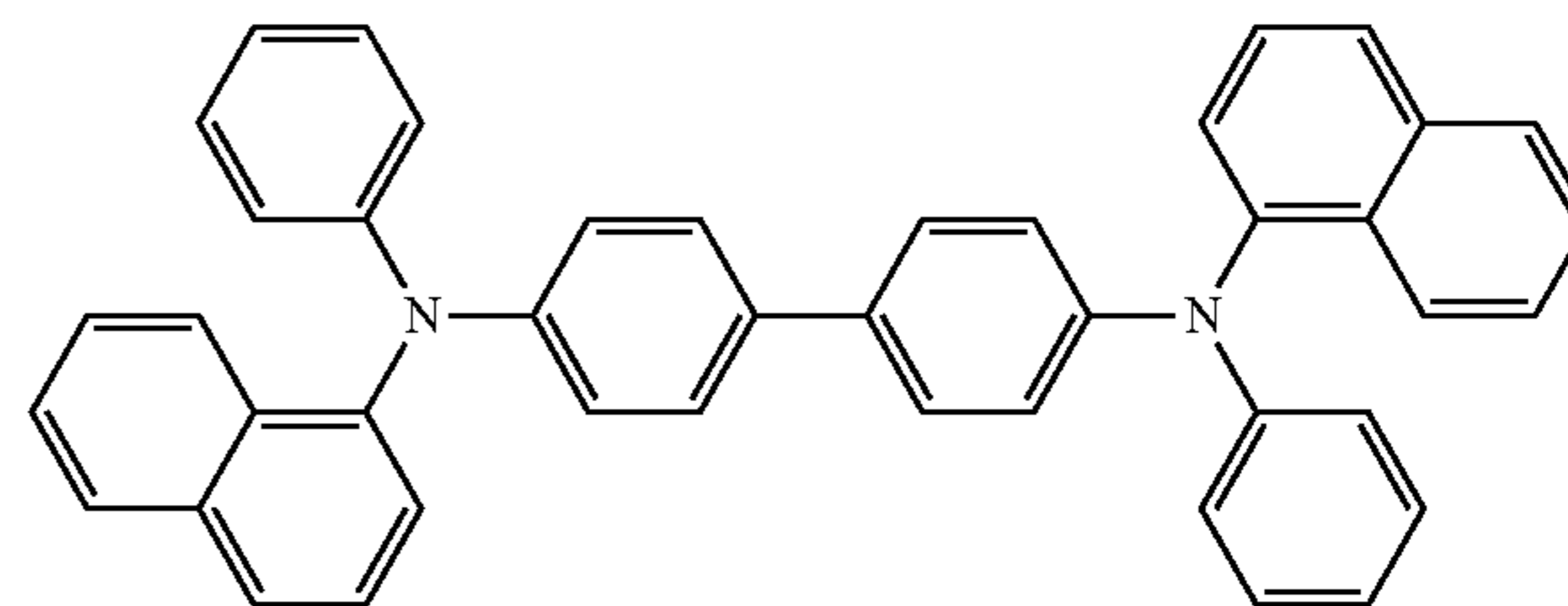
\alpha -NOA
