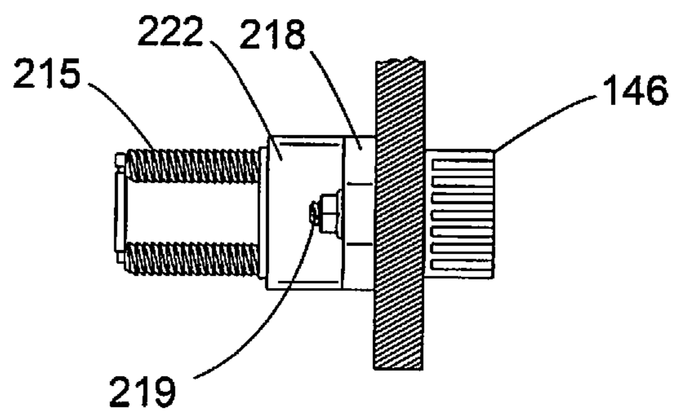
FIG. 39C
