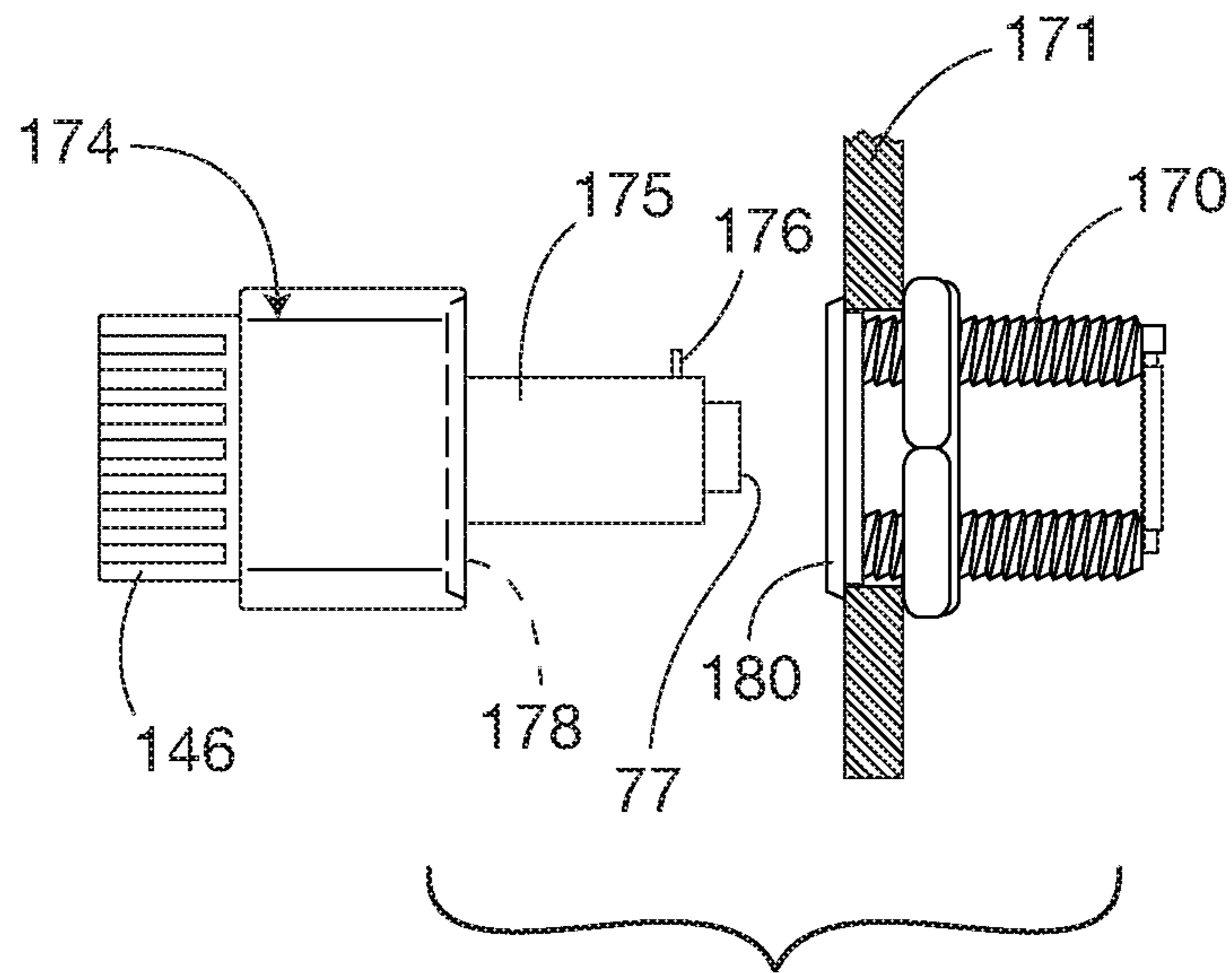
FIG. 34A
