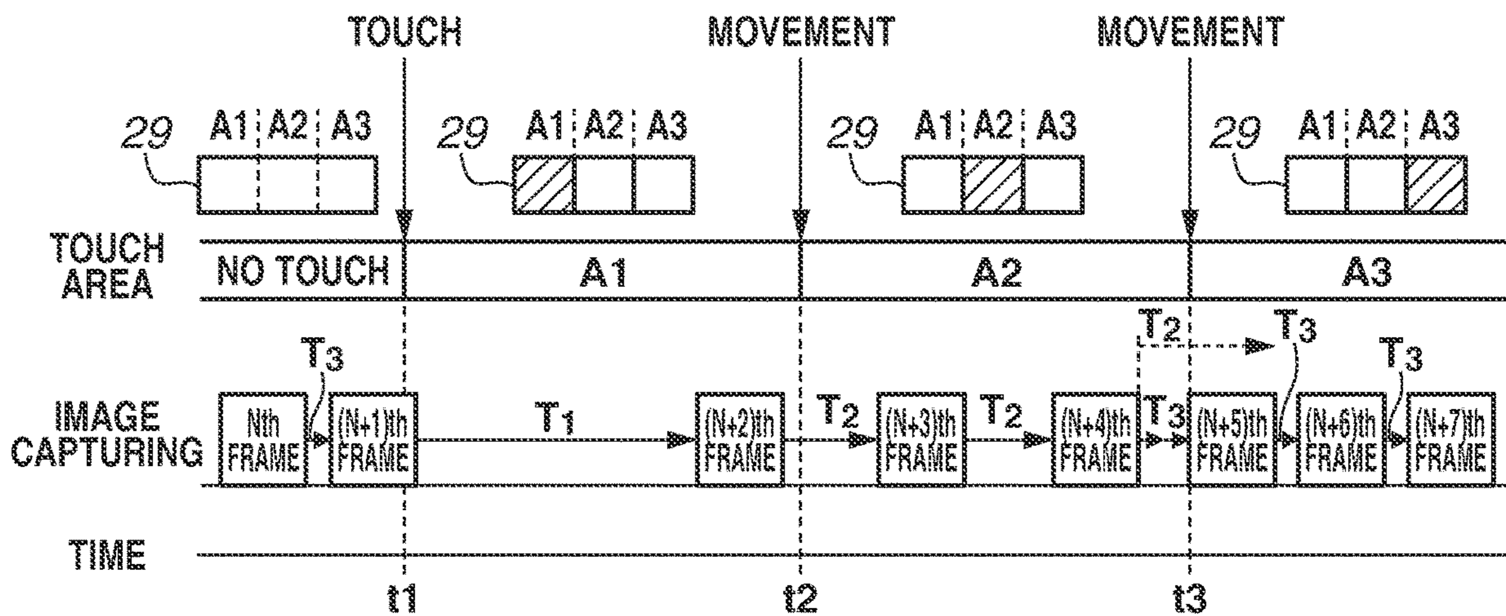
FIG.5B
