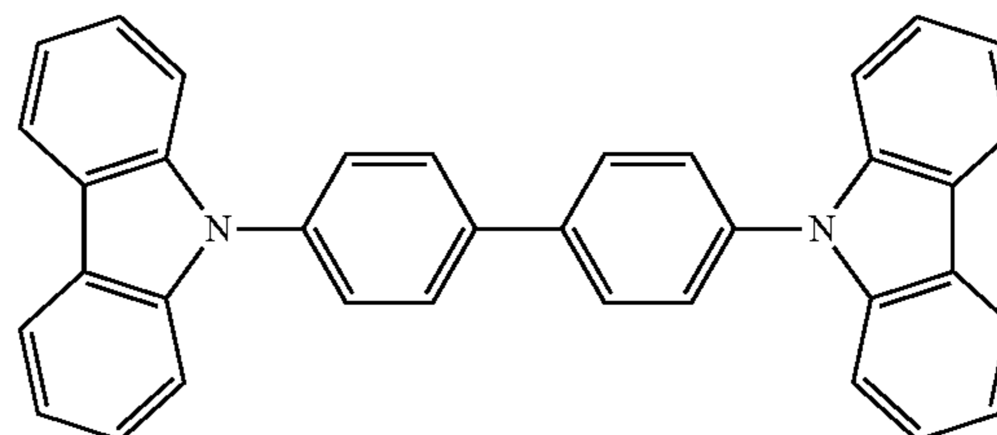
CBP
