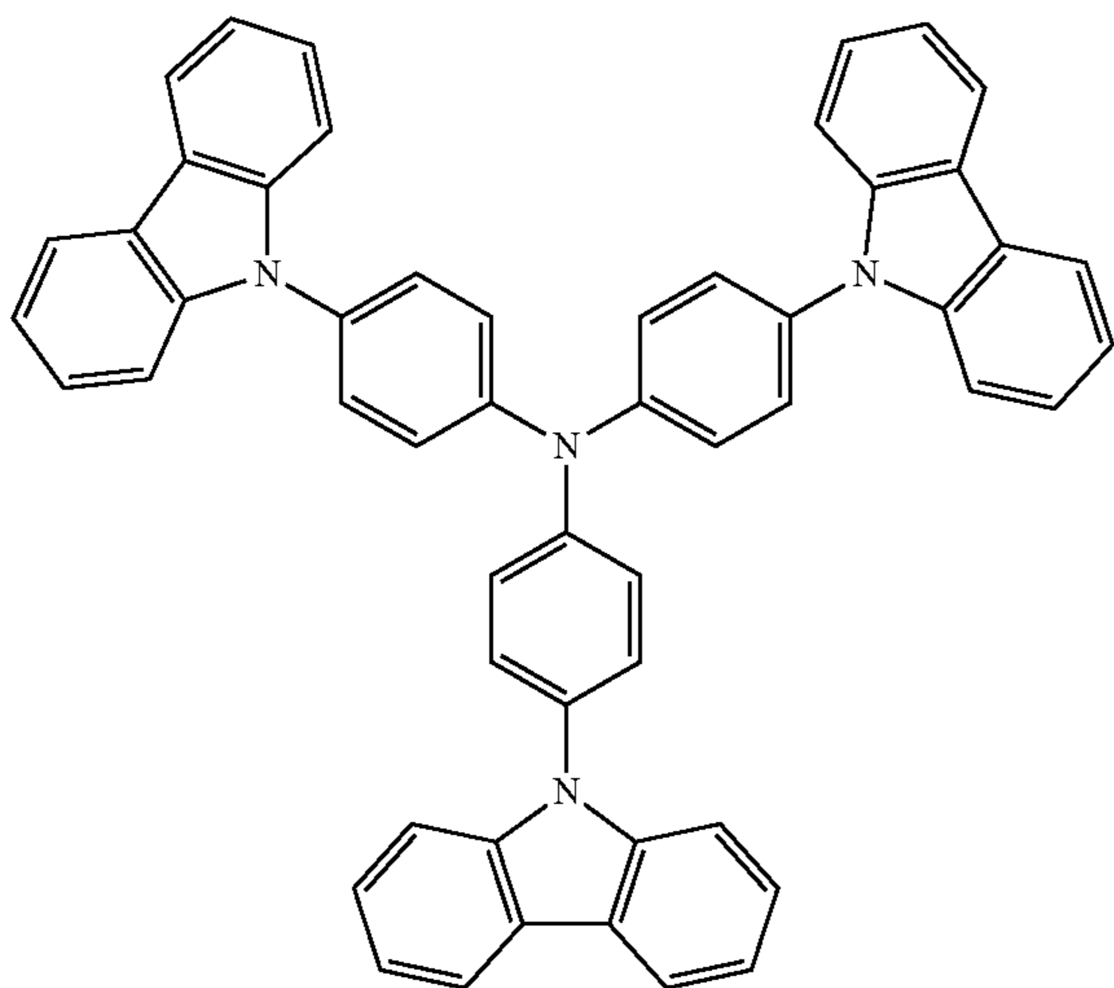
TCTA
