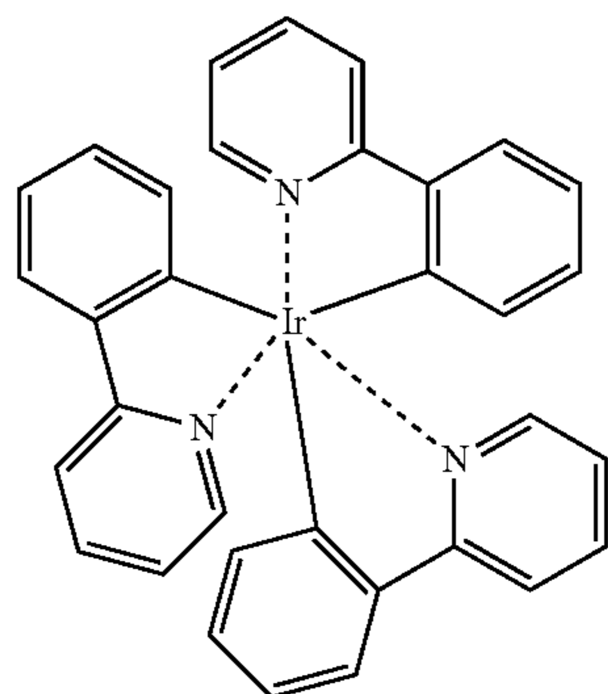
Ir(ppy) 3
