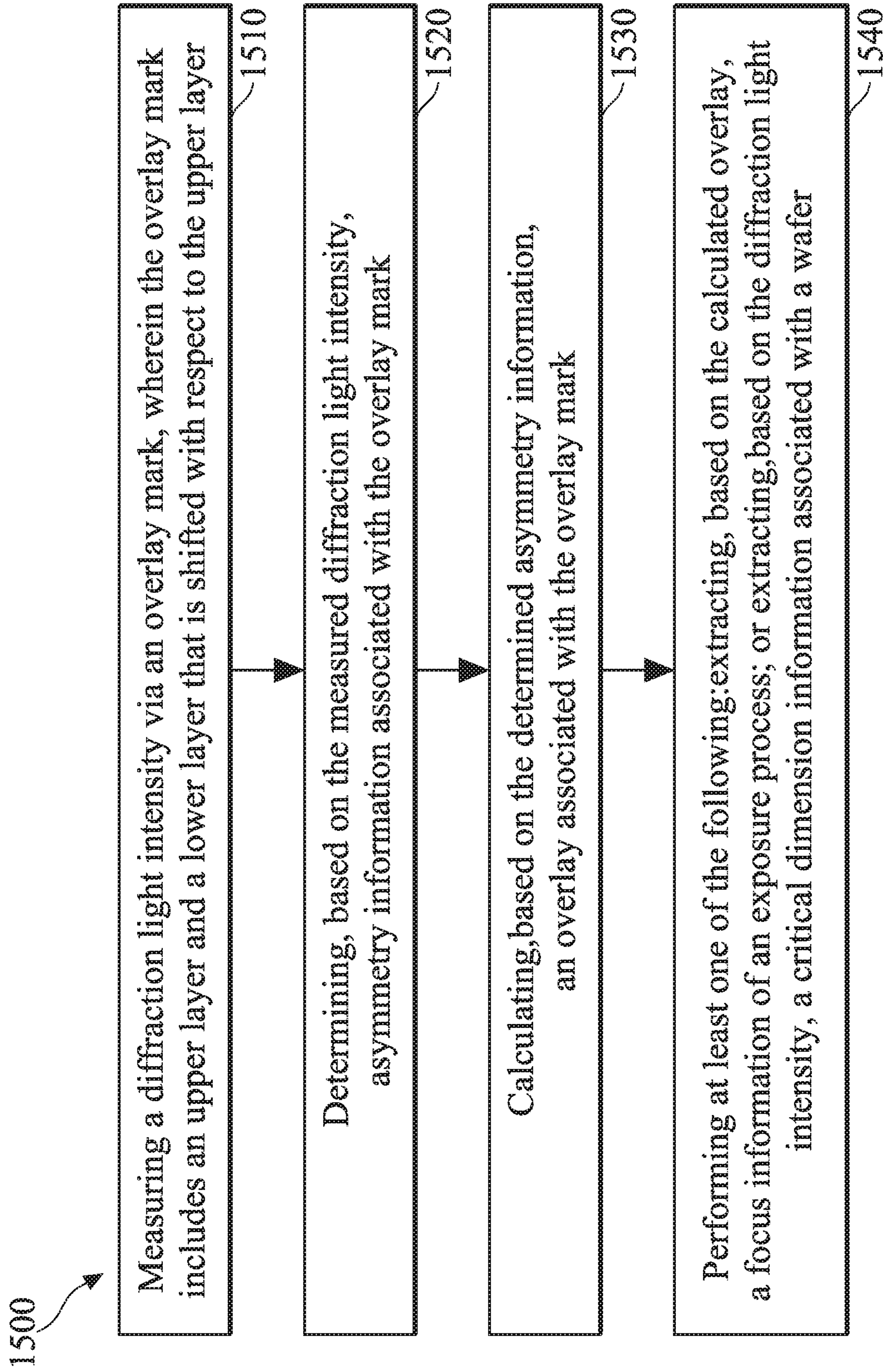
FIG. 24
