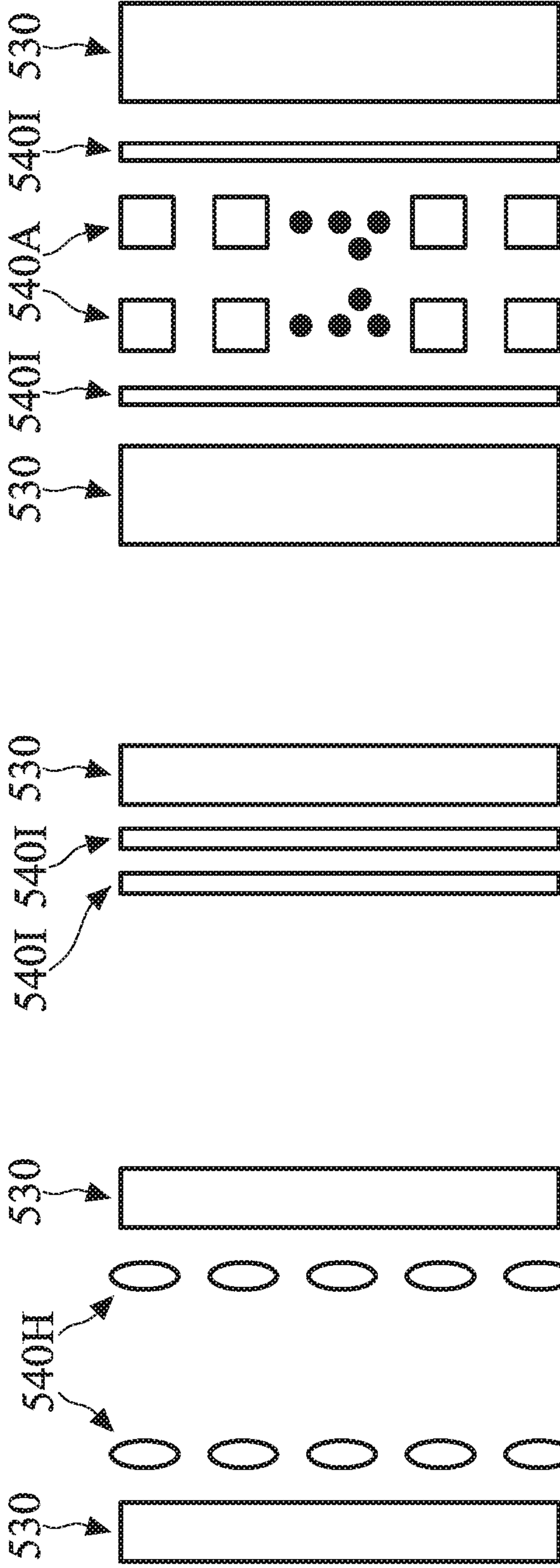
FIG. 18A
