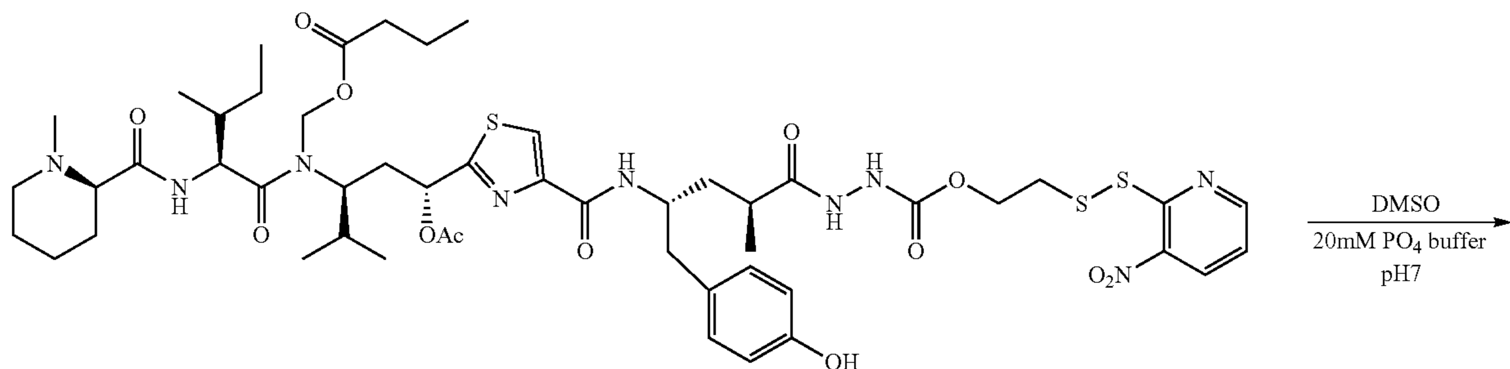
D-Asp-D-Asp
