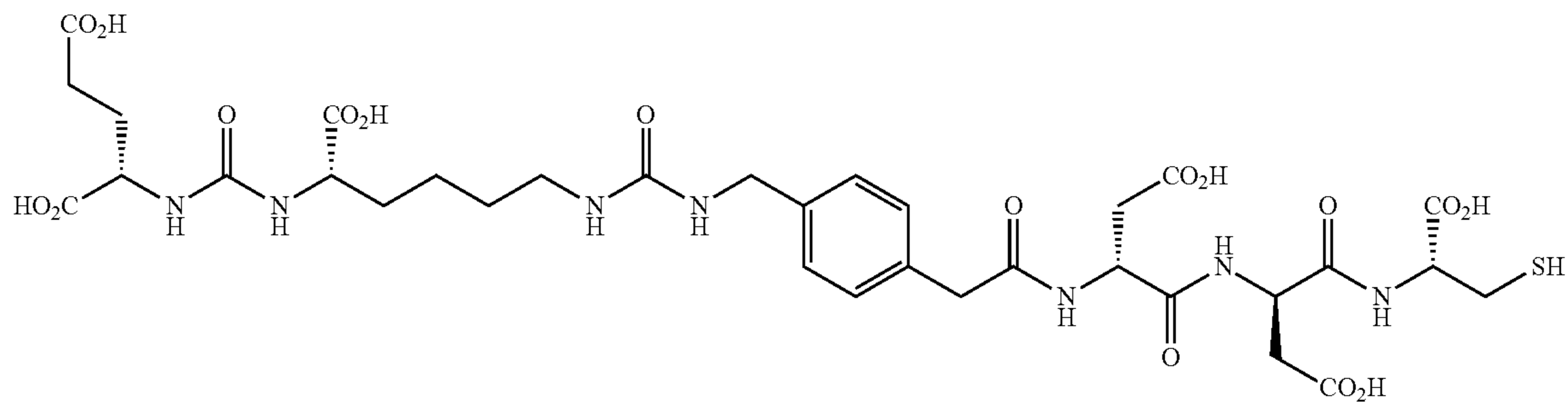
D-Asp-D-Asp
