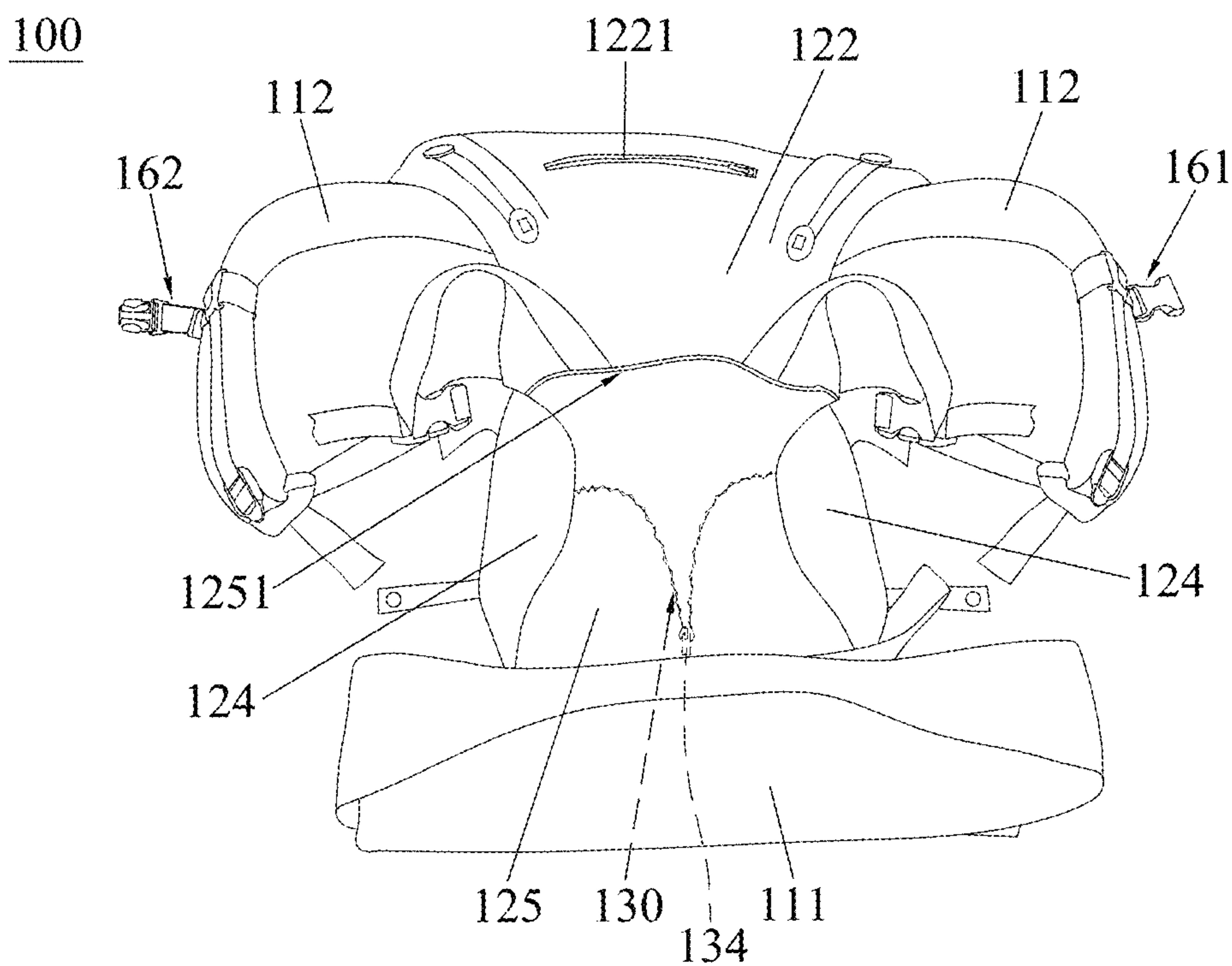
FIG. 12
