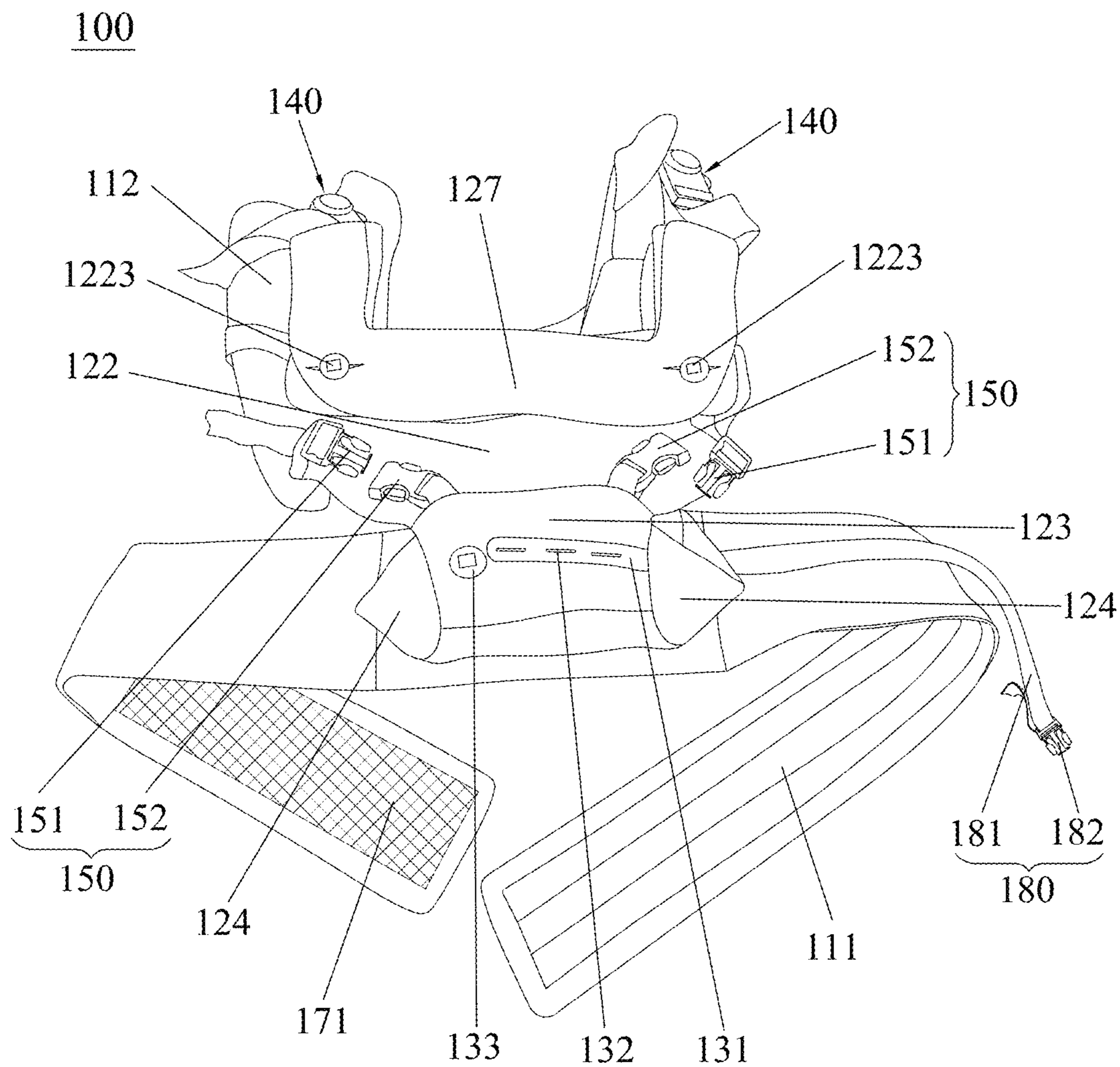
FIG.20
