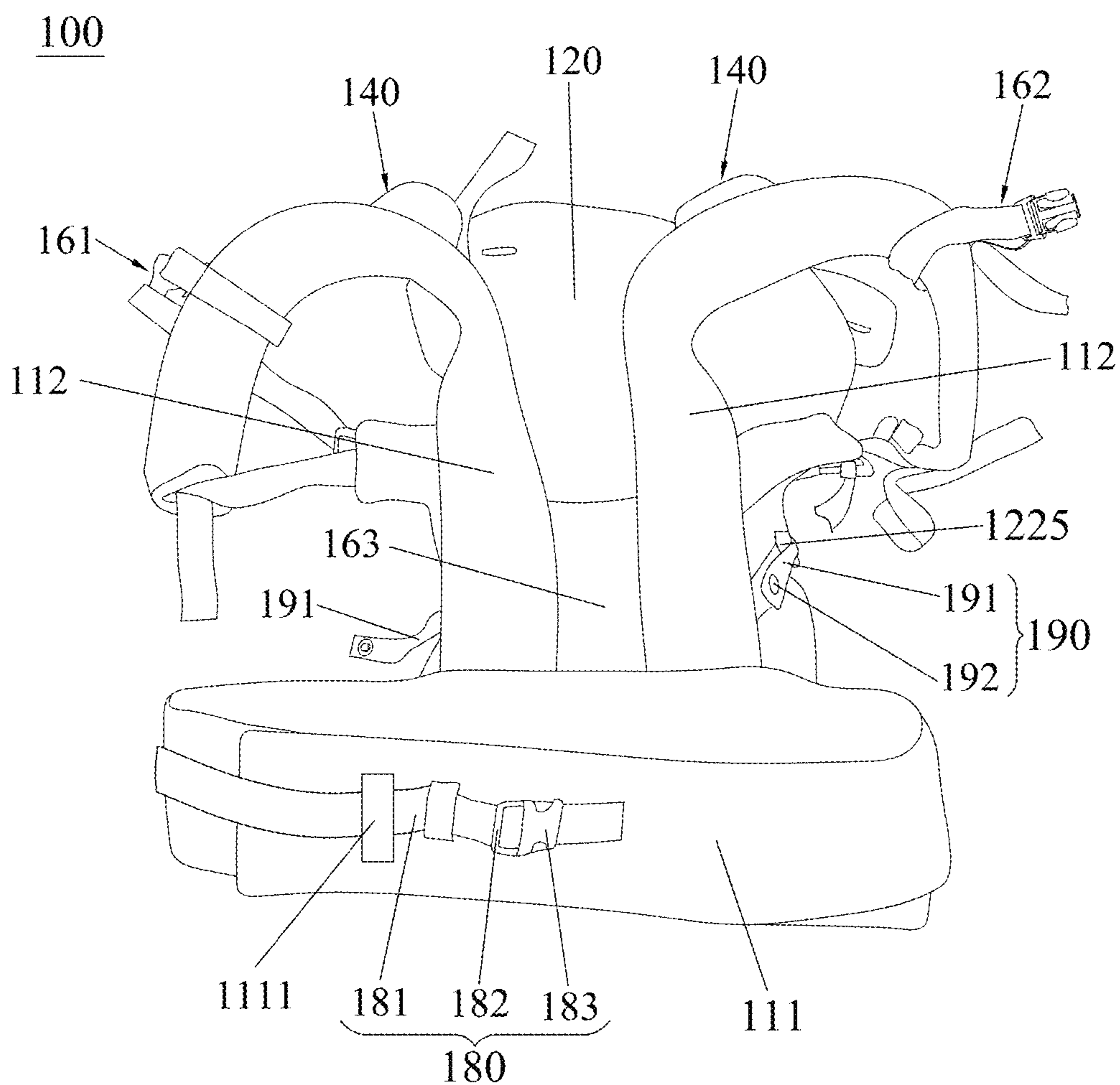
FIG. 15
