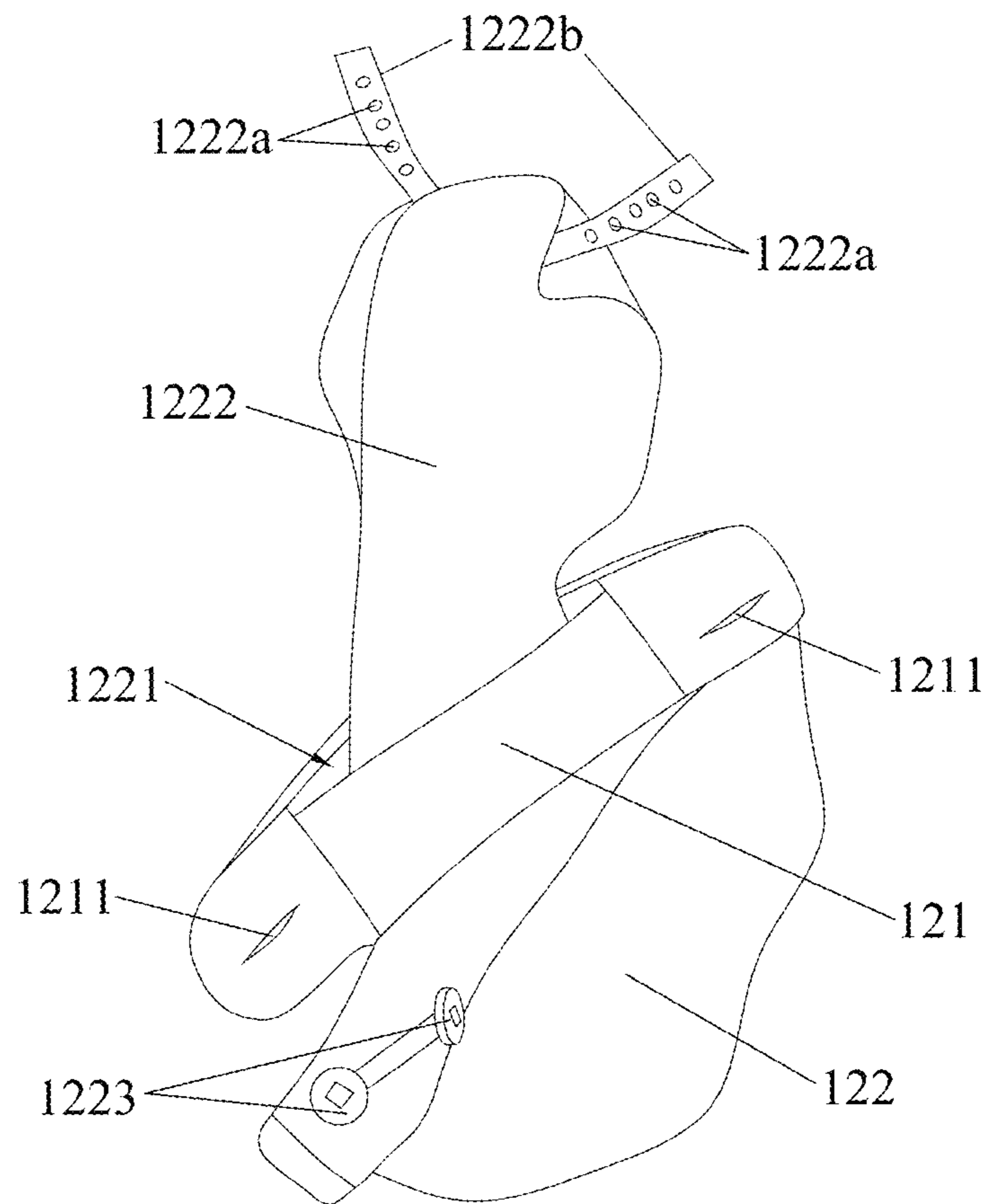
FIG. 19
