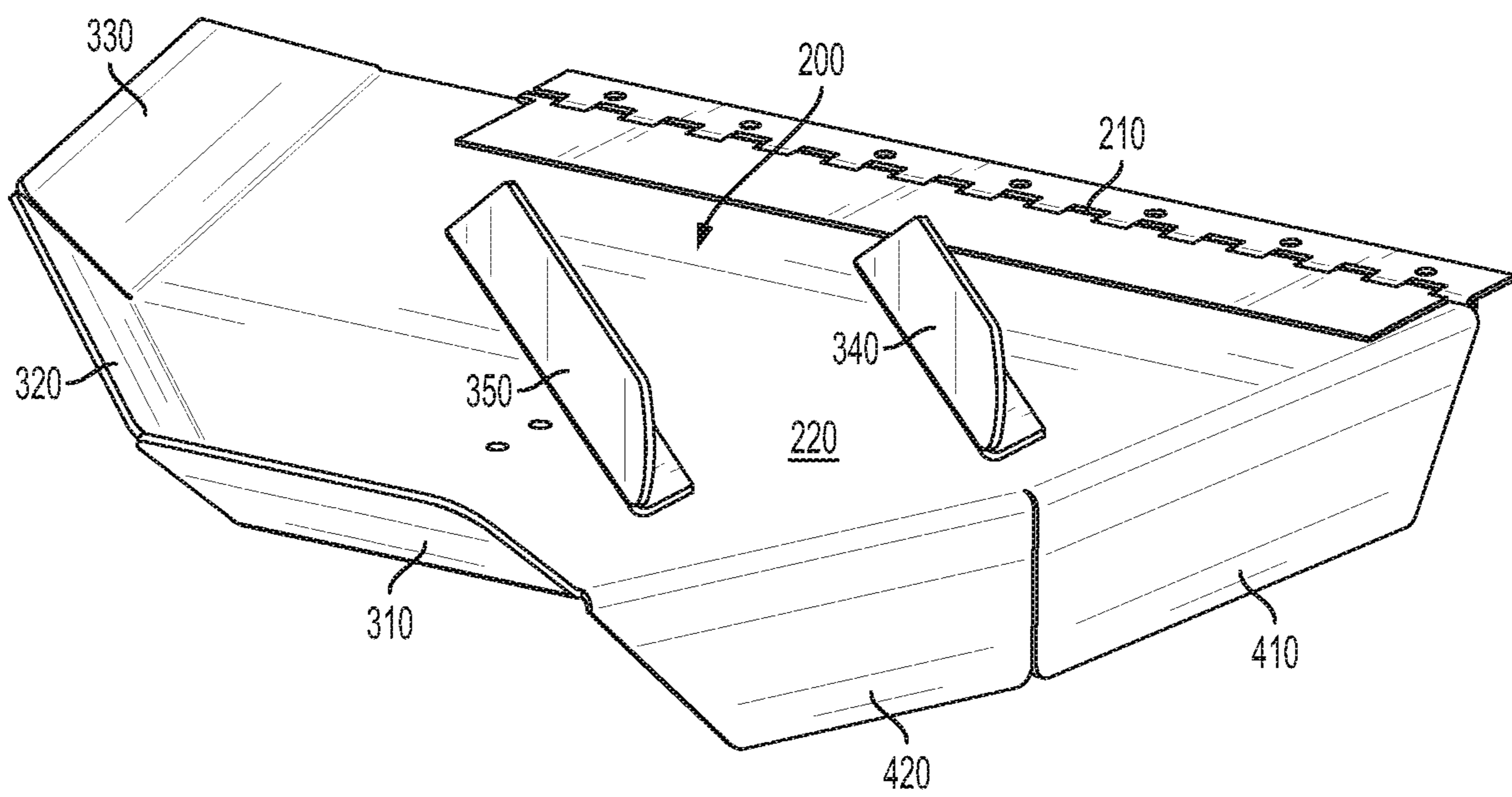
FIG. 63
