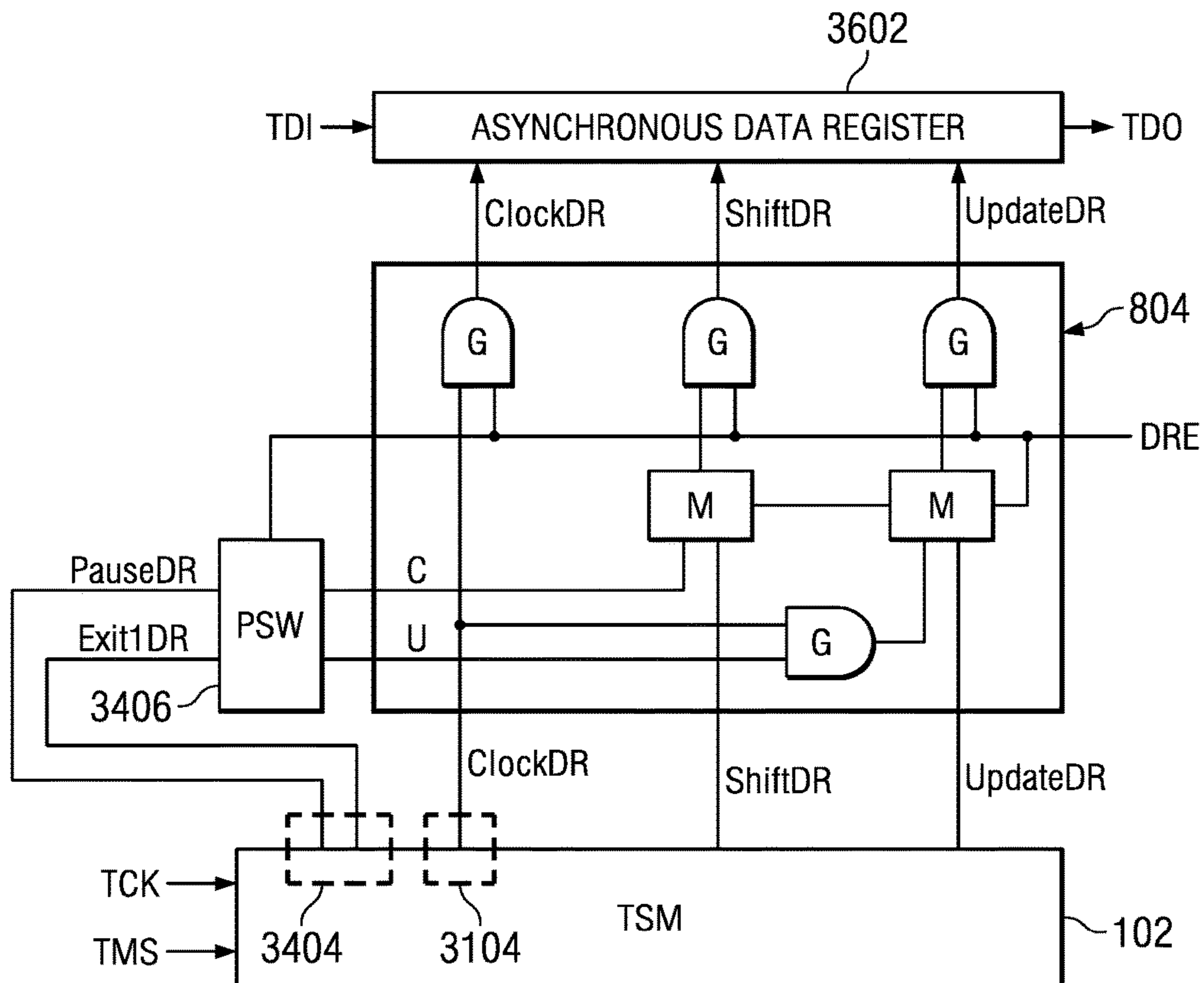
FIG. 36
