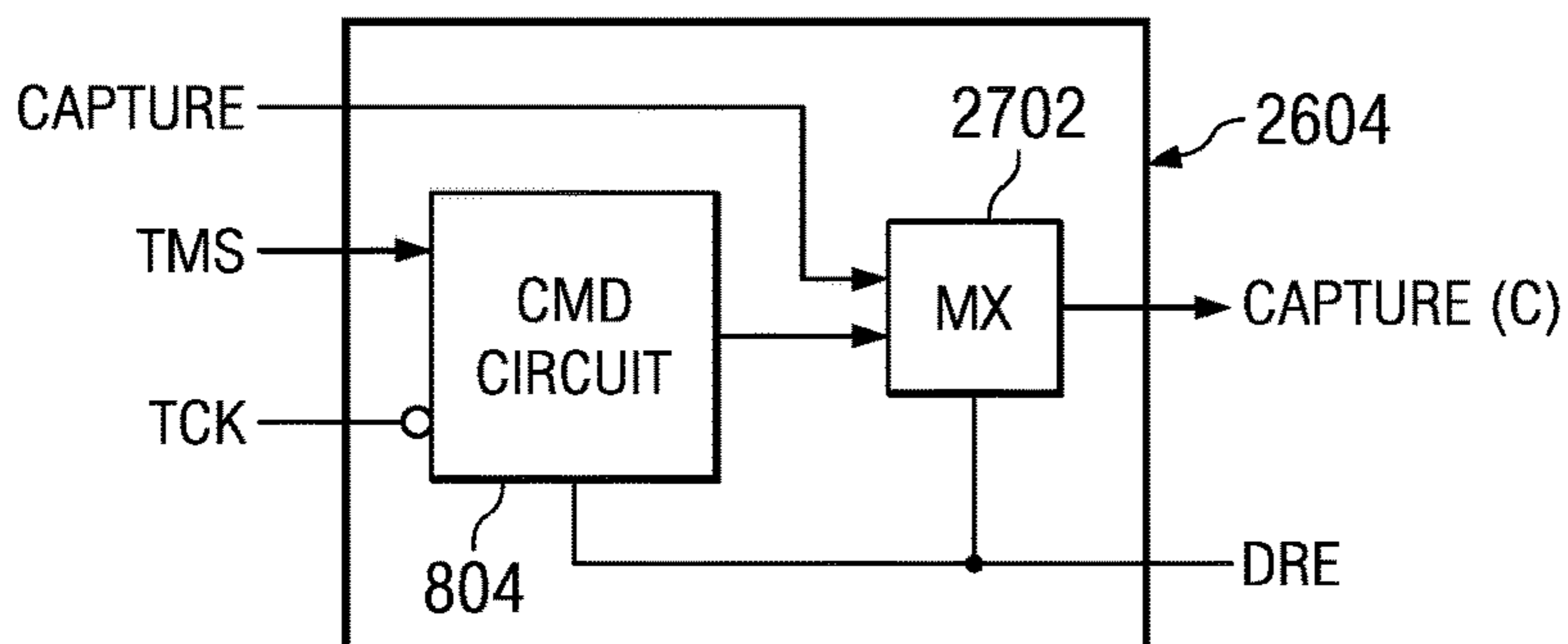
FIG. 27
