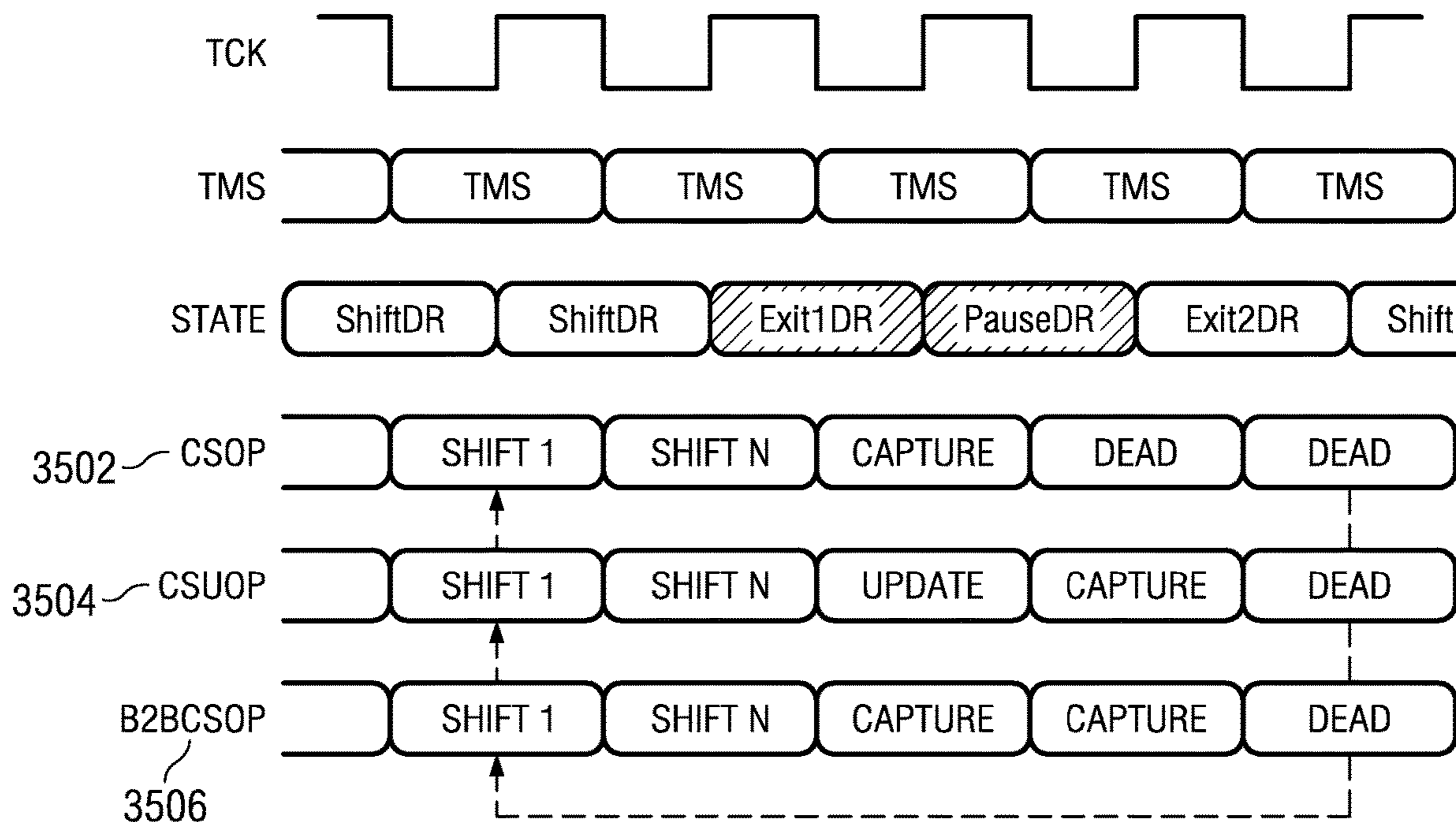
FIG. 35
