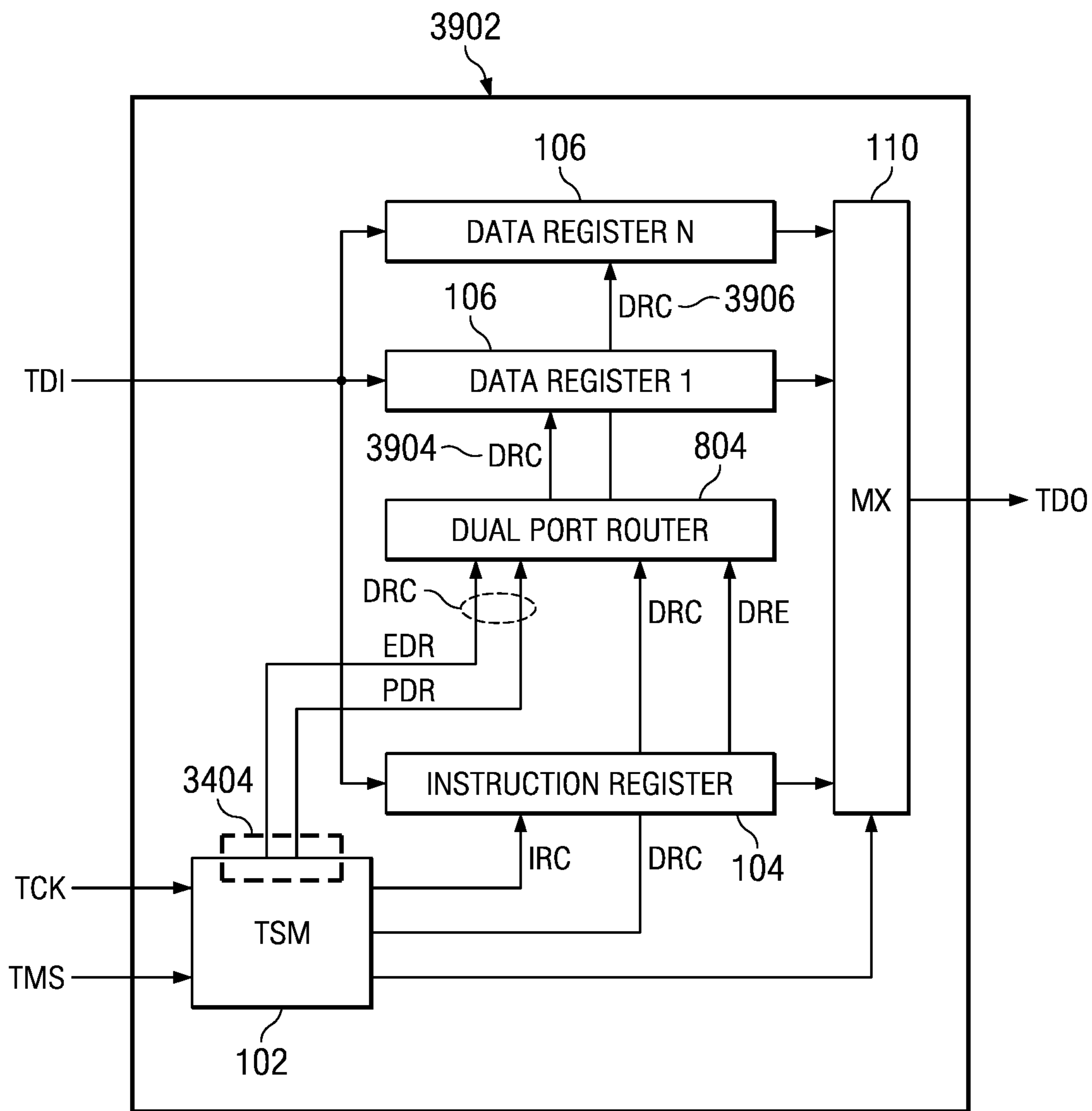
FIG. 39
