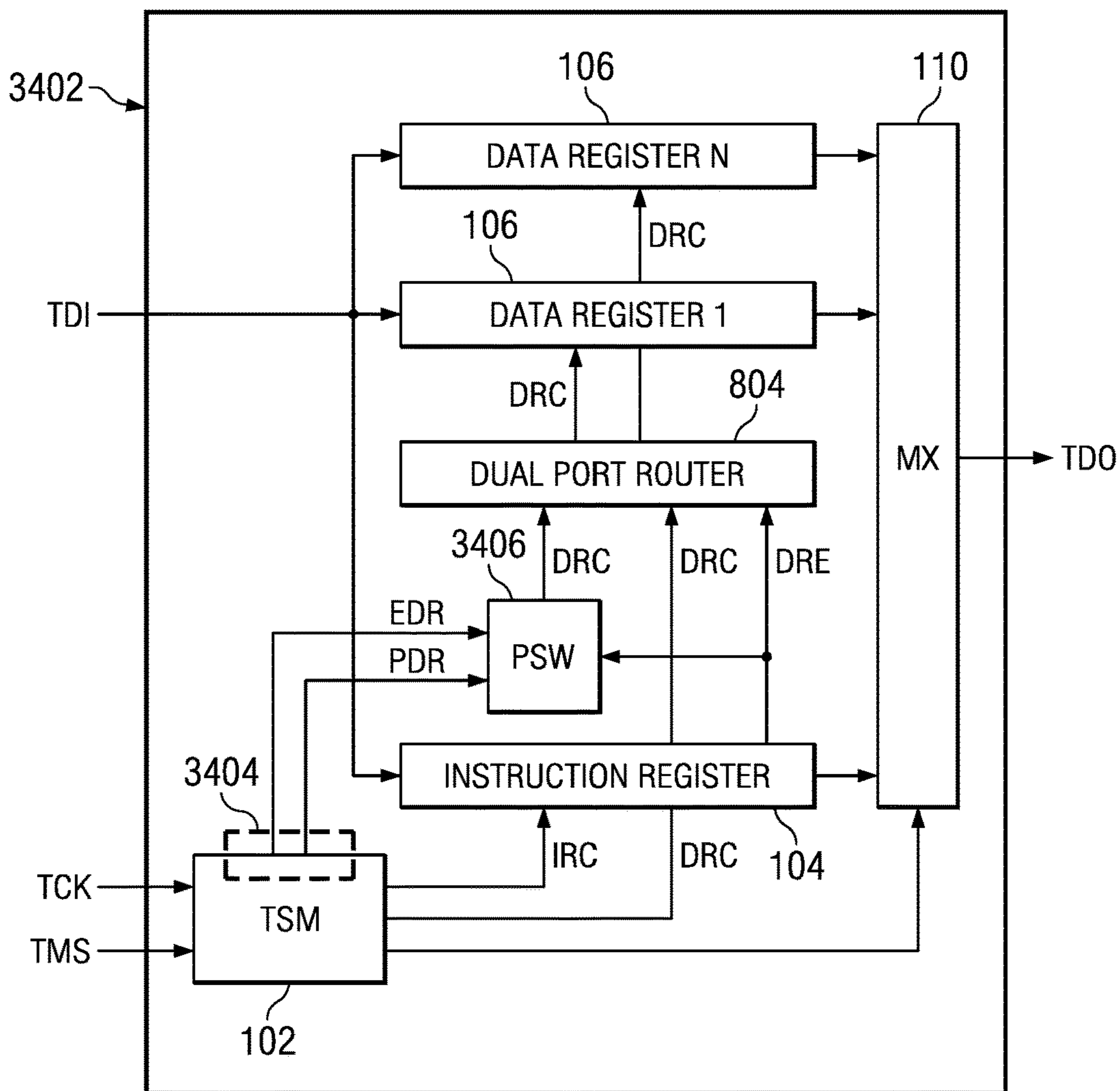
FIG. 34A
