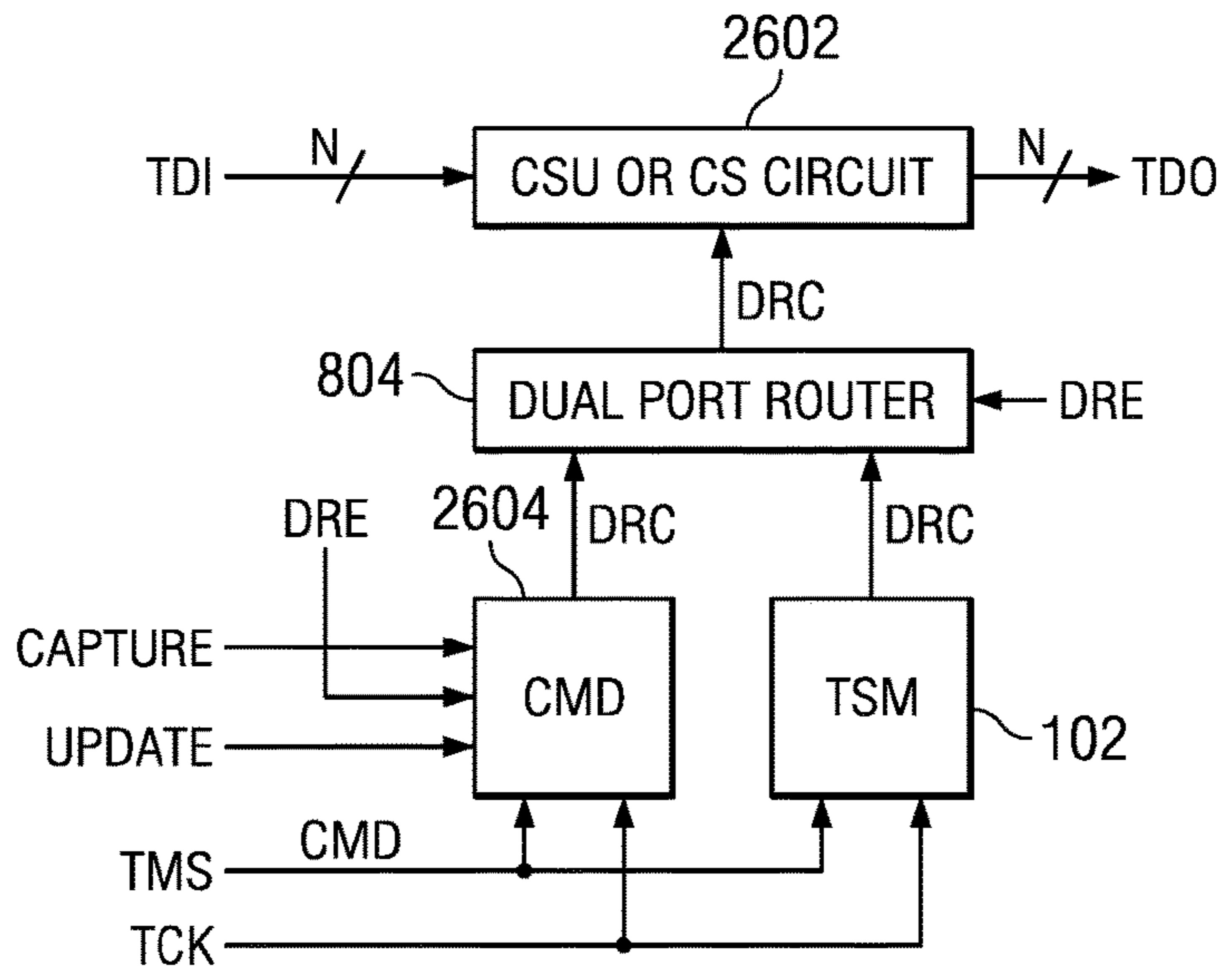
FIG. 26
