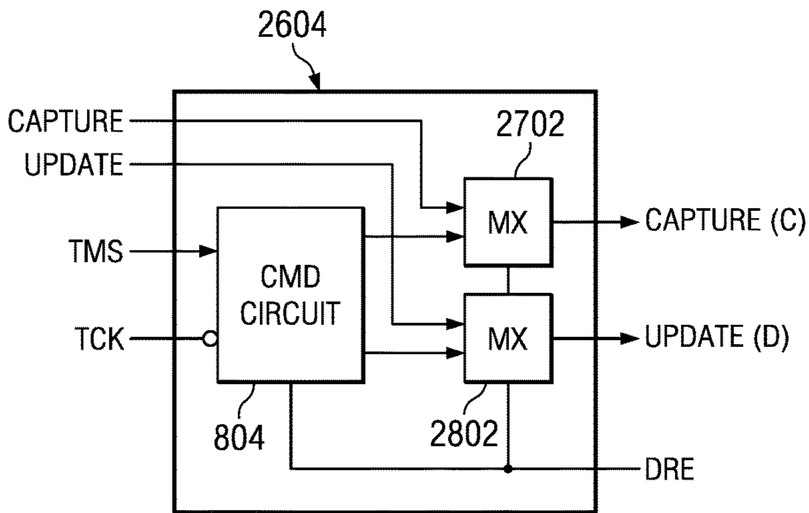
FIG. 28
