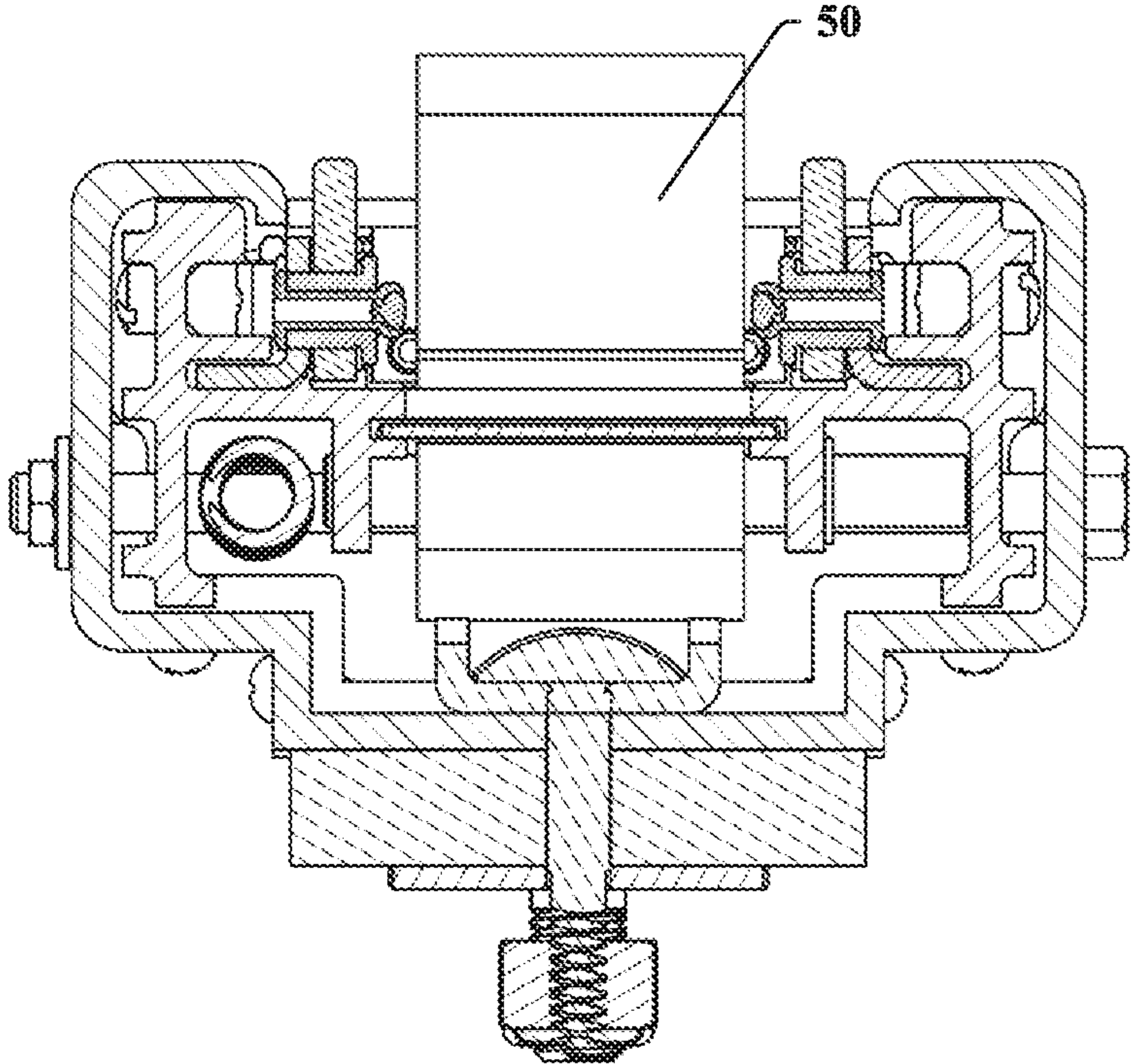
FIG. 16
