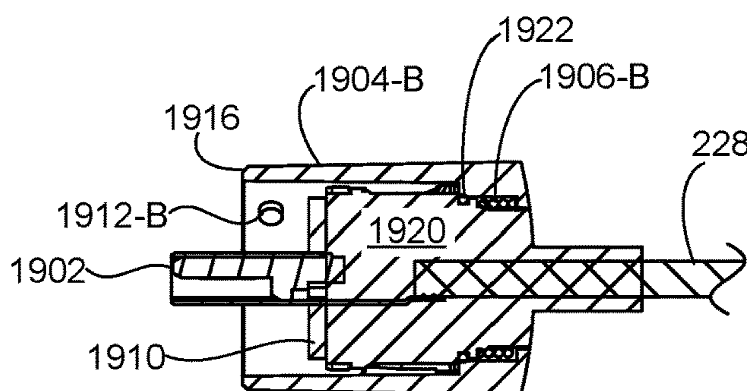
SECTION V-V
