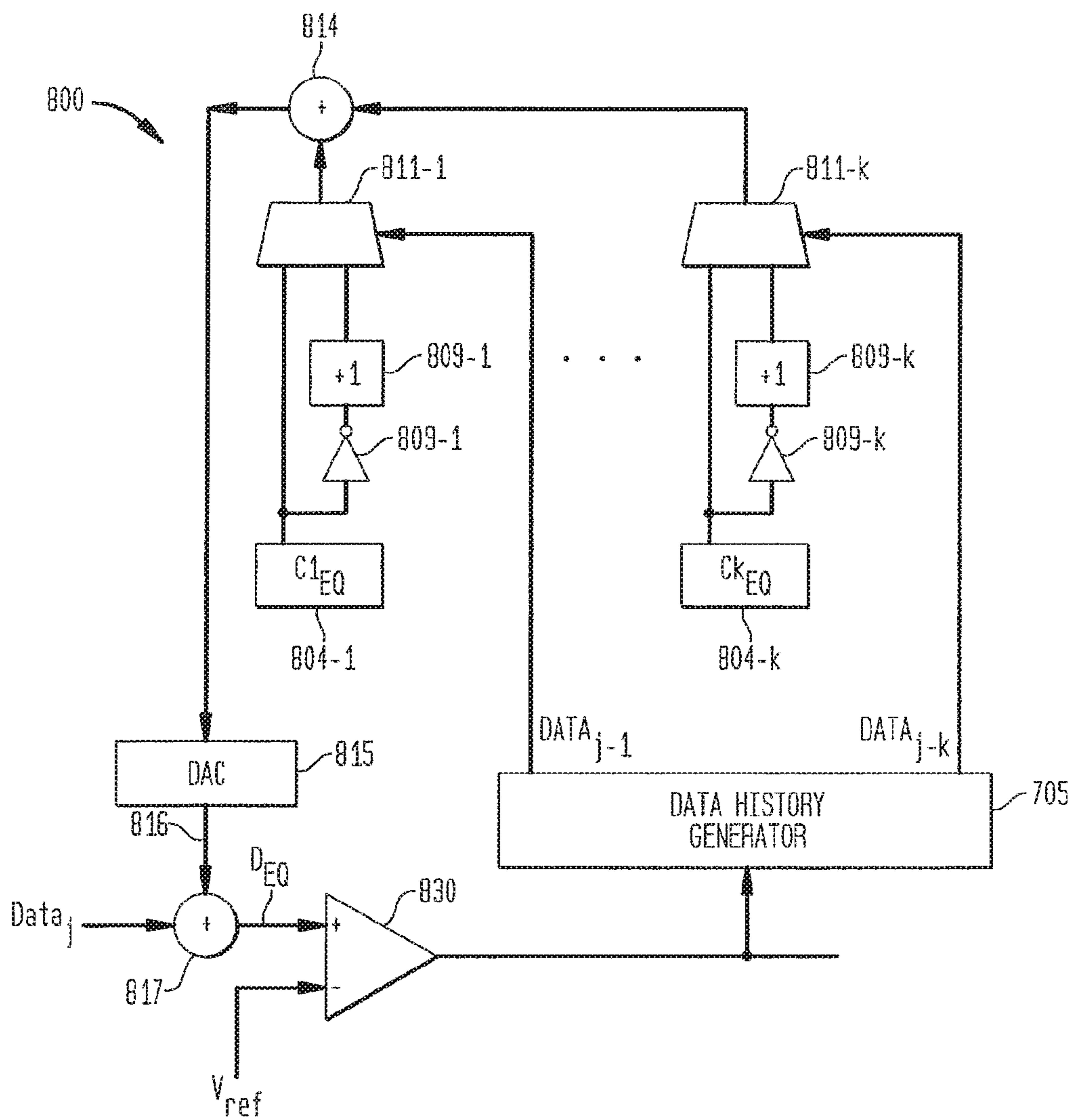
FIG. 17
