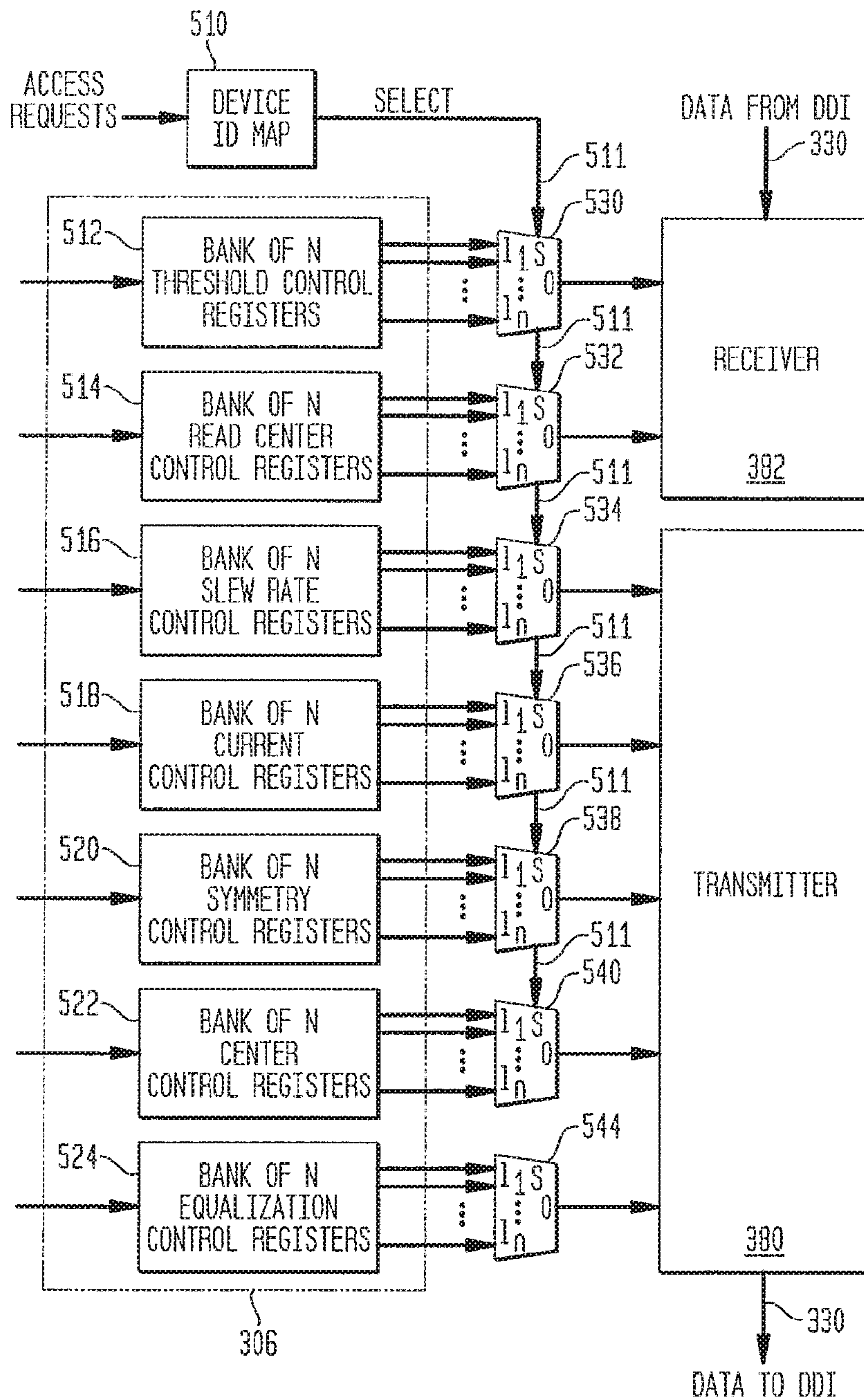
FIG. 16
