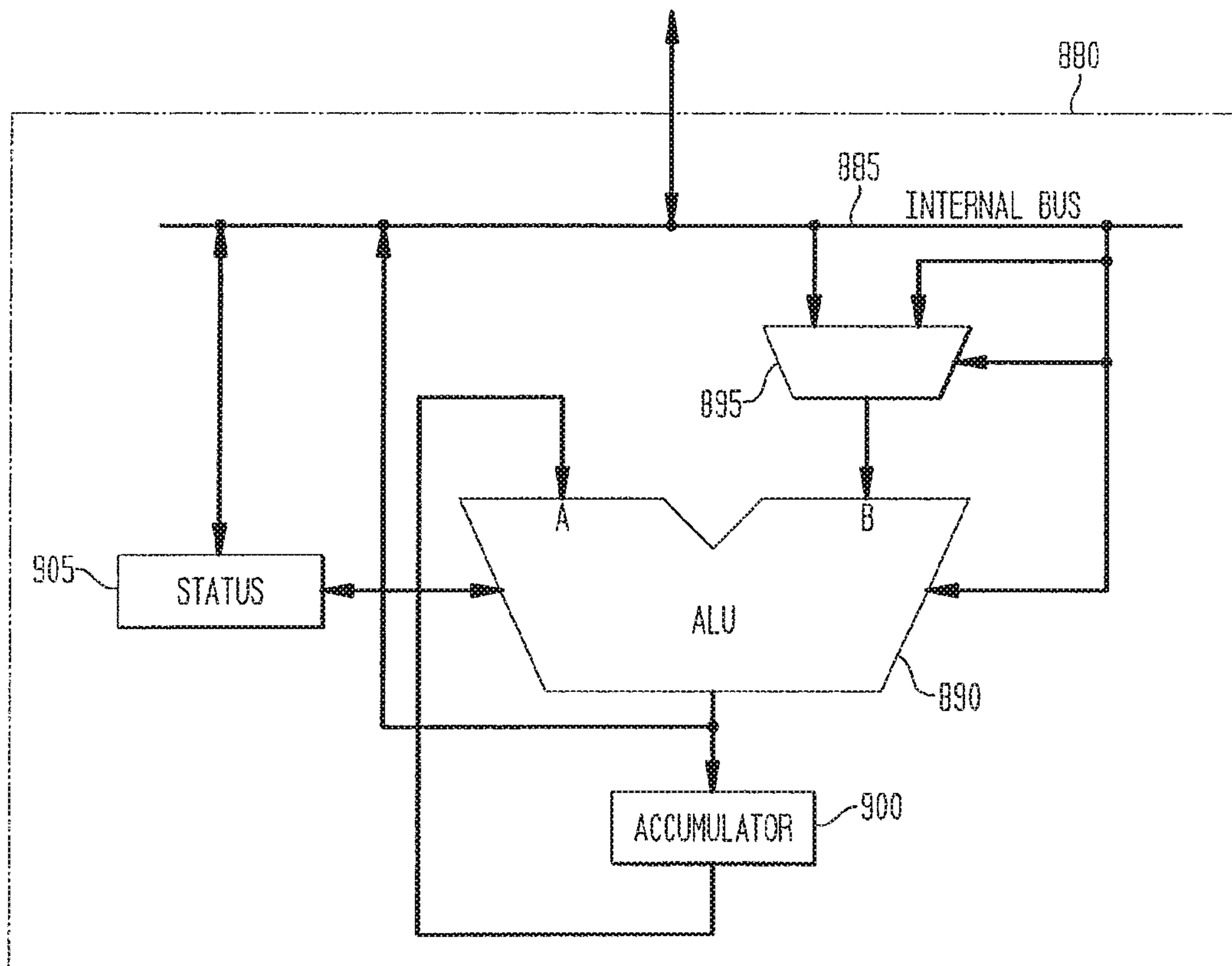
FIG. 20
