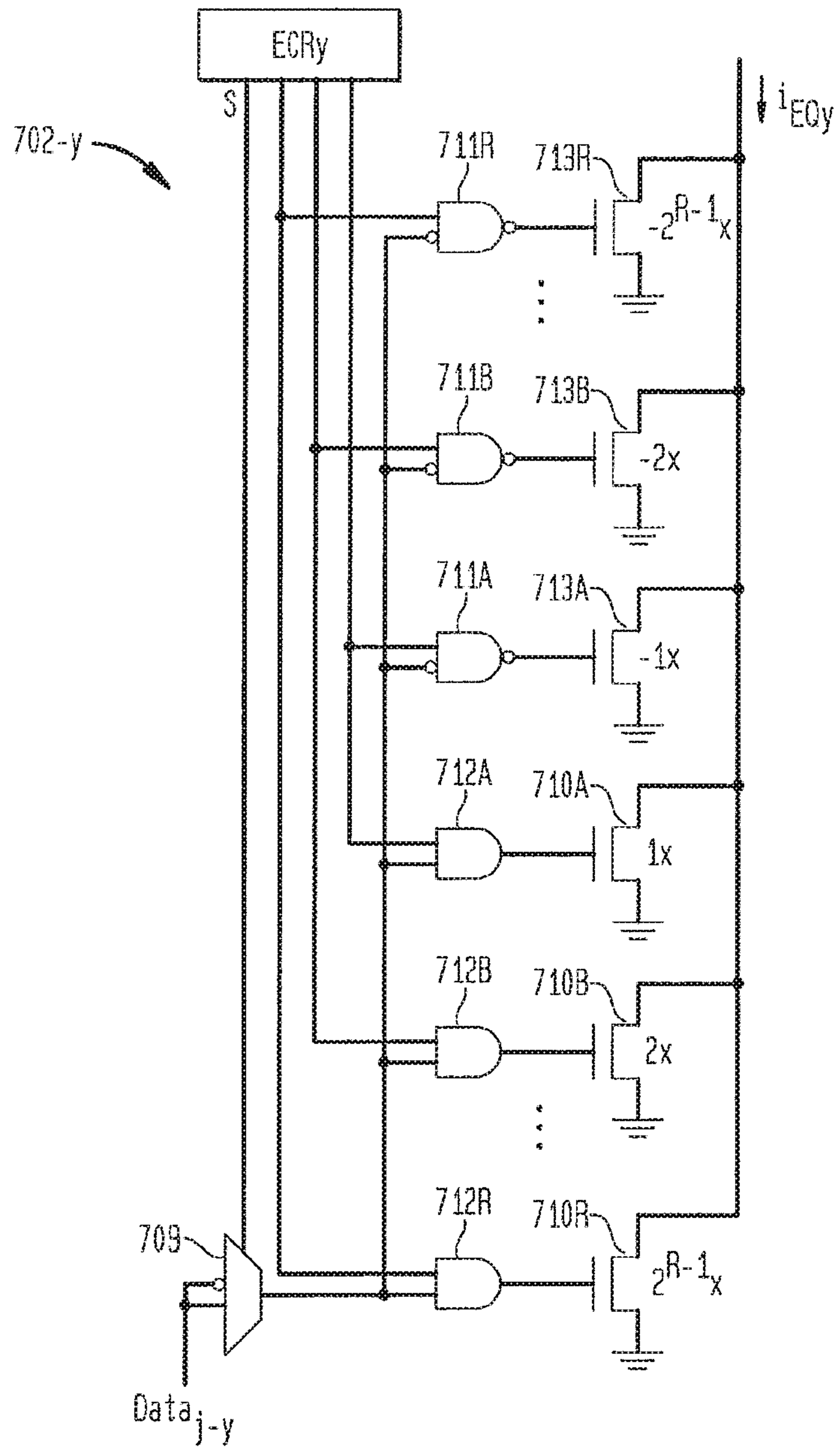
FIG. 18B
