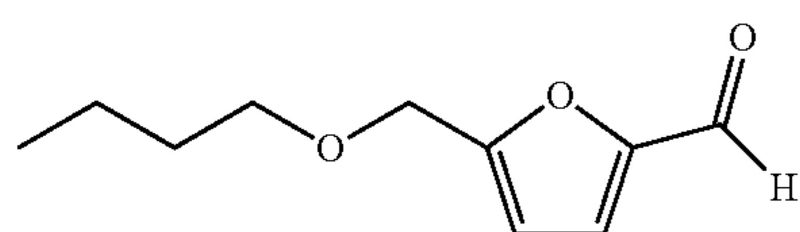
5-butoxymethylfurfural
