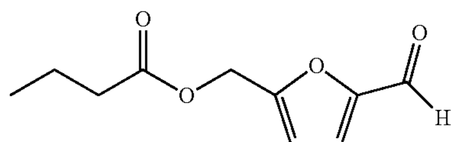
5-butyroxymethylfurfural
