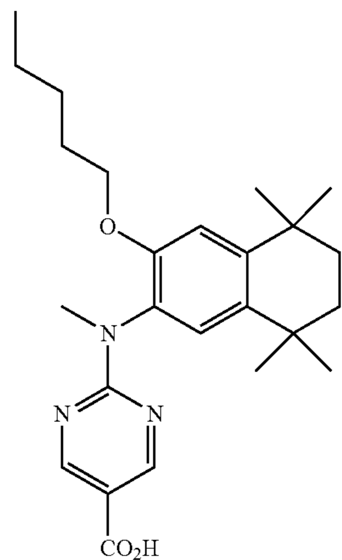
PA 451
