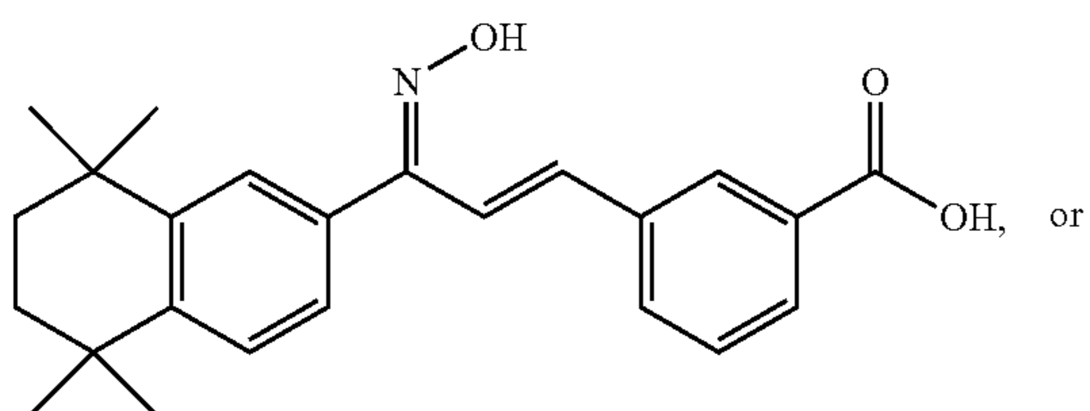
AGN 204647
