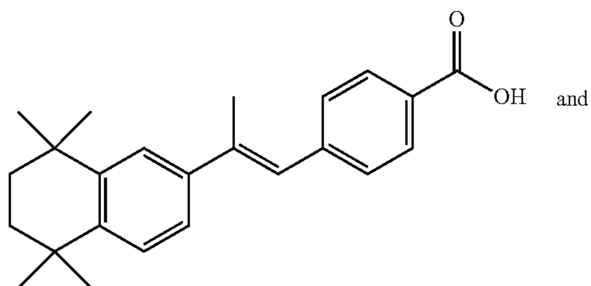
AGN 190183
