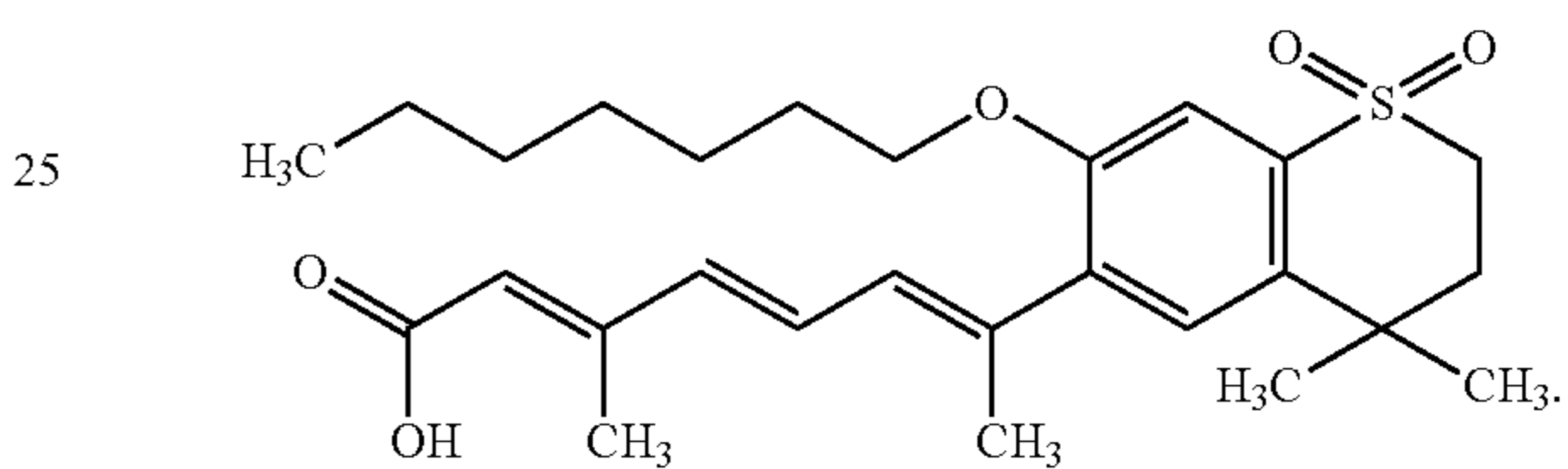
Ro46-5471
