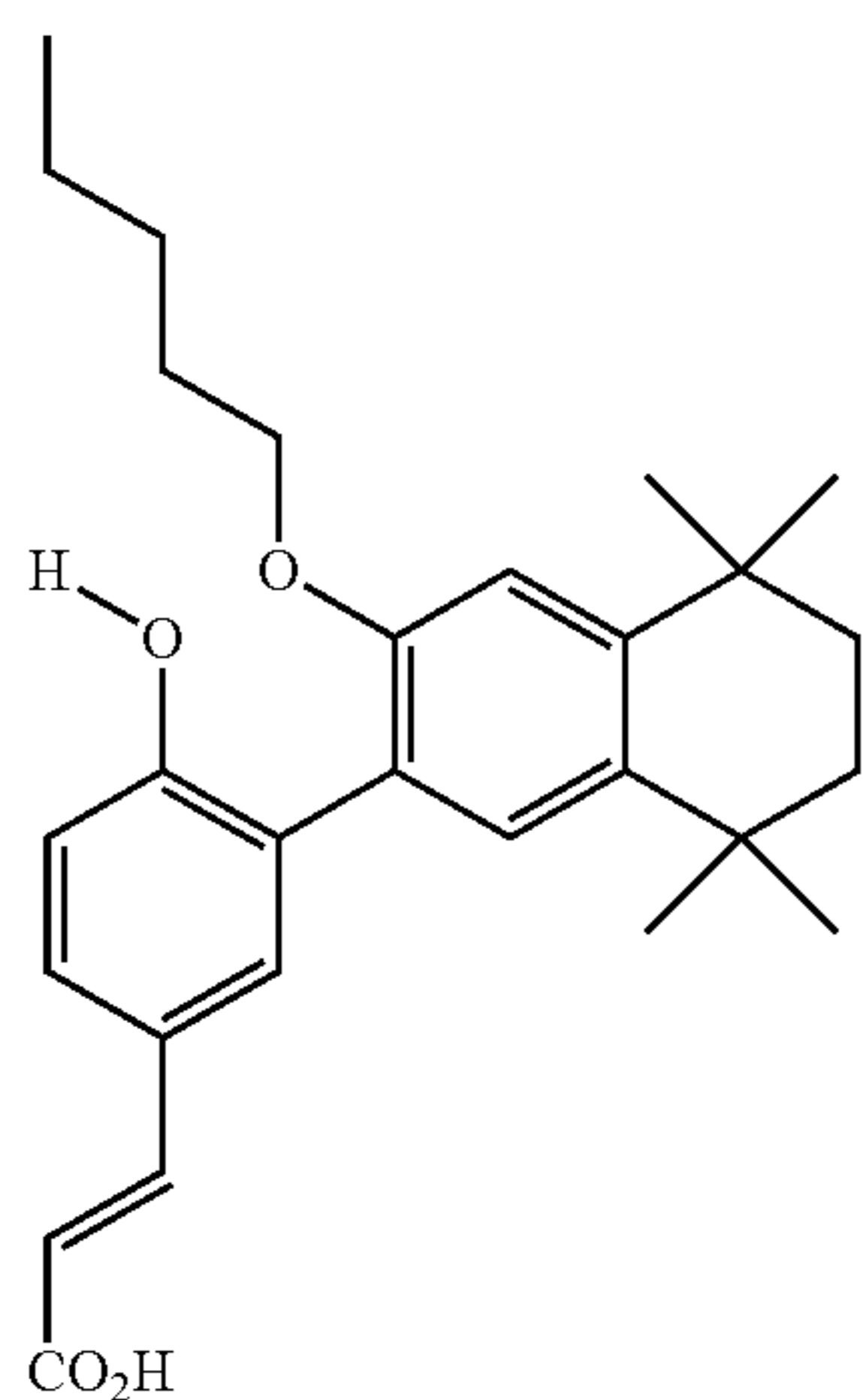
UVI 3003
