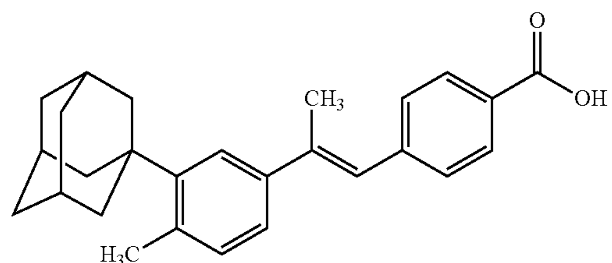
CD2325
