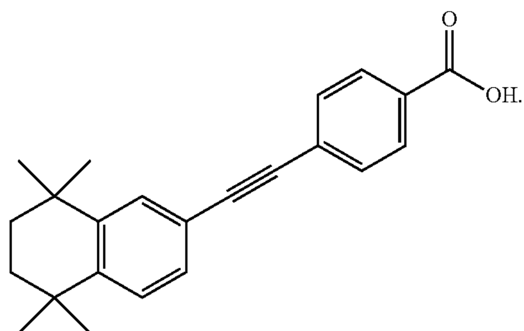
AGN 190205
