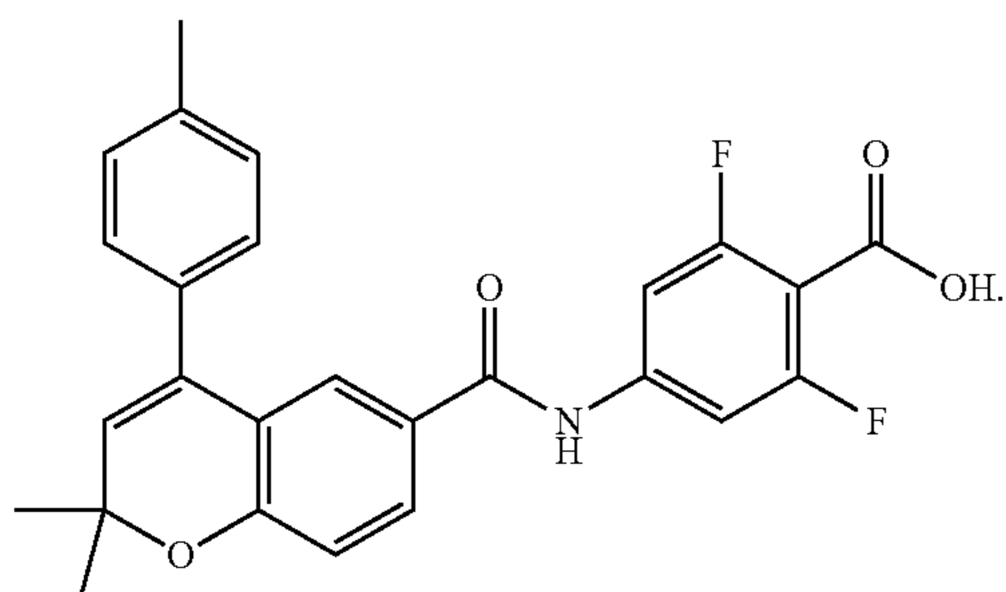
AGN 194574
