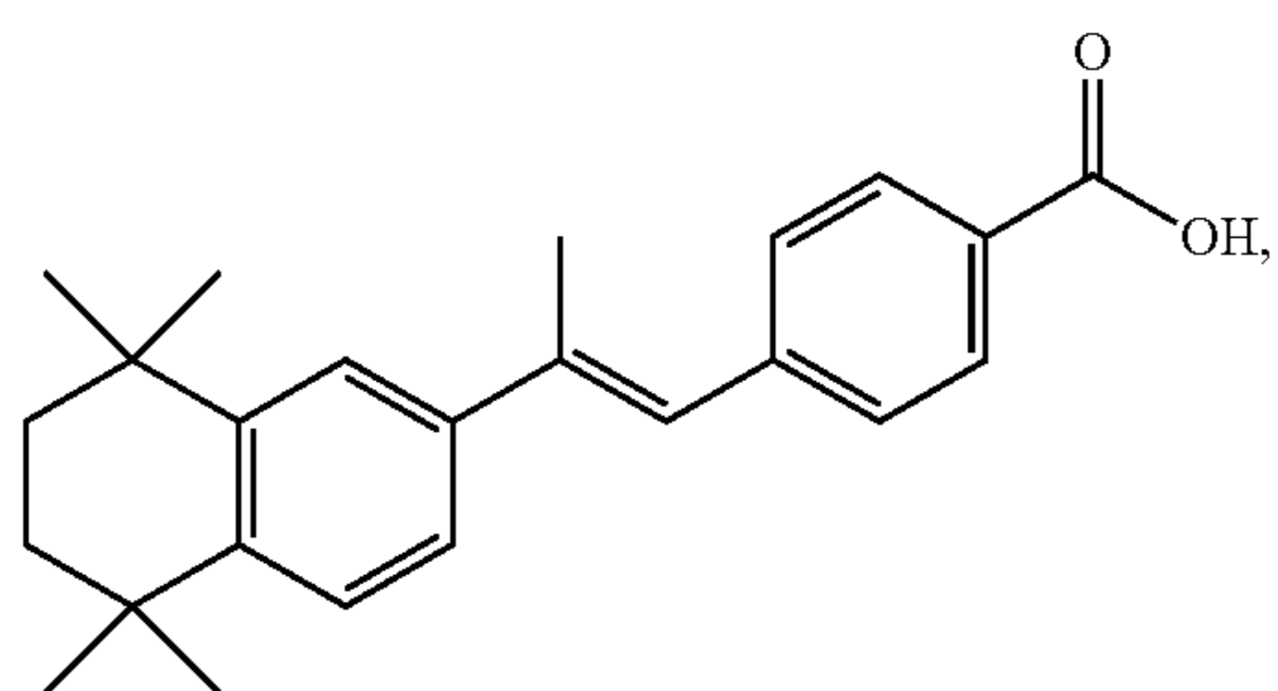
AGN 190183
