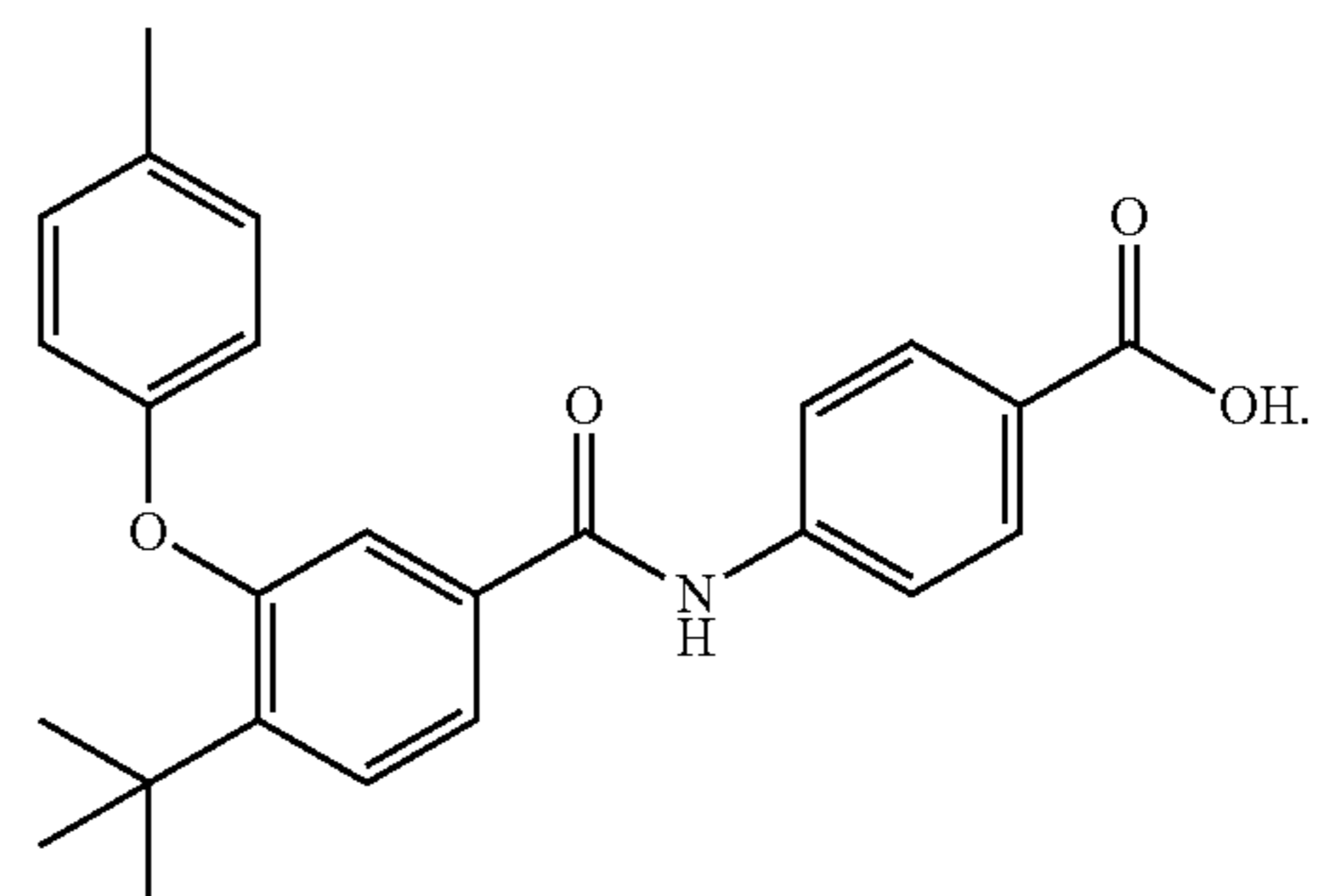
AGN 194777
