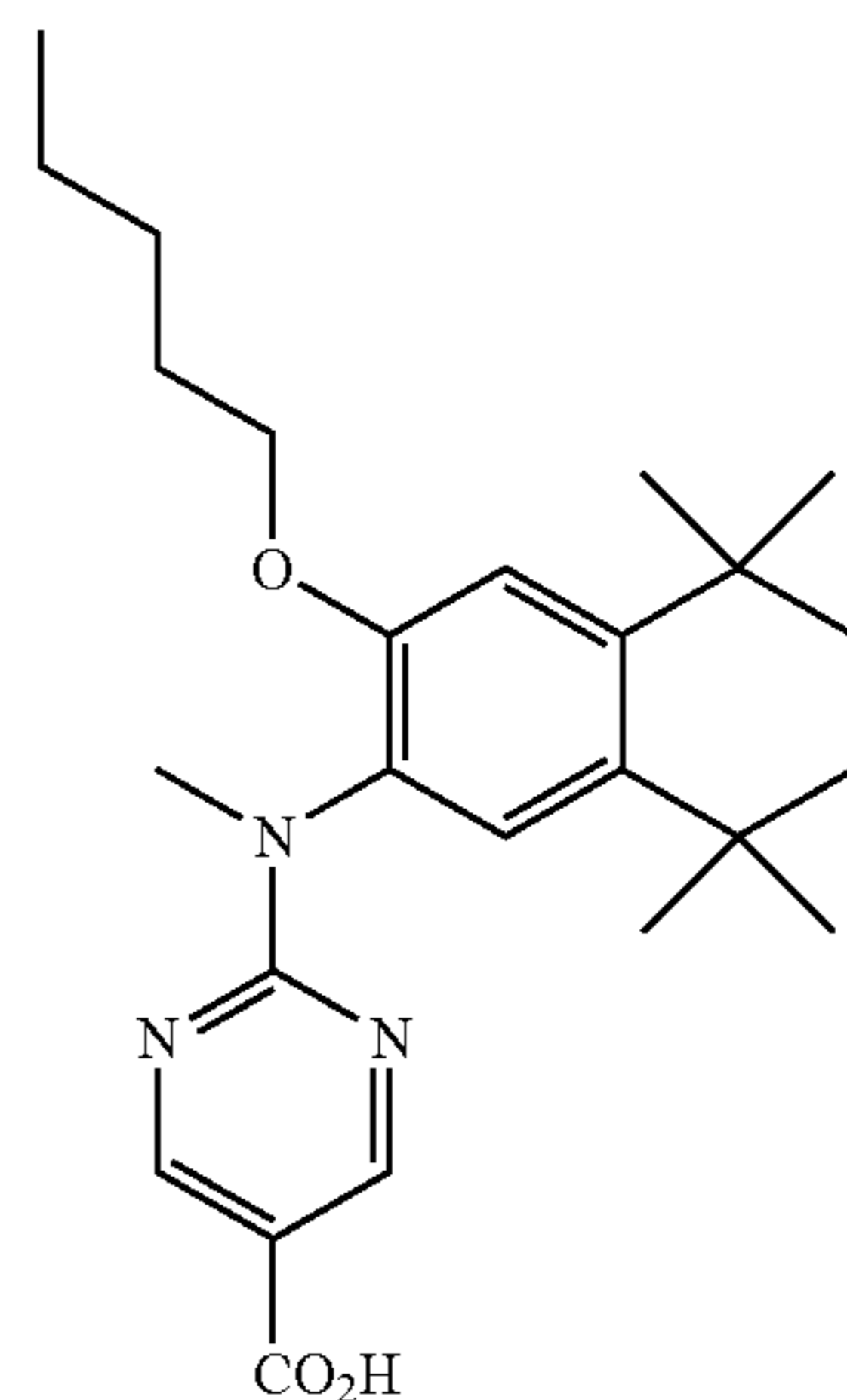
PA 451
