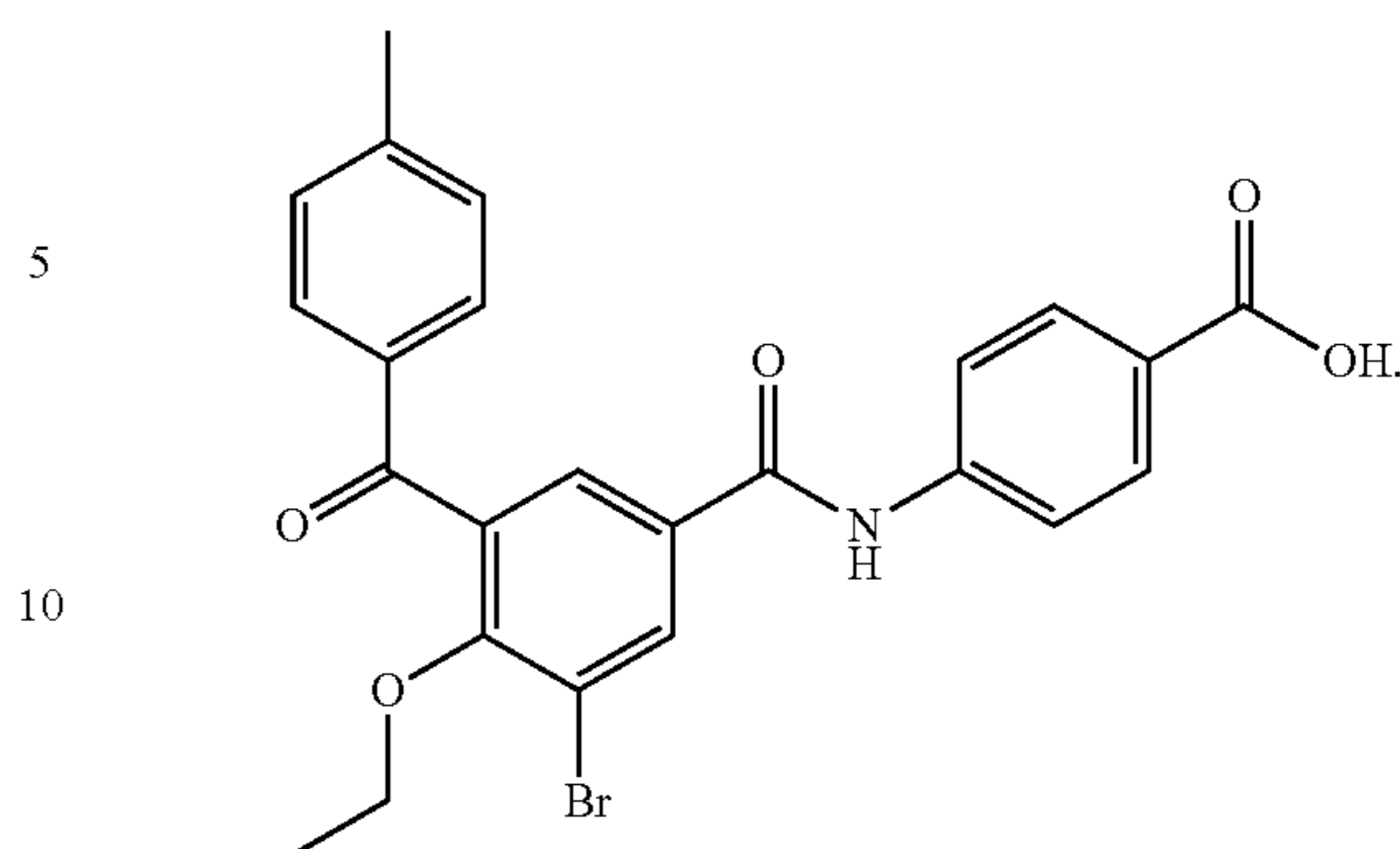
VTP 196696
