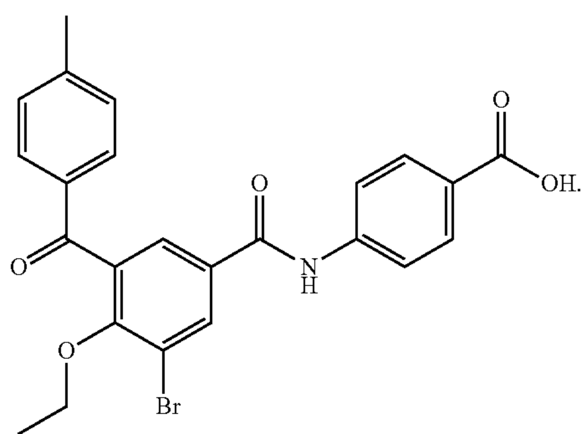
VTP 196696
