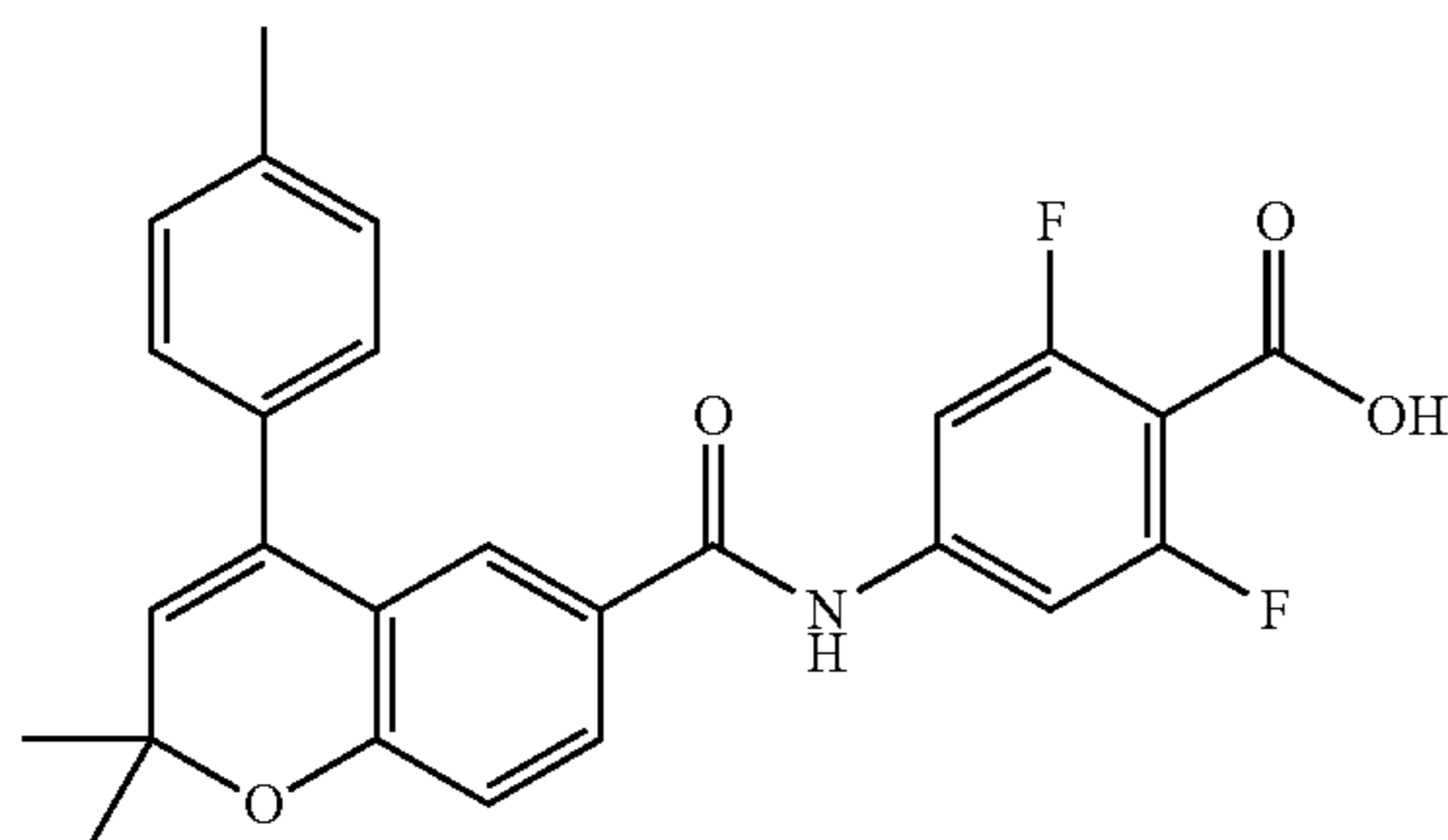
AGN 194574
