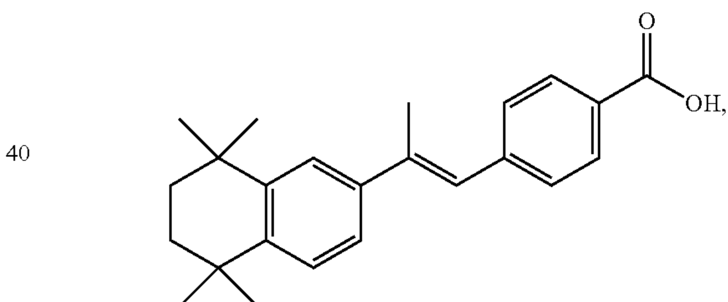
AGN 190183
