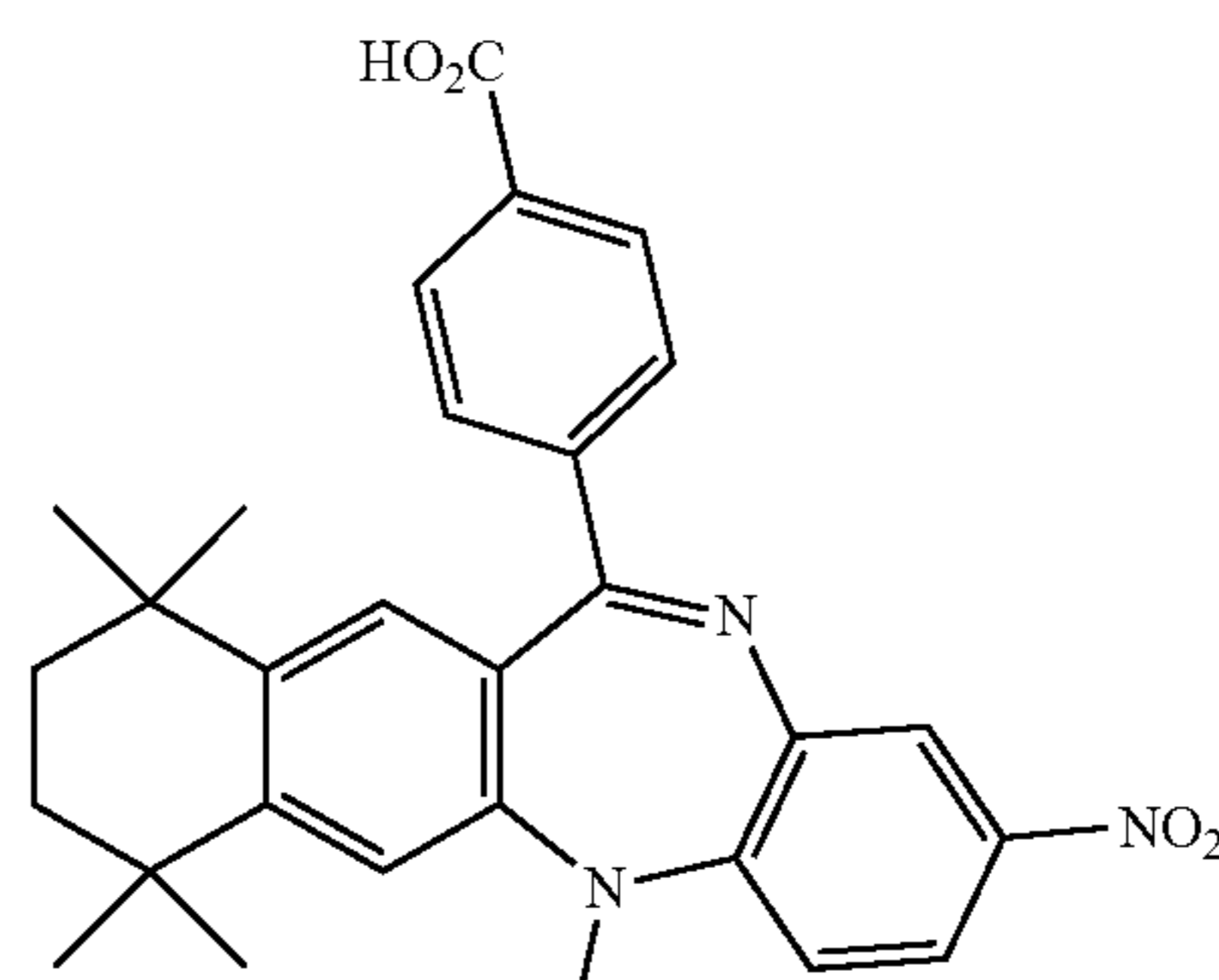
HX 531
