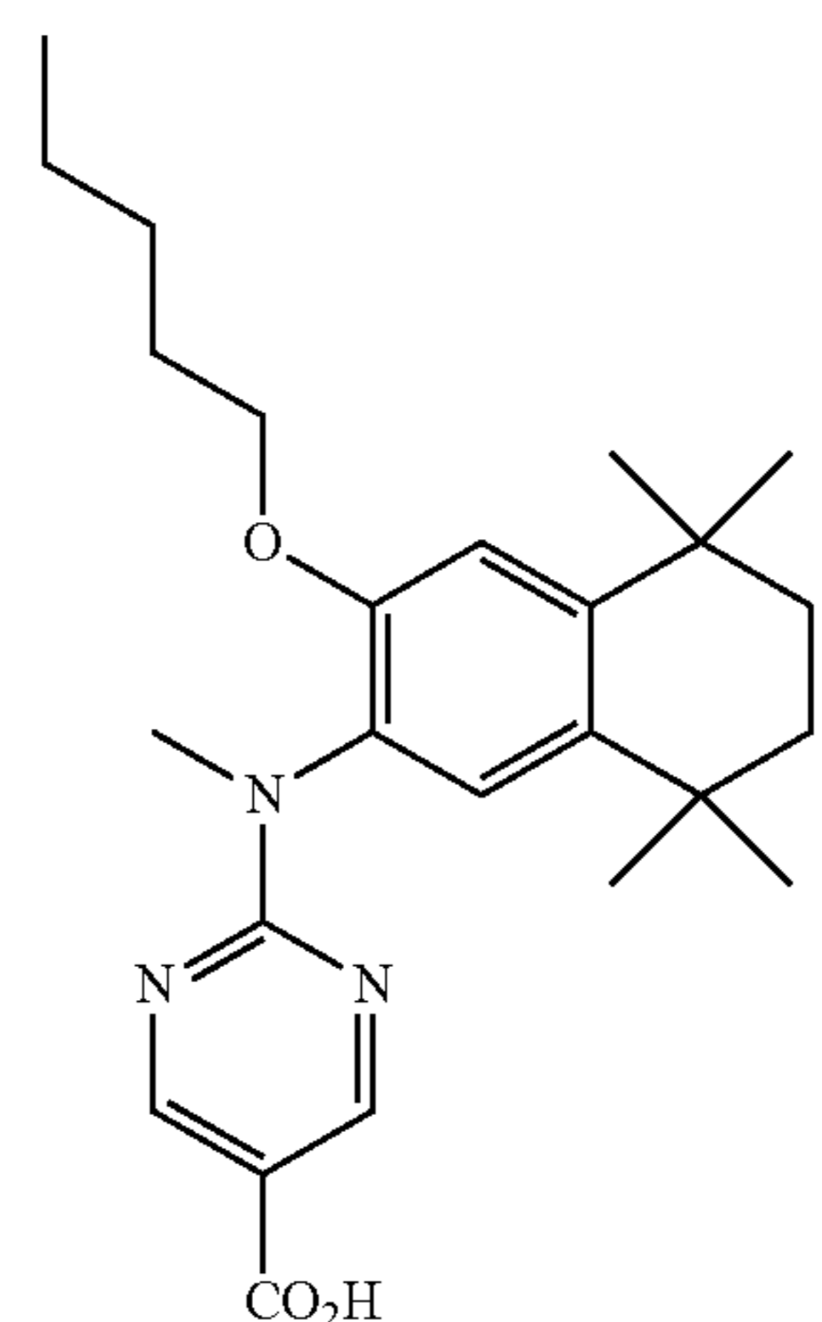
PA 451
