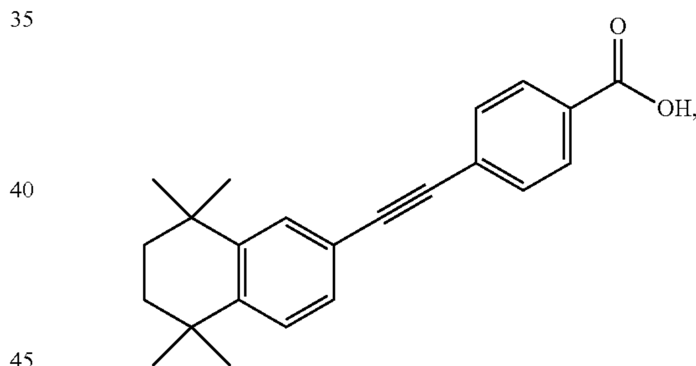
AGN 190183
