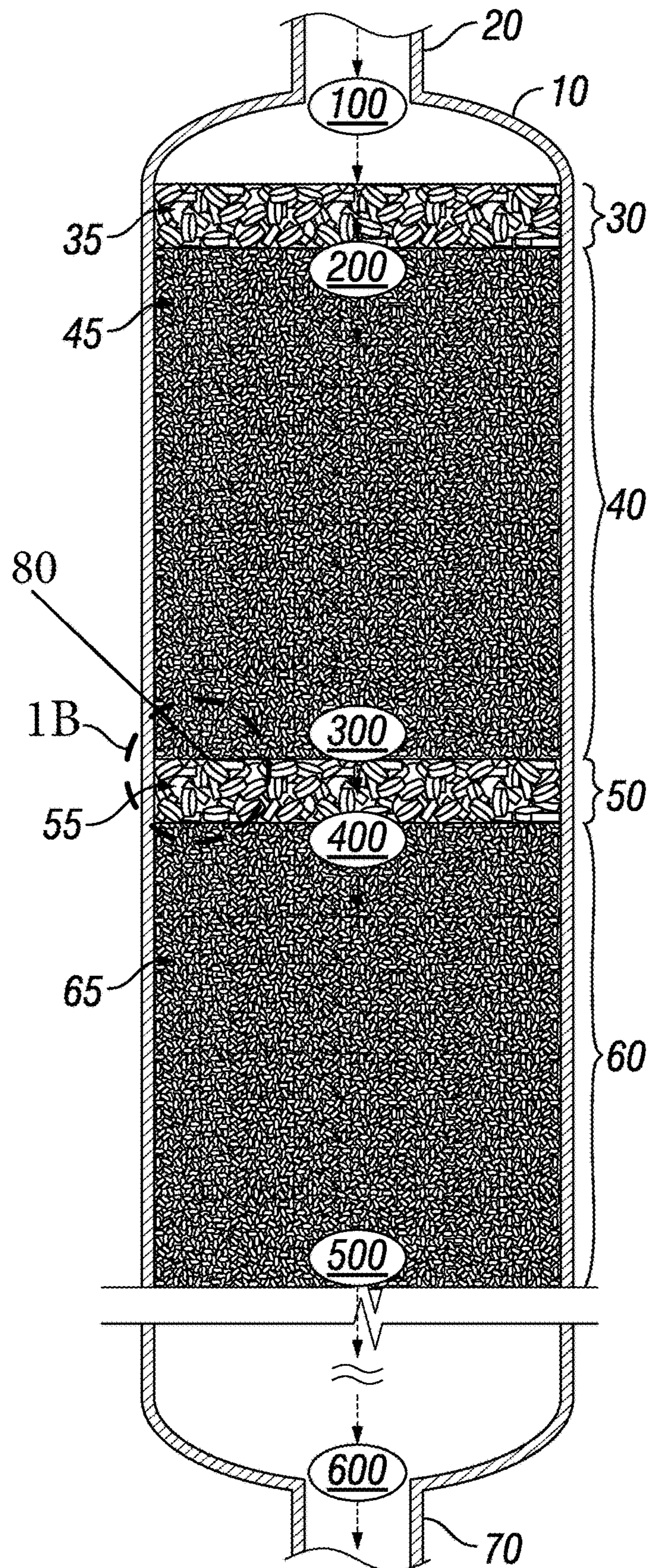
FIG. 1A
