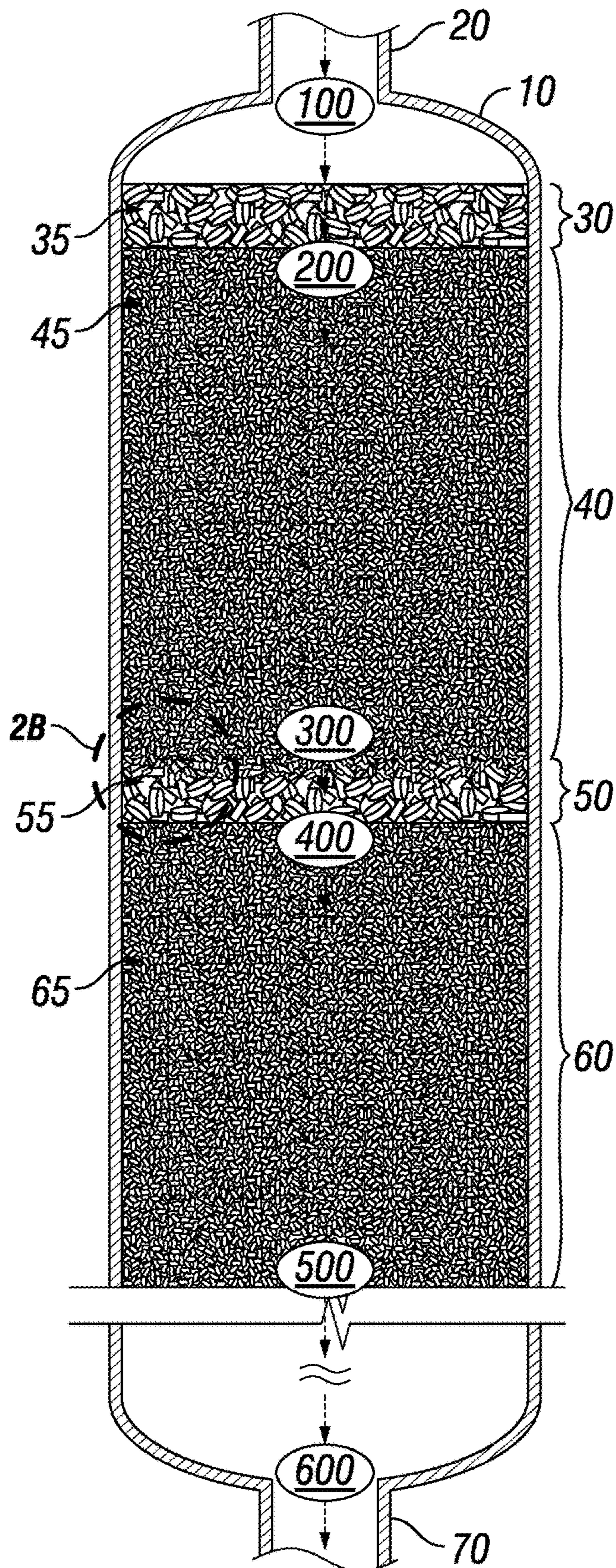
FIG. 2A
