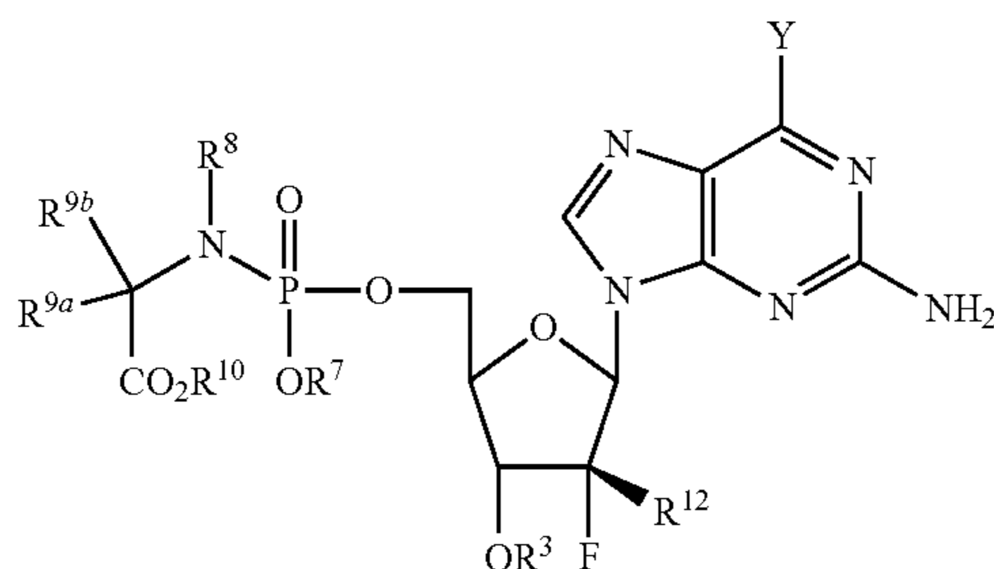
Formula Ic
