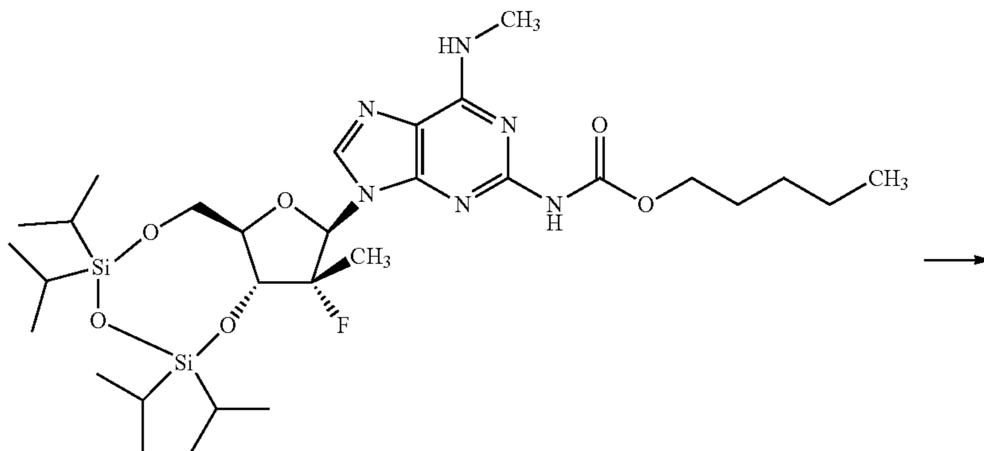
54
