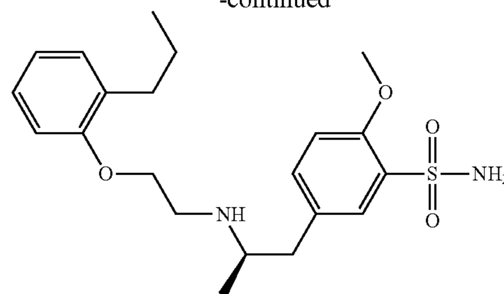
(R)-5-(2-(2-(2-ethoxyphenoxy)ethylamino)propyl)-2-methoxybenzenesulfonamide
