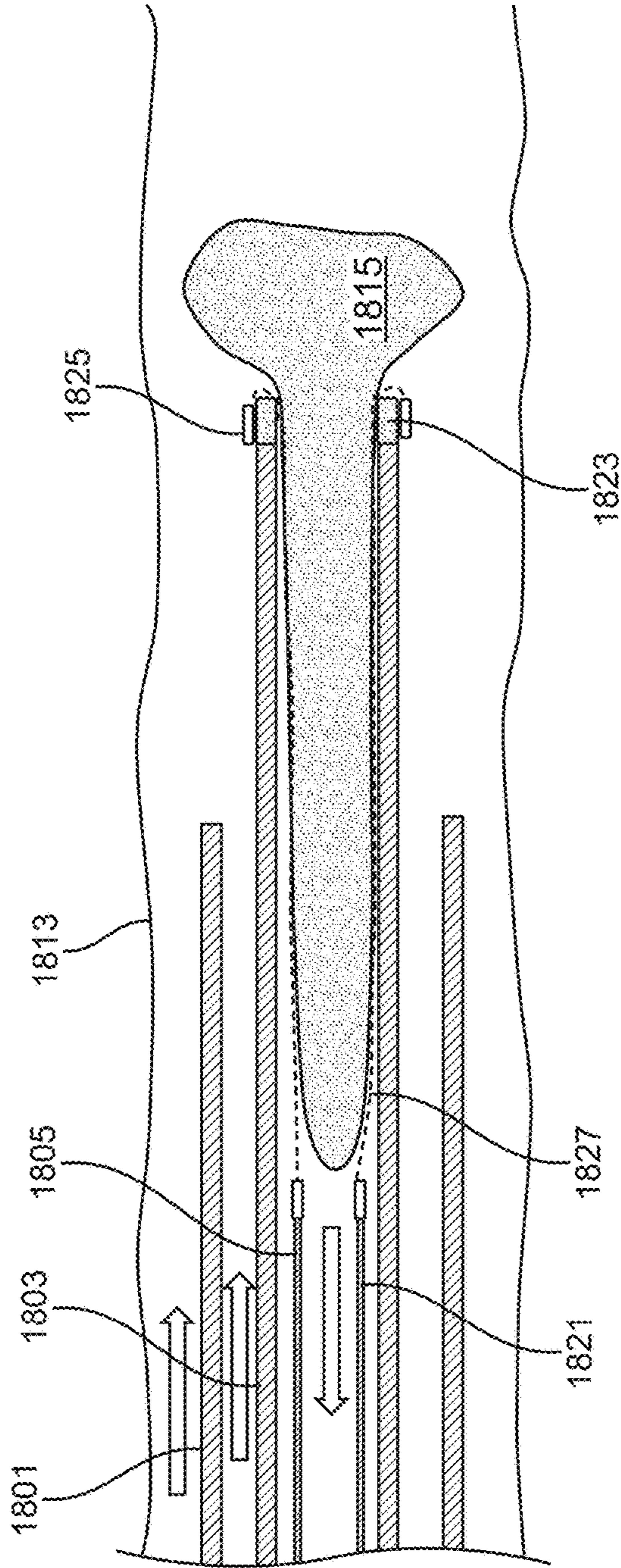
FIG. 18H
