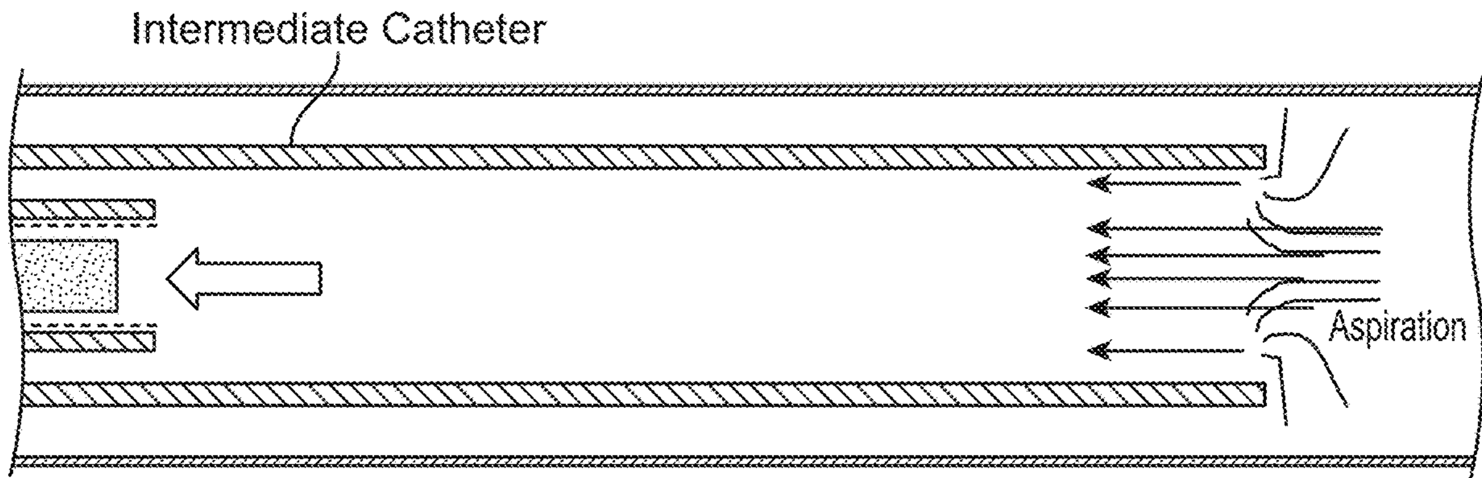
FIG. 9J
