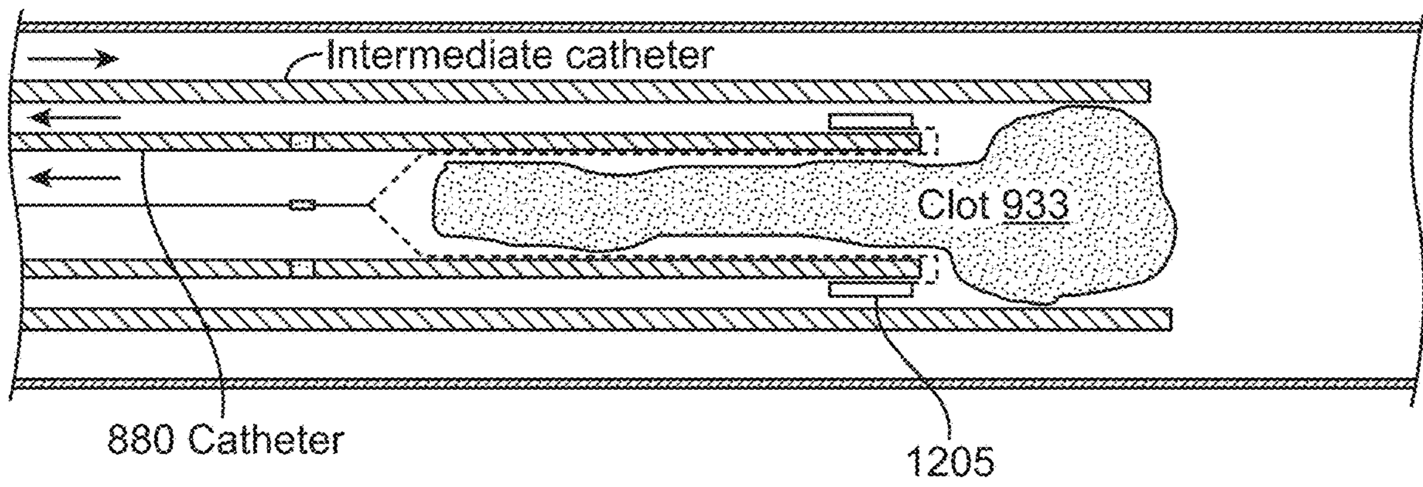
FIG. 12A
