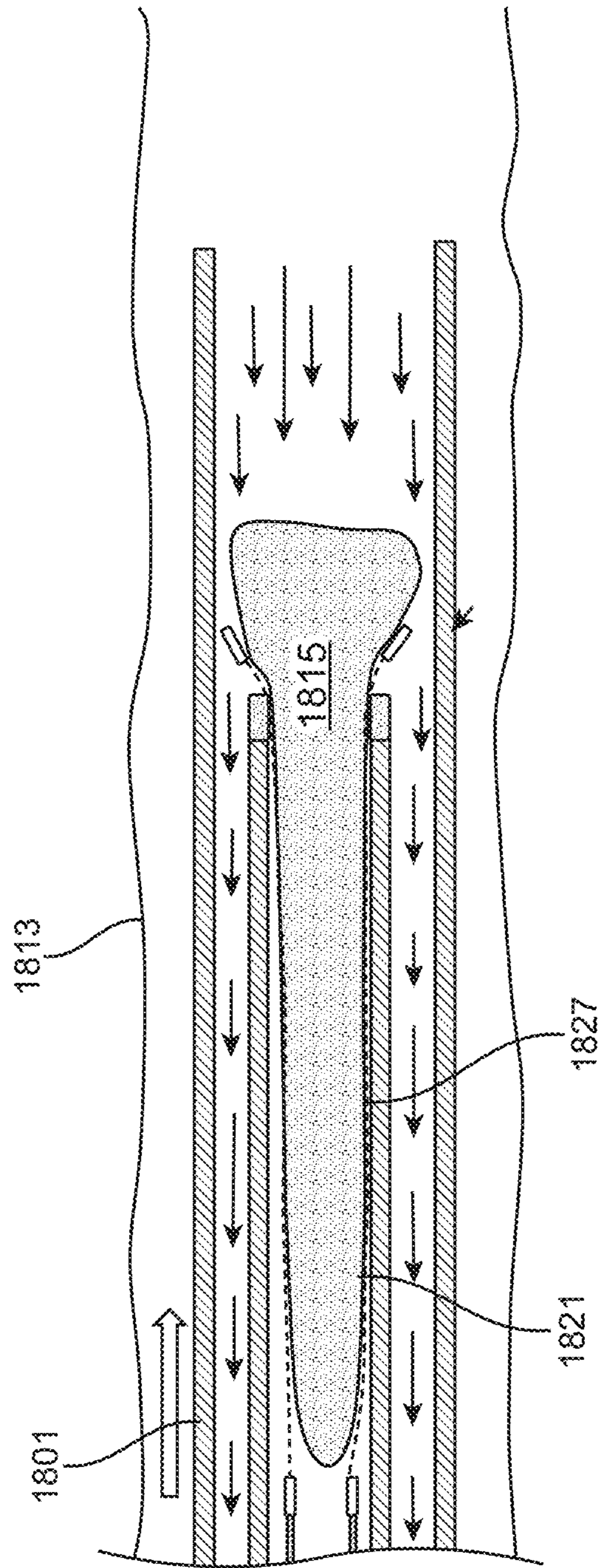
FIG. 18J
