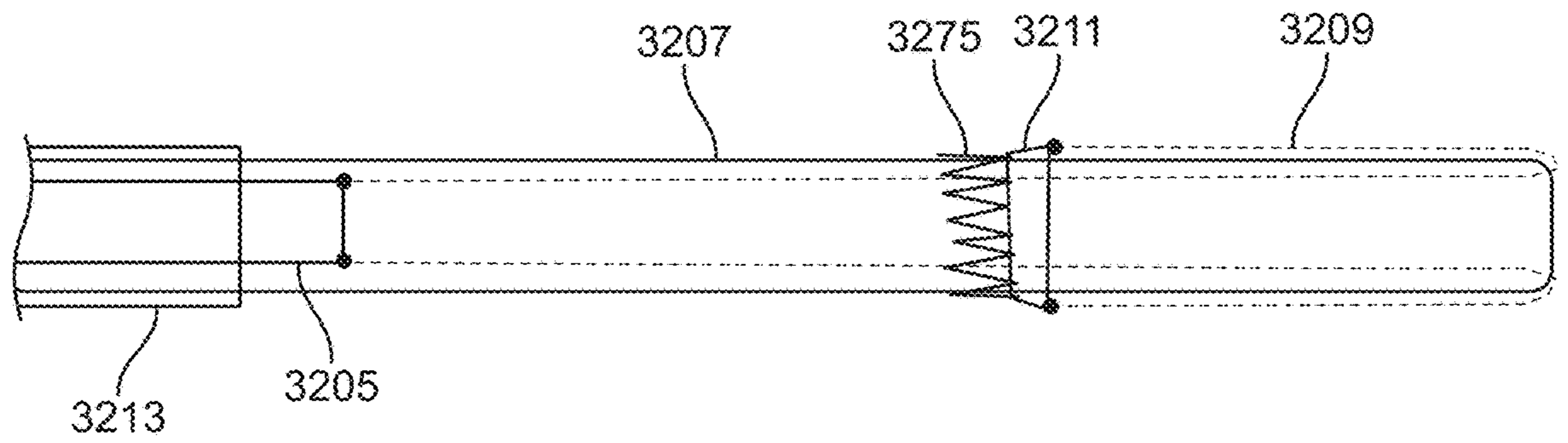
FIG. 32F
