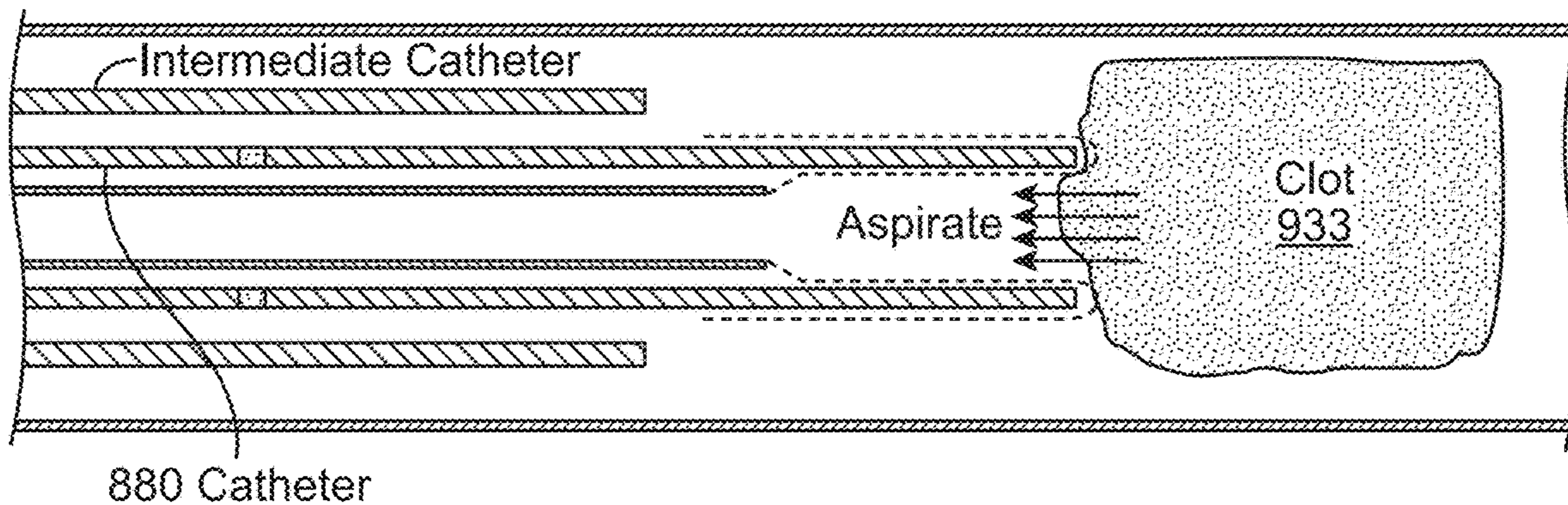
FIG. 9D
