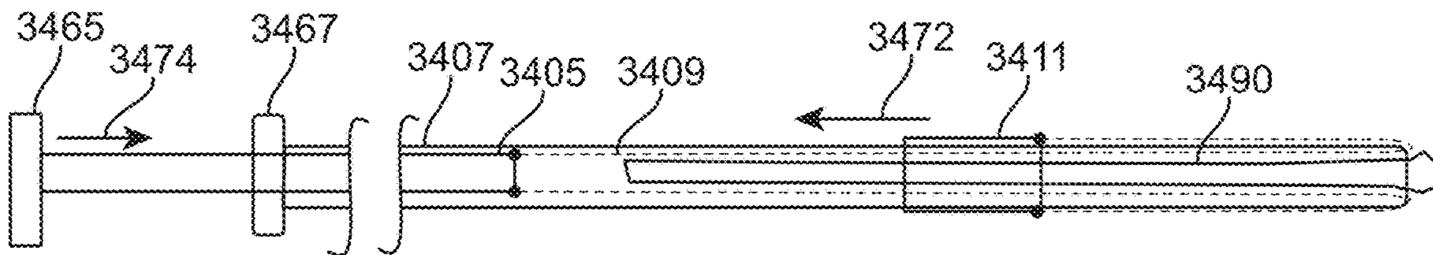
FIG. 34B
