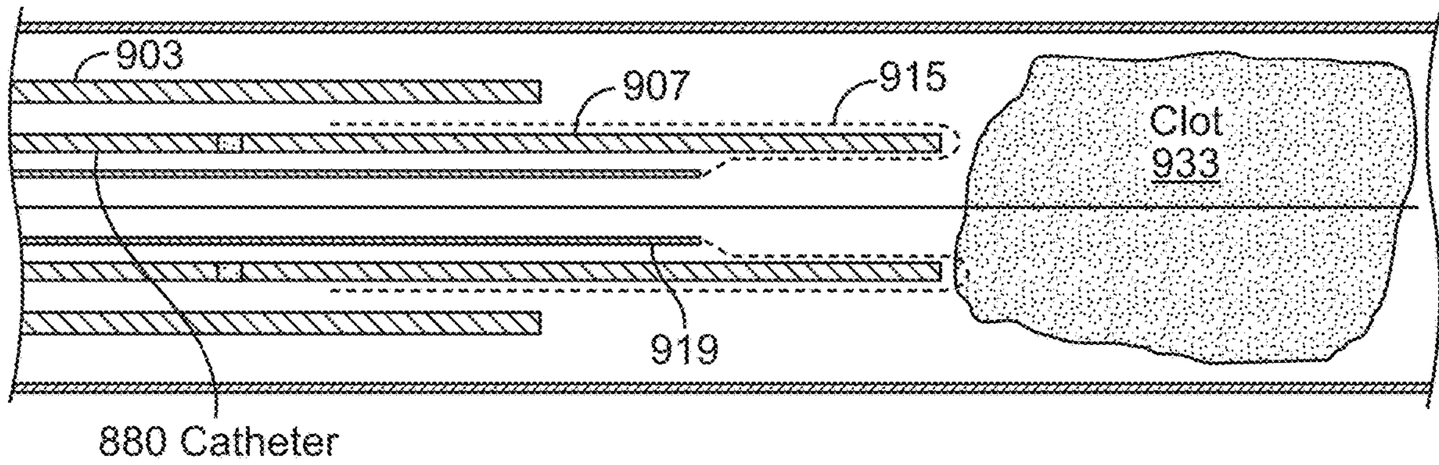
FIG. 9B
