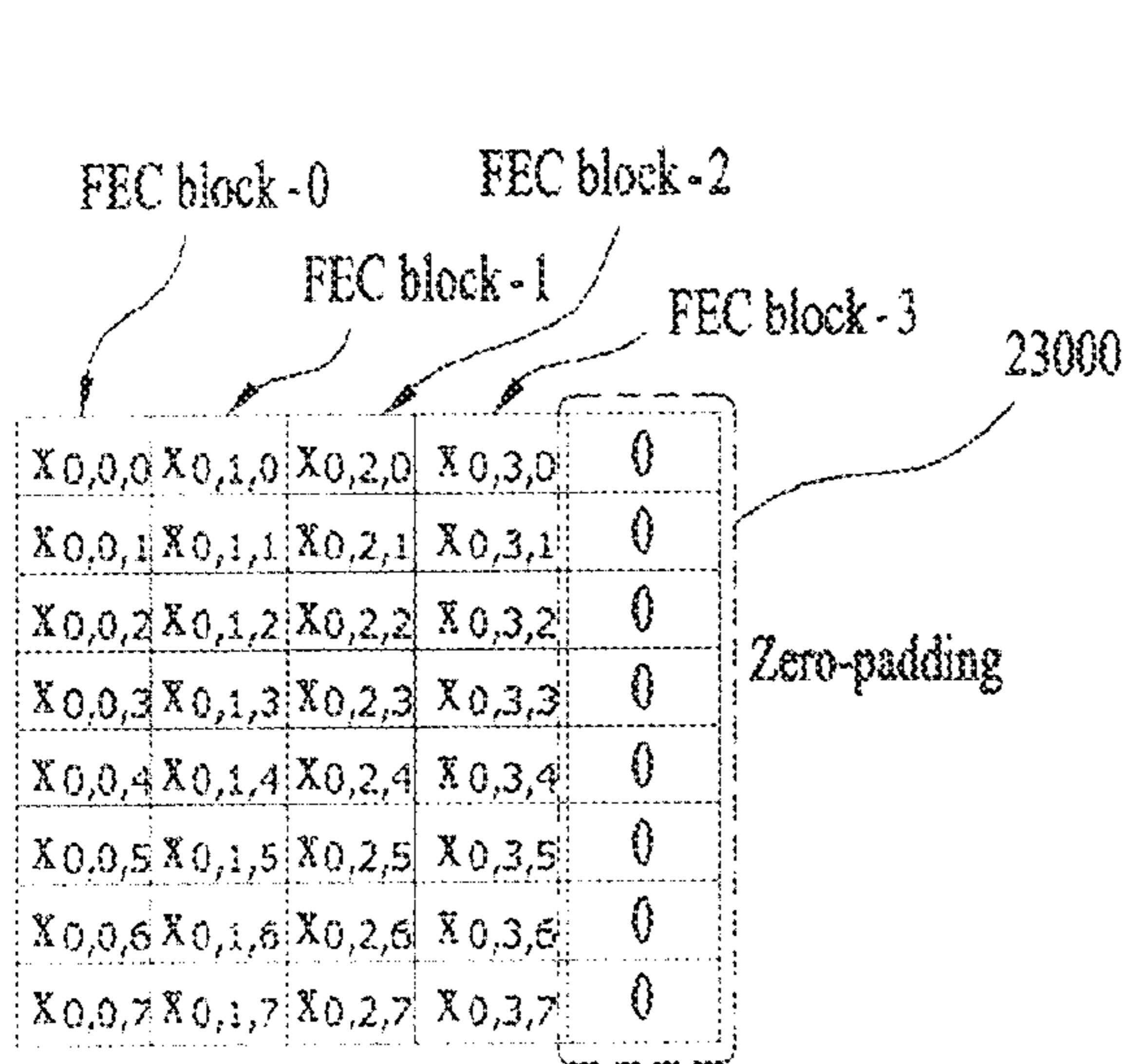
[TI FEC blocks]
