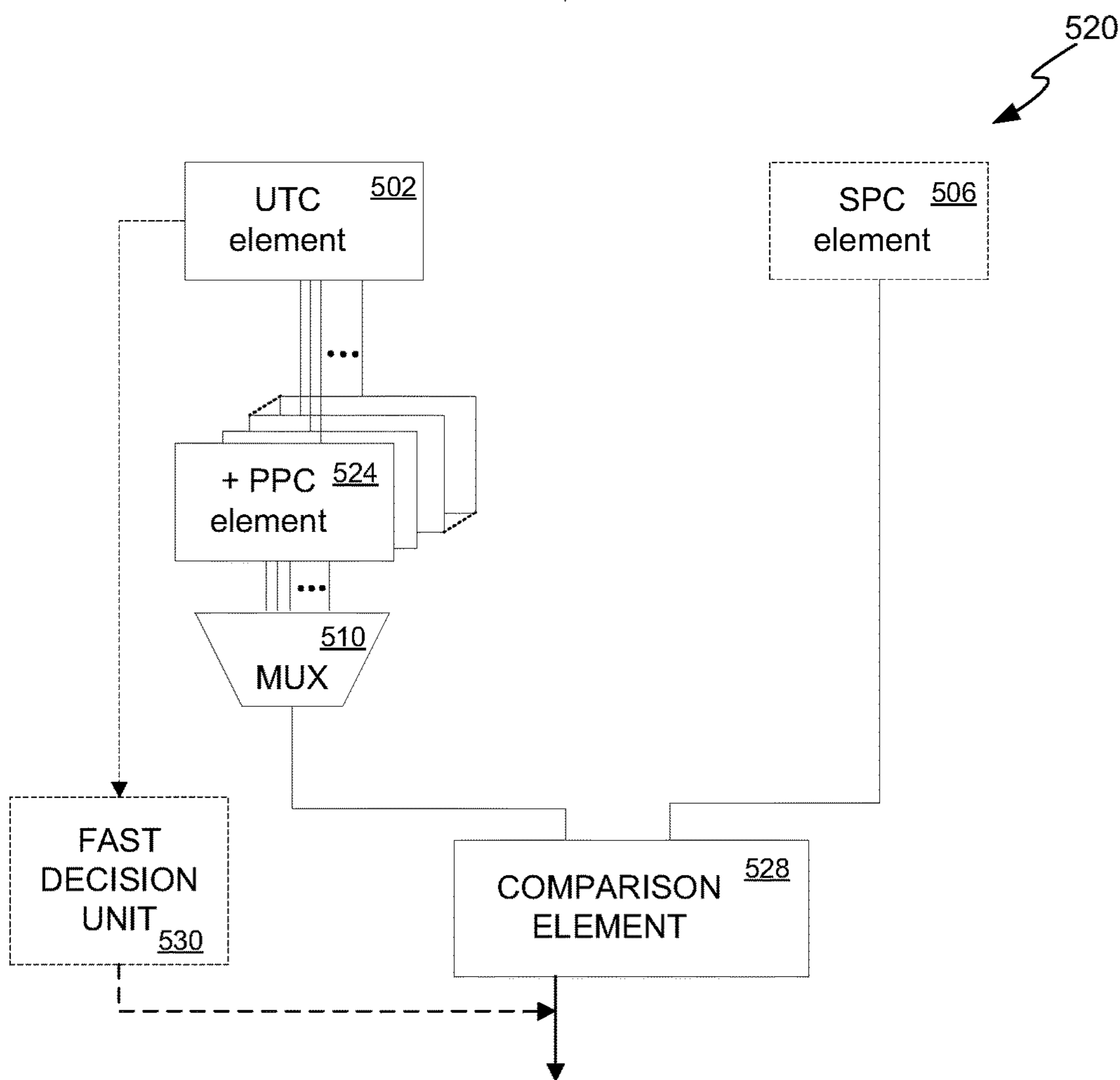
FIG. 5B
