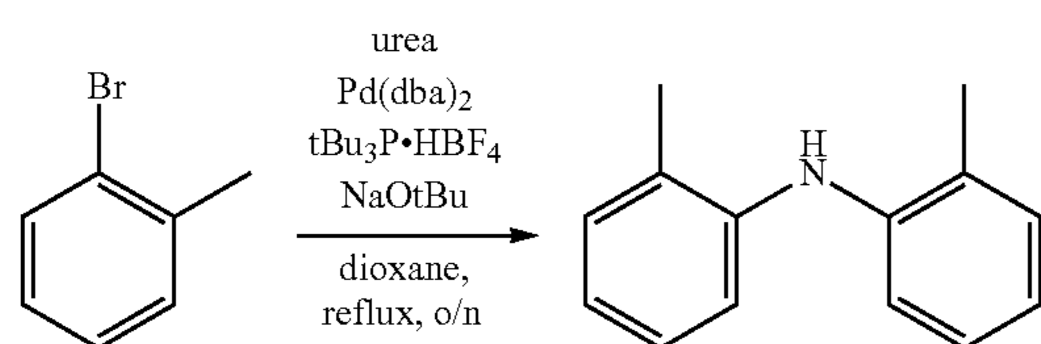
Bis(o-tolyl)amine
