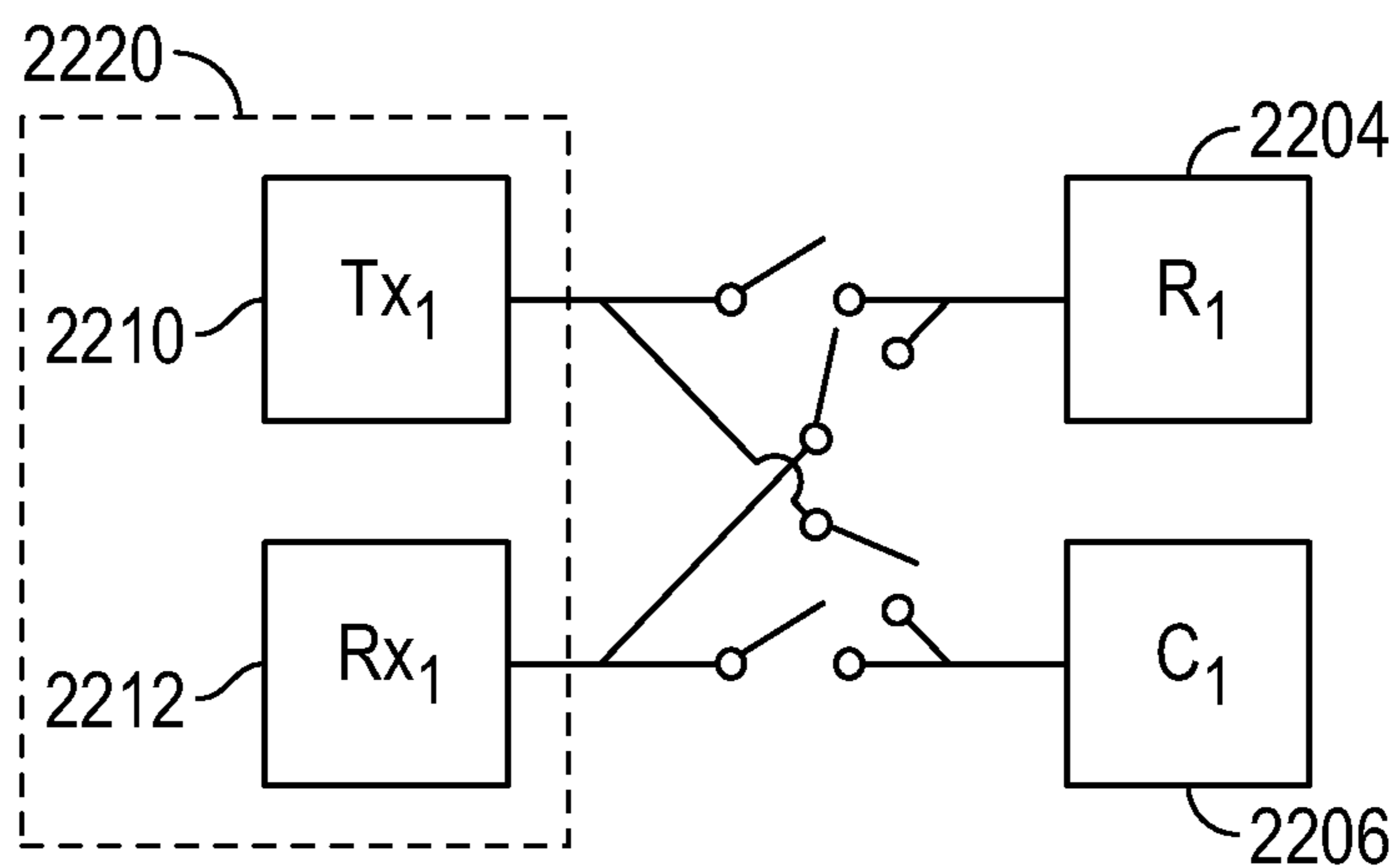
FIG. 22B
