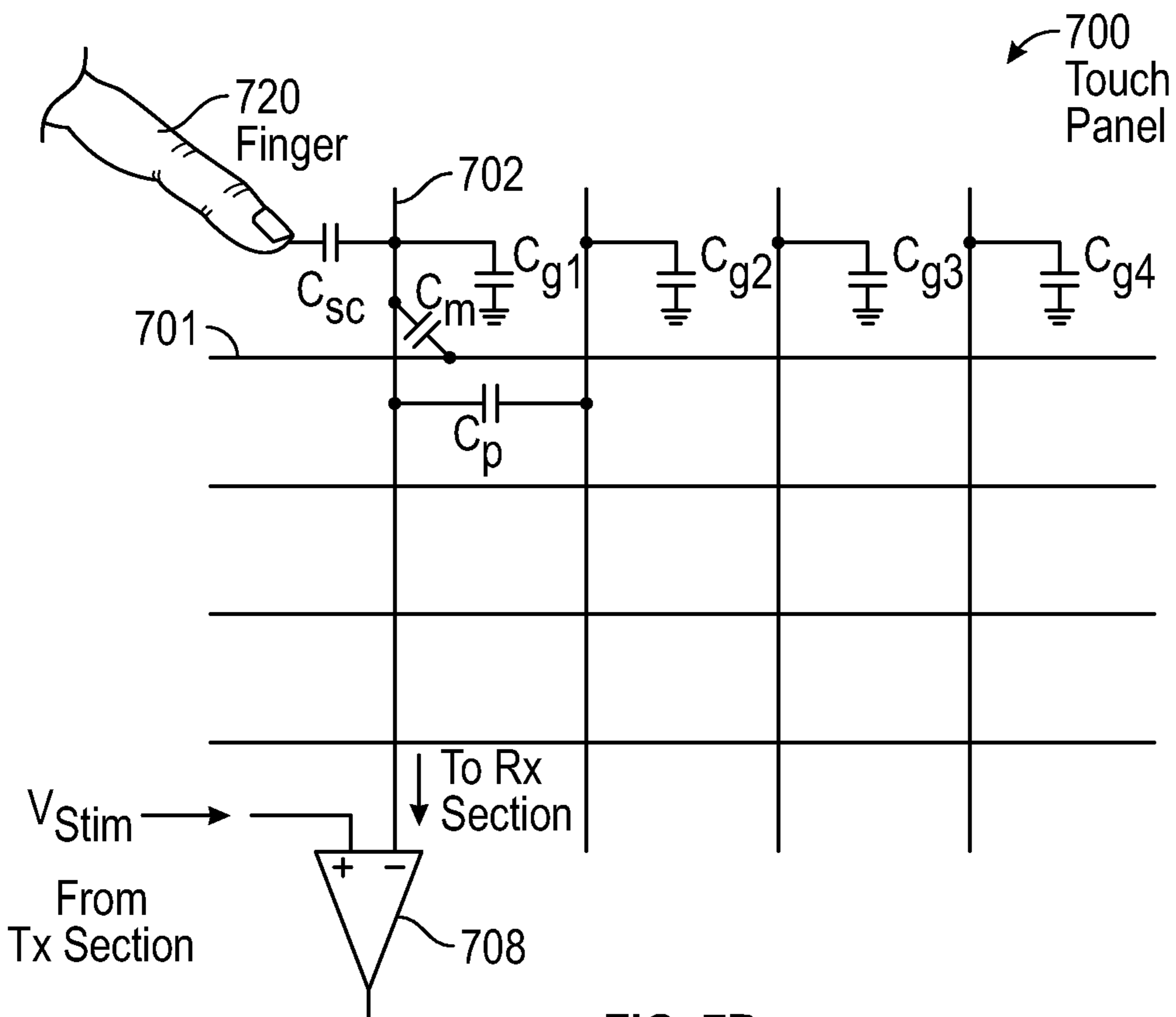
FIG. 7B
