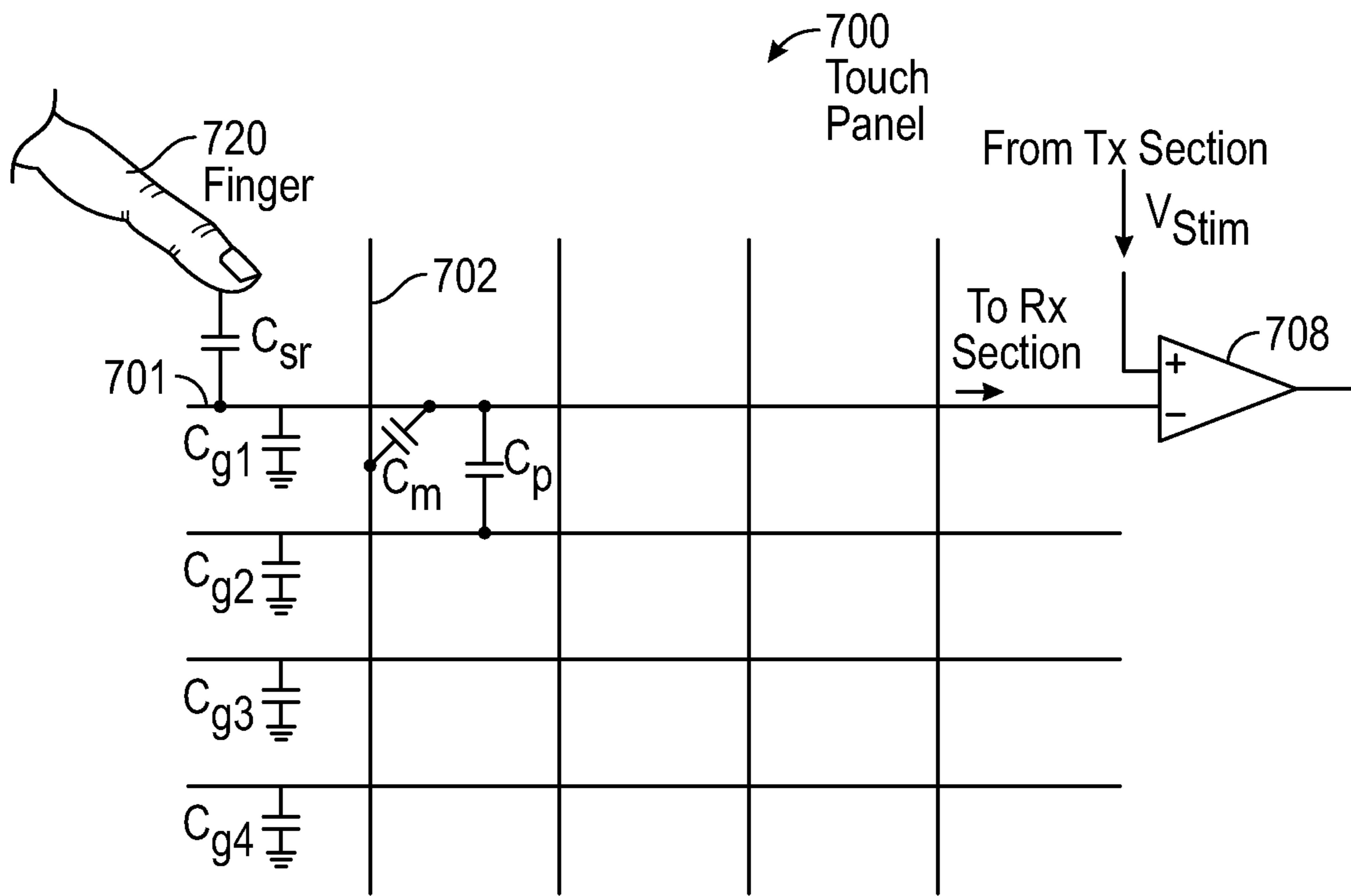
FIG. 7A
