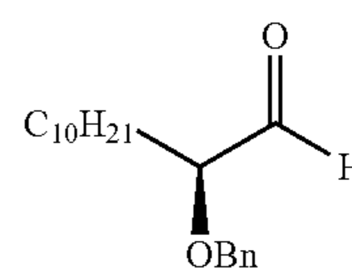
(S)-2-(benzyloxy)dodecanal (404)
