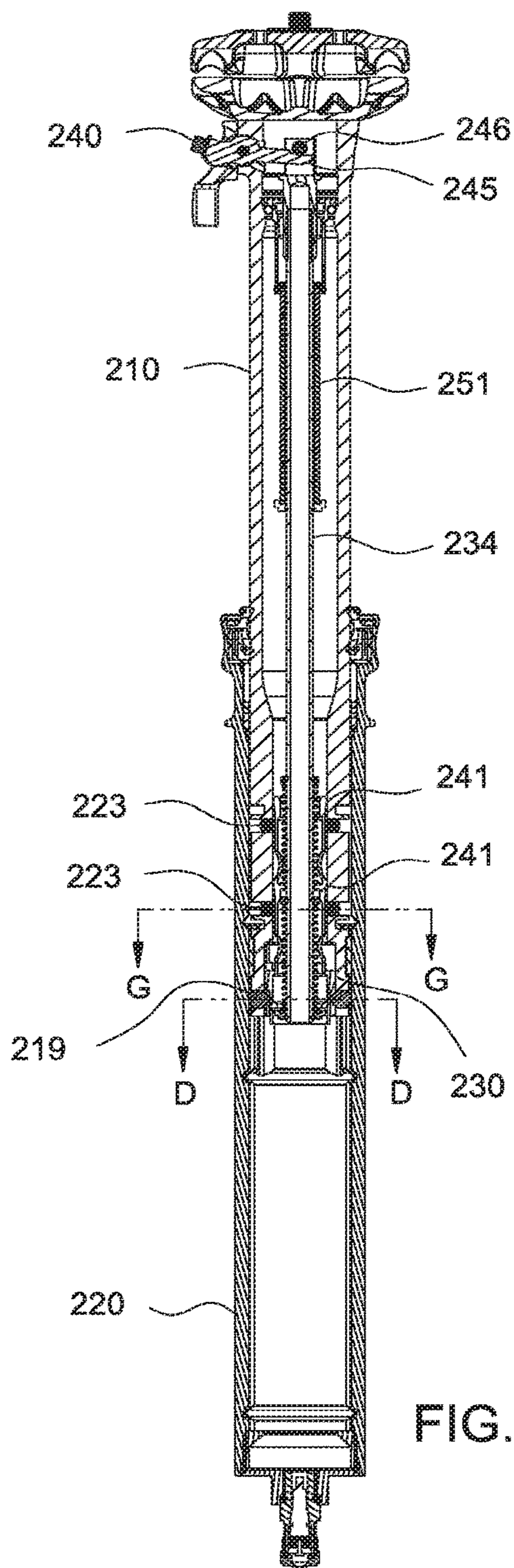
SECTION A-A
