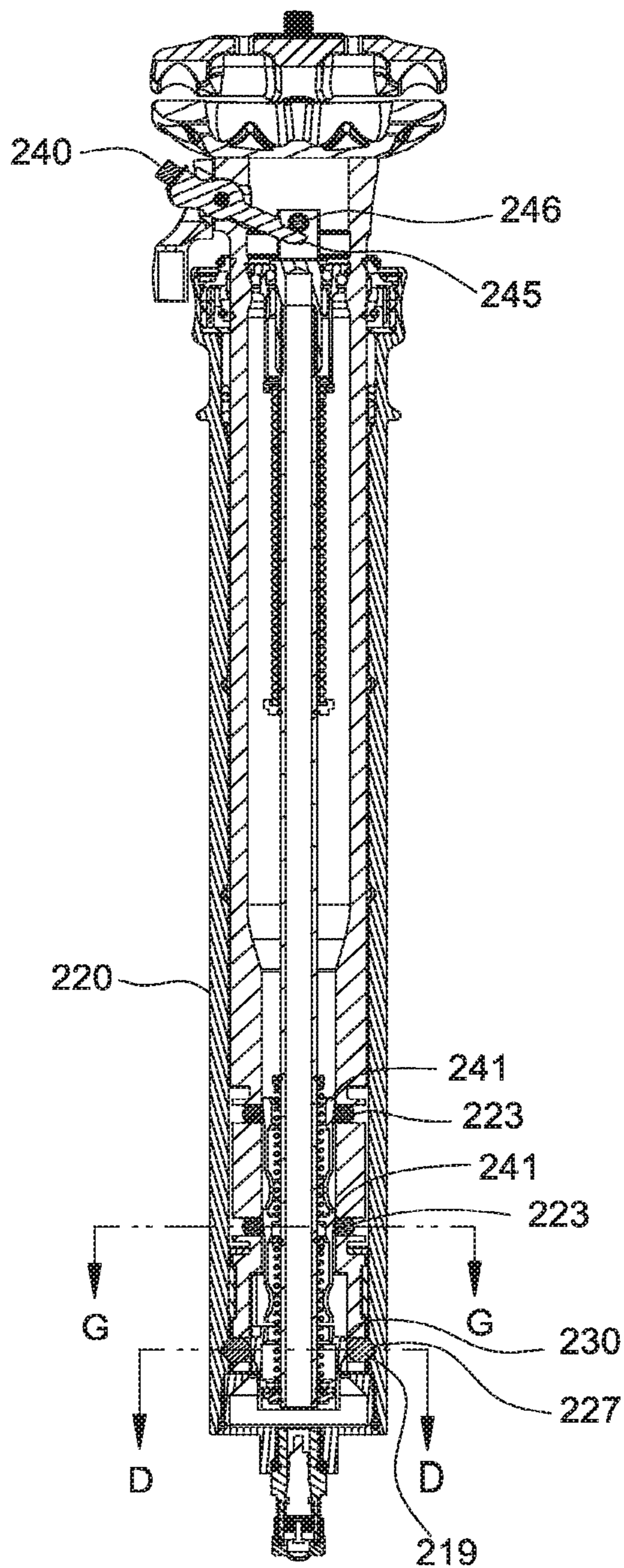
SECTION A-A
