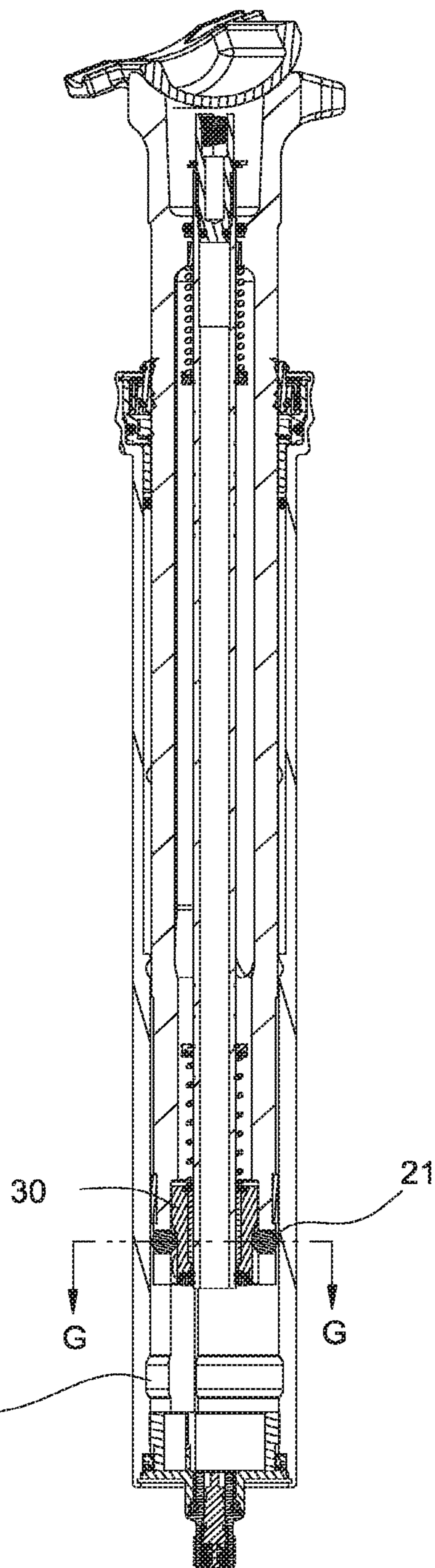
SECTION D-D
