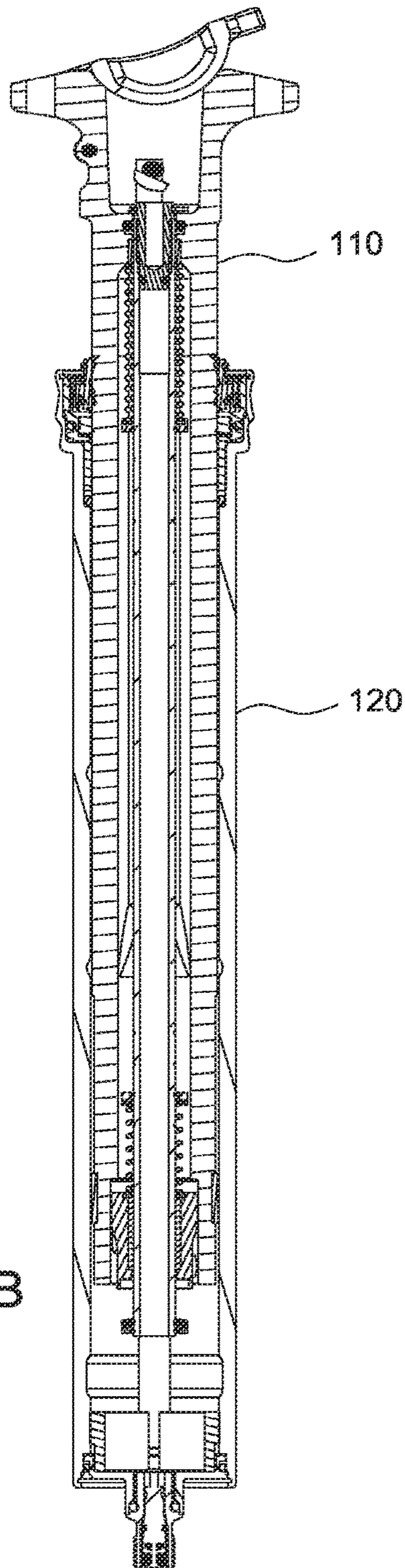
SECTION A-A
