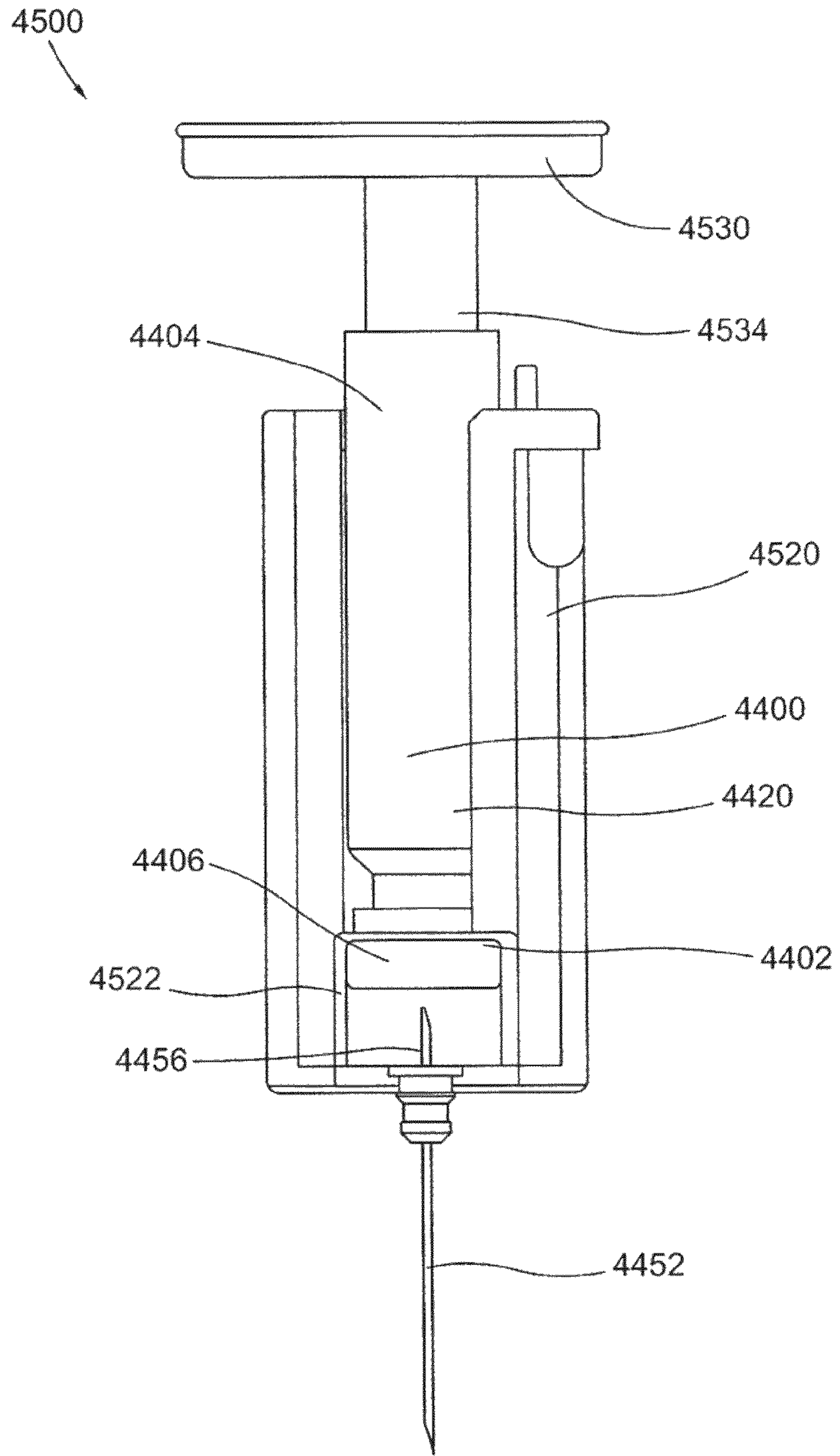
FIG. 25
