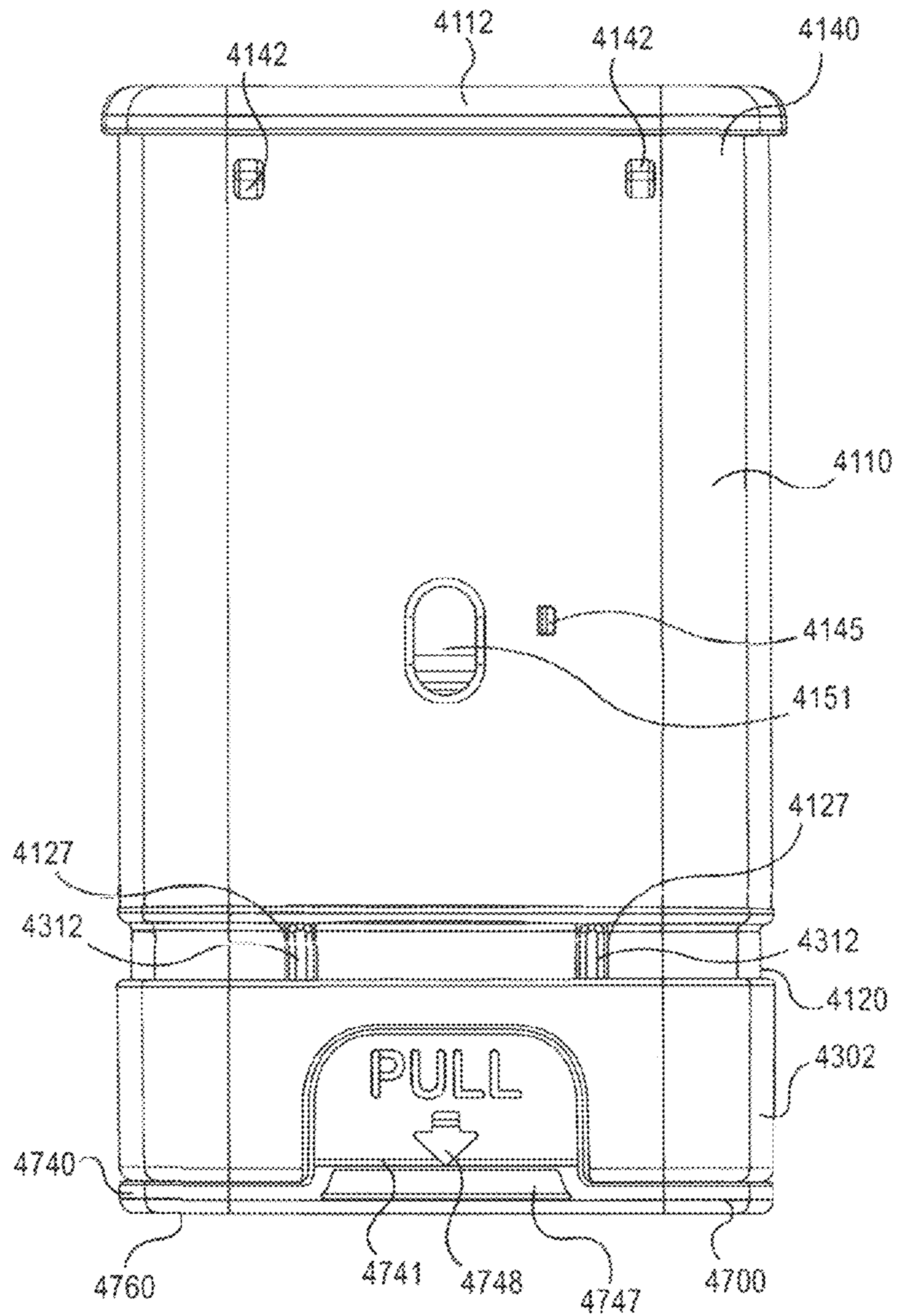
FIG. 15
