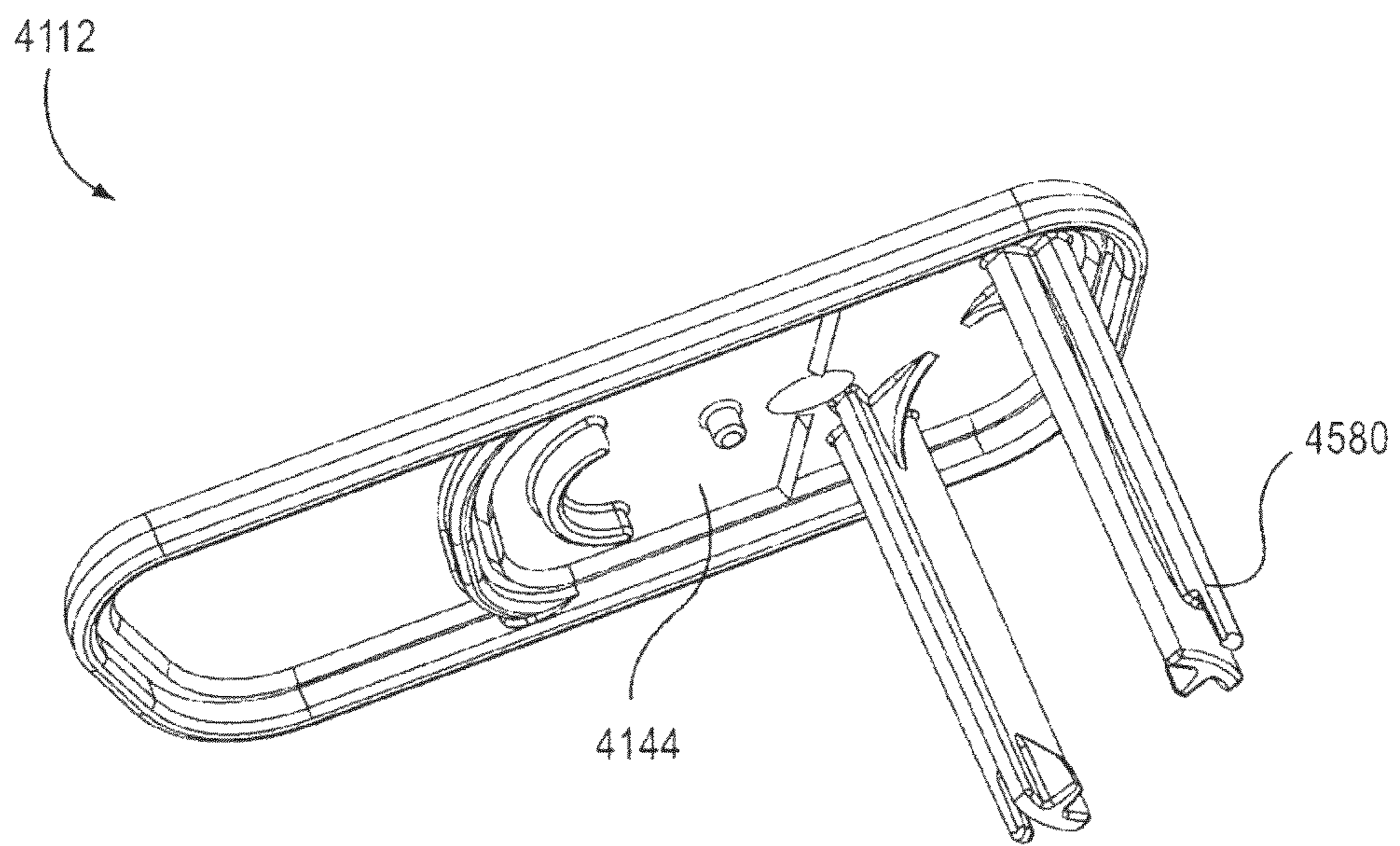
FIG. 20
