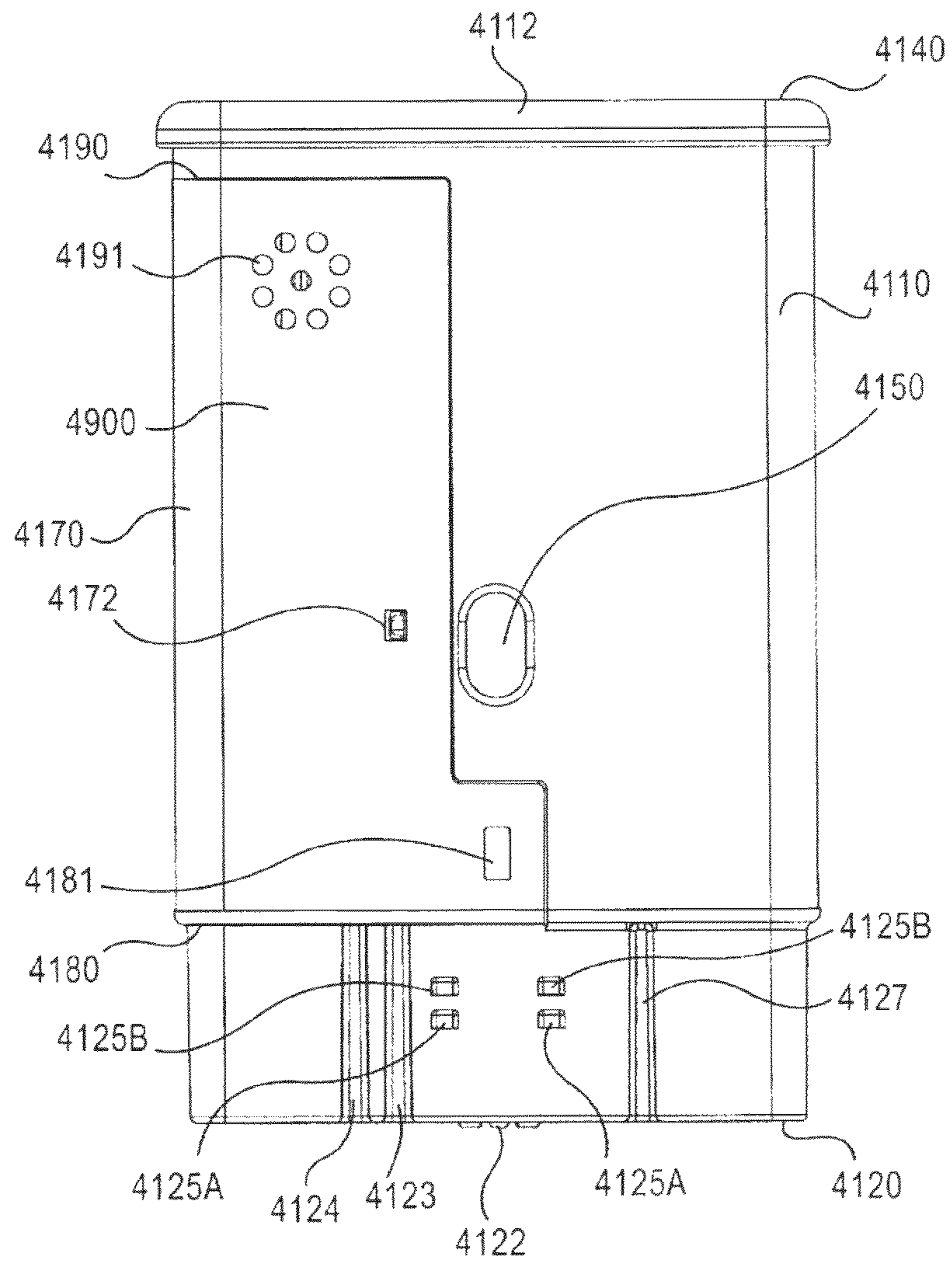
FIG. 16
