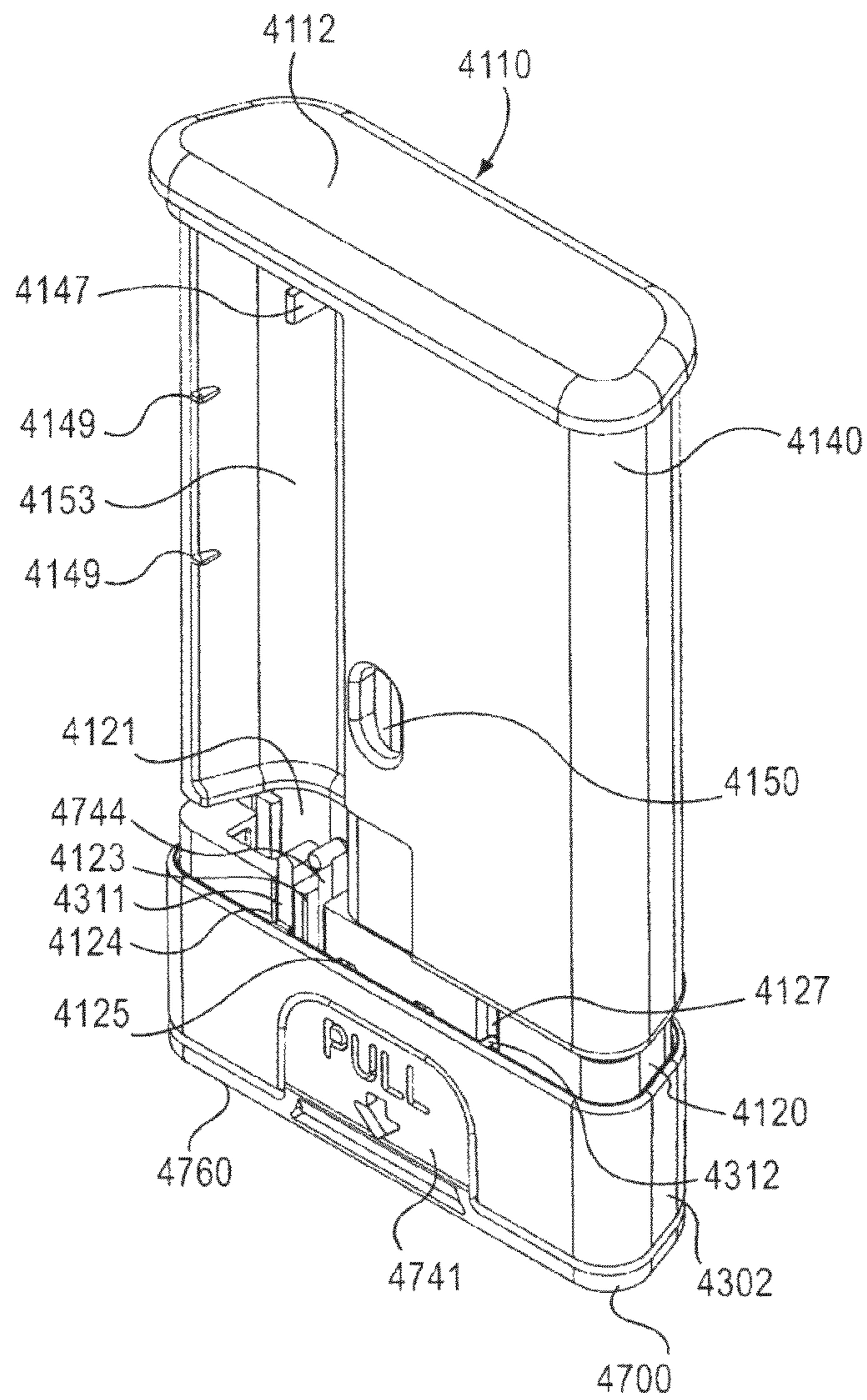
FIG. 17
