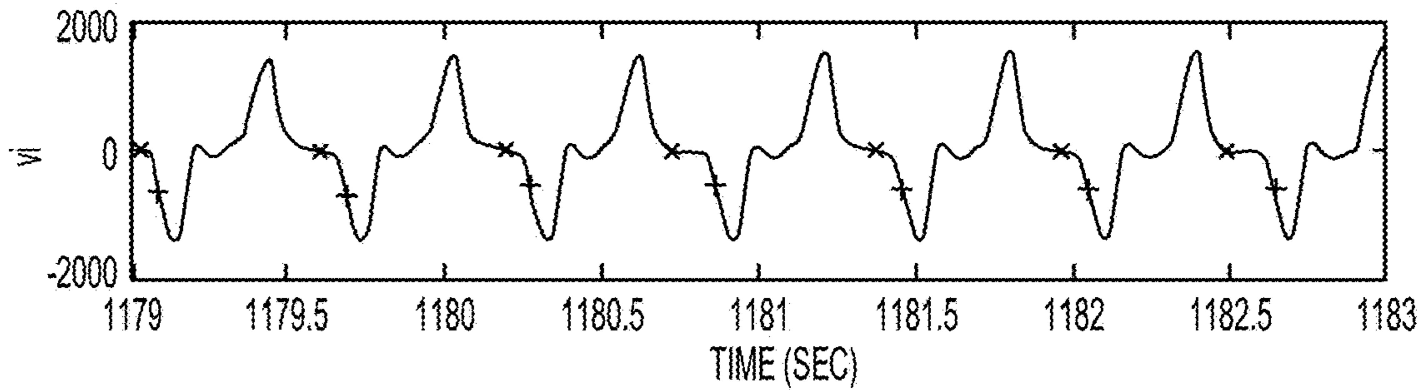
FIG. 7C
