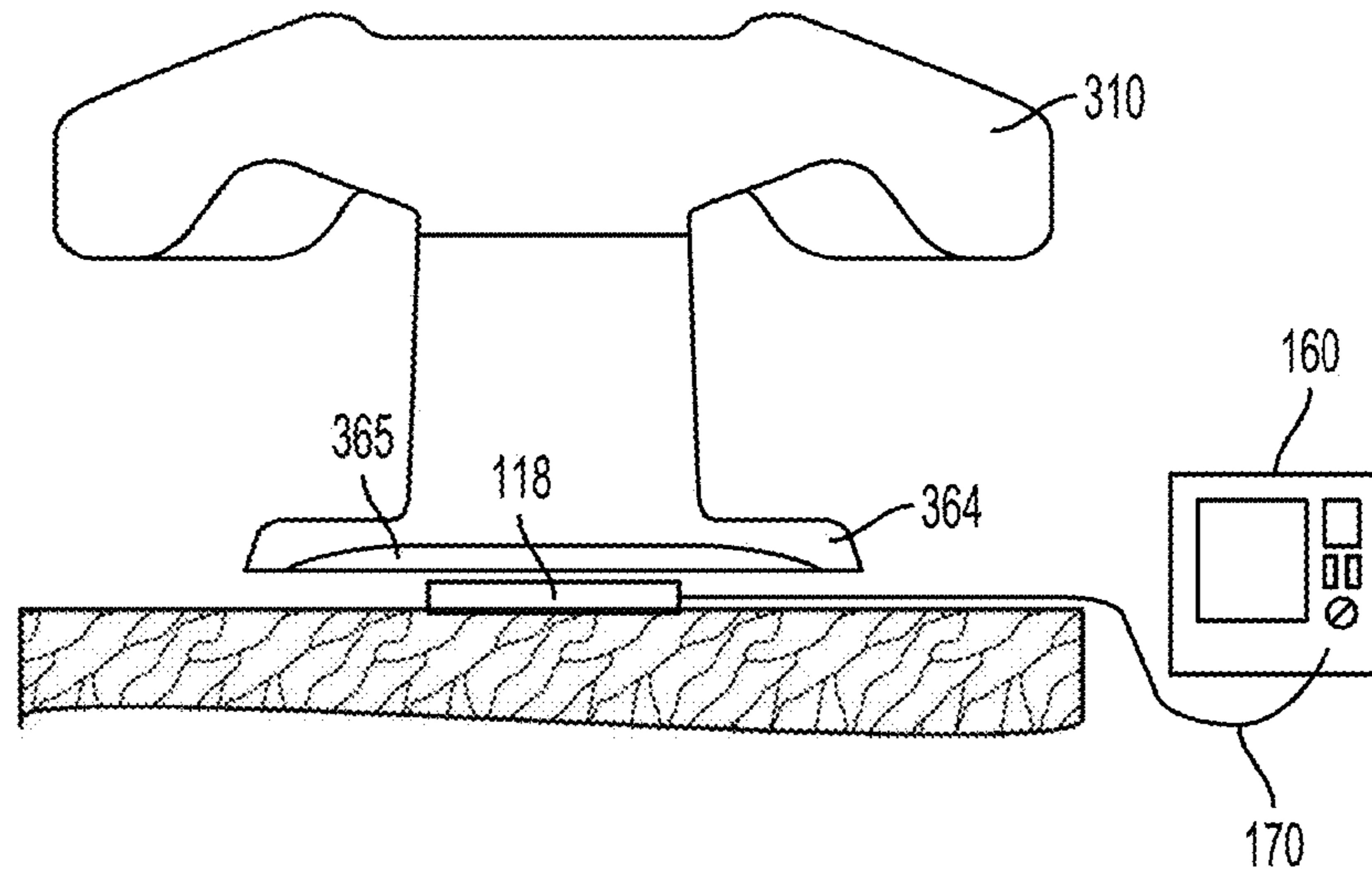
FIG. 3C
