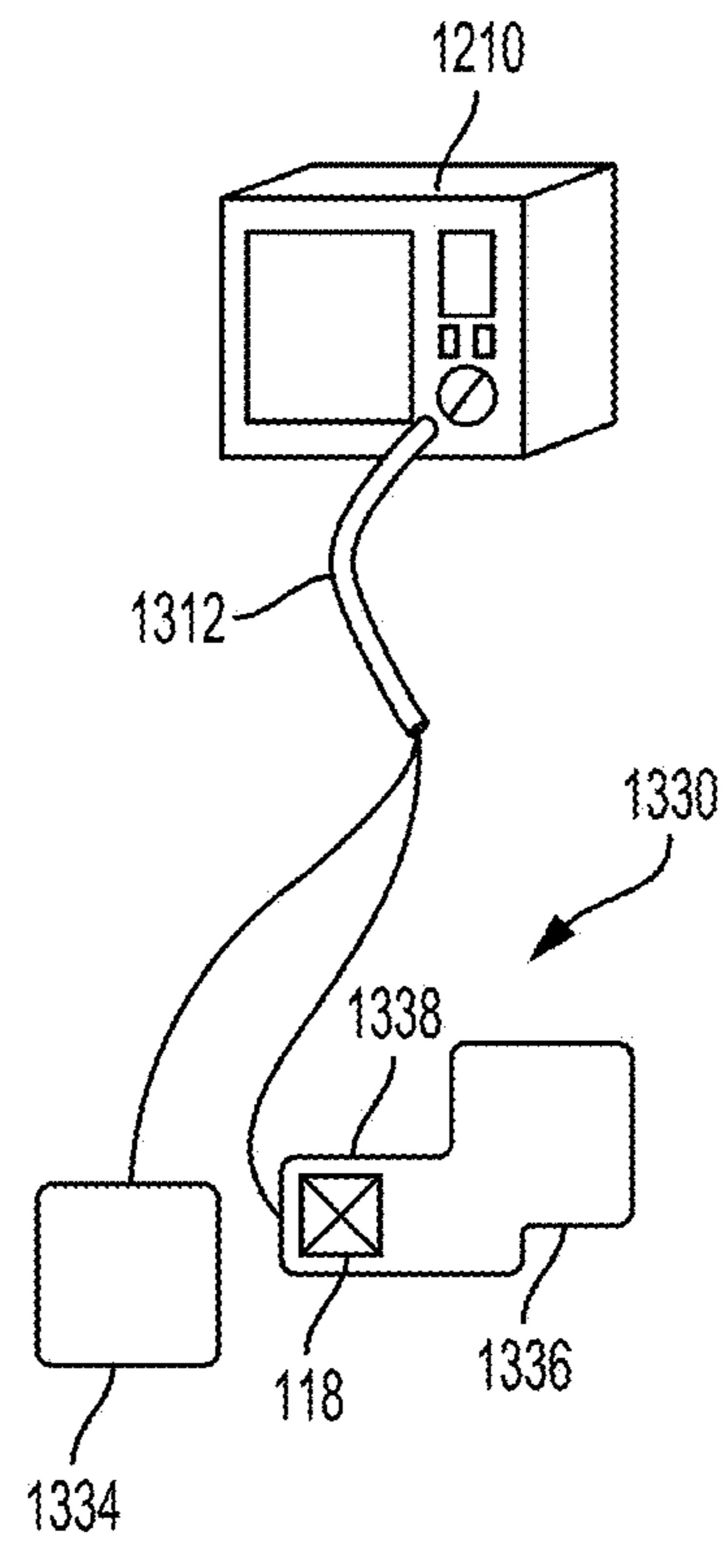
FIG. 13B
