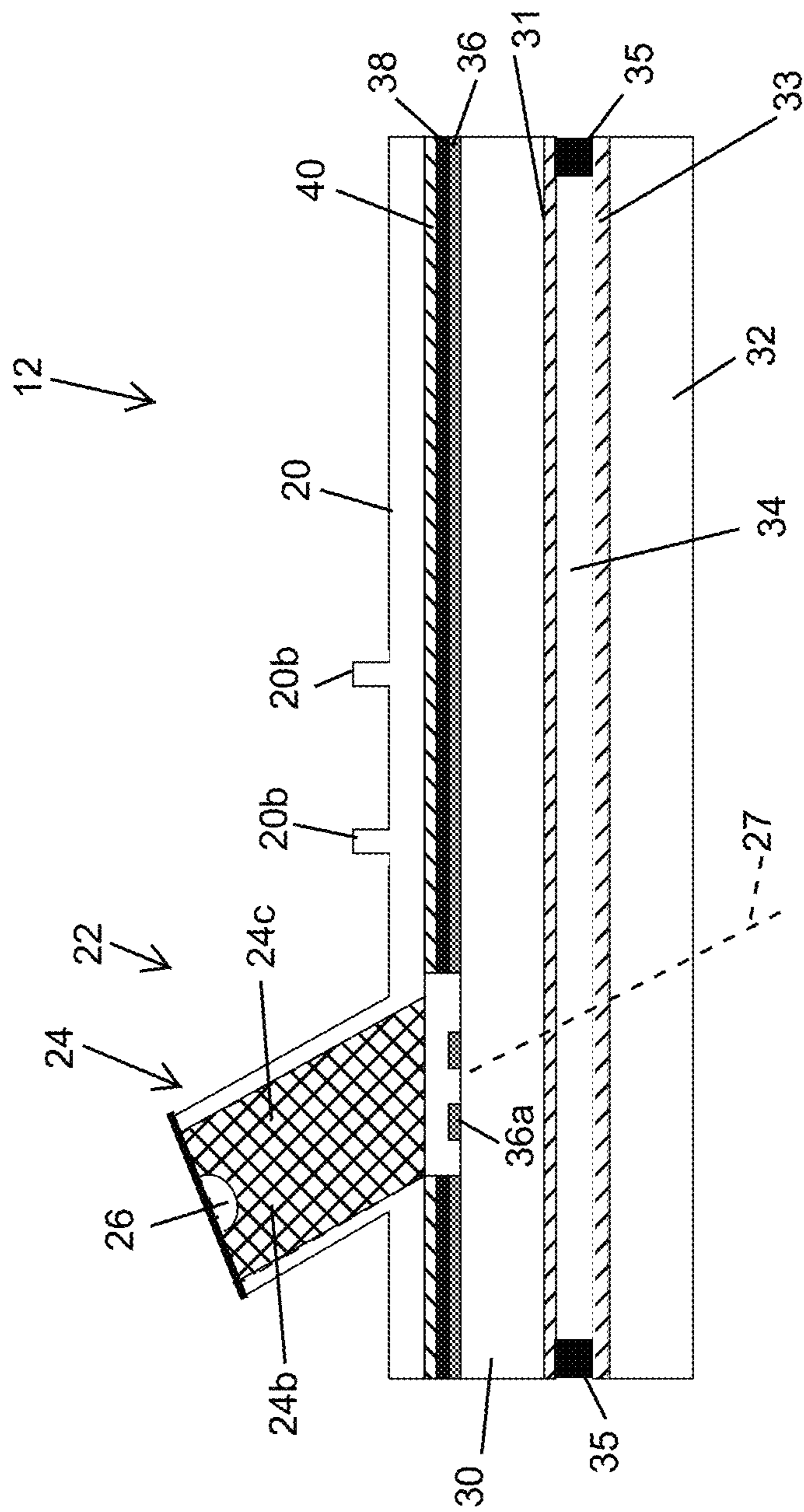
FIG. 3A
