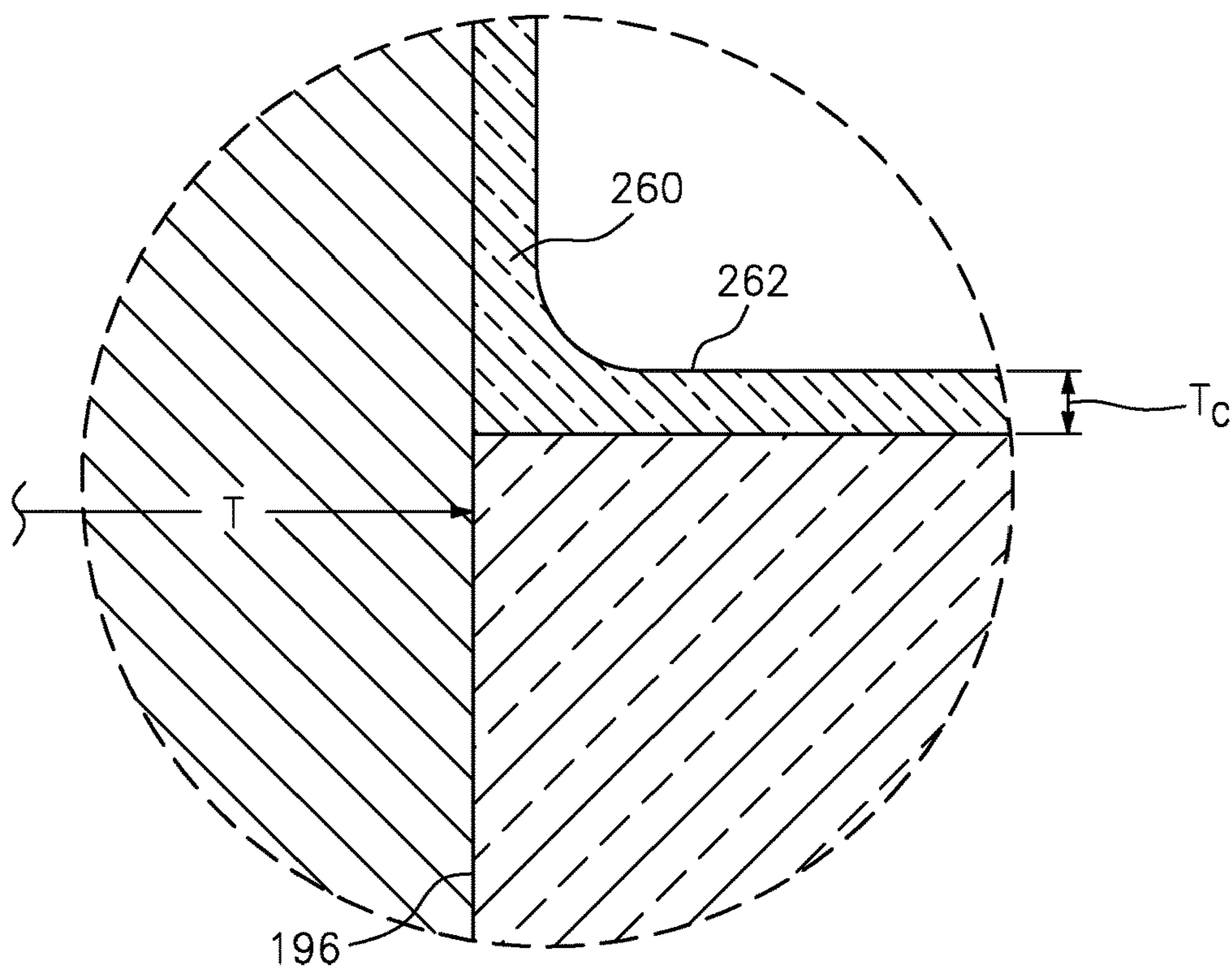
FIG. 6A
