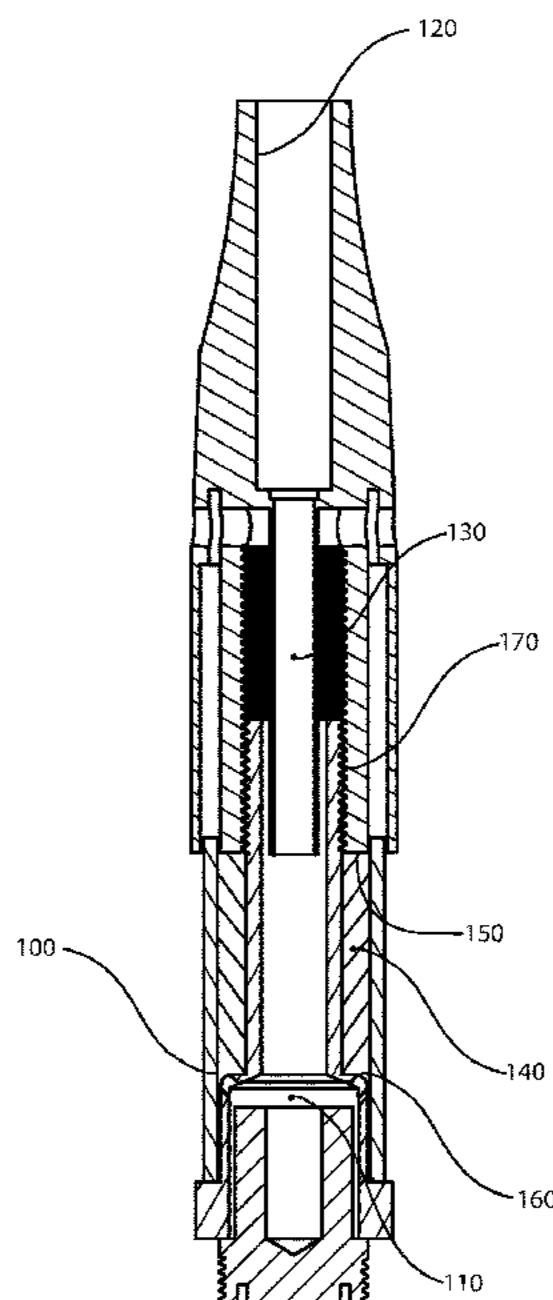
A-A (3:1)
