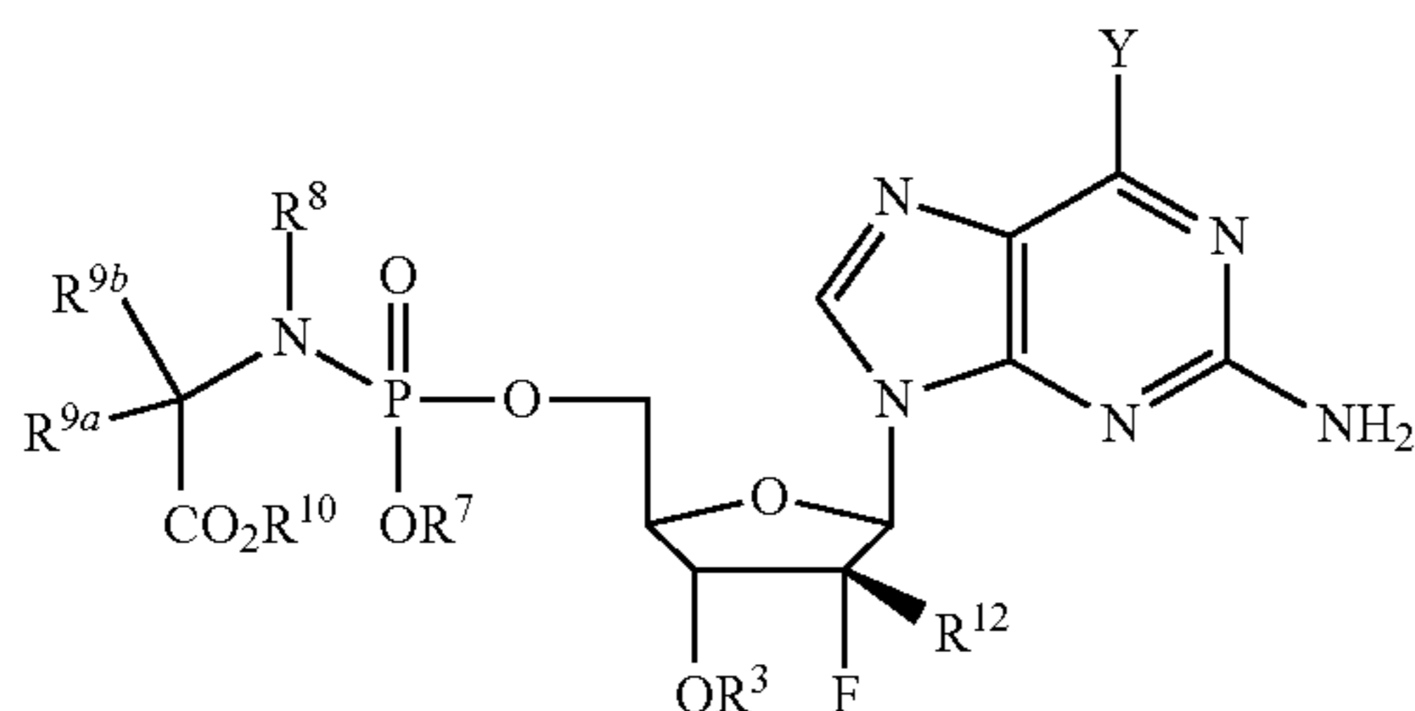
Formula Ic
