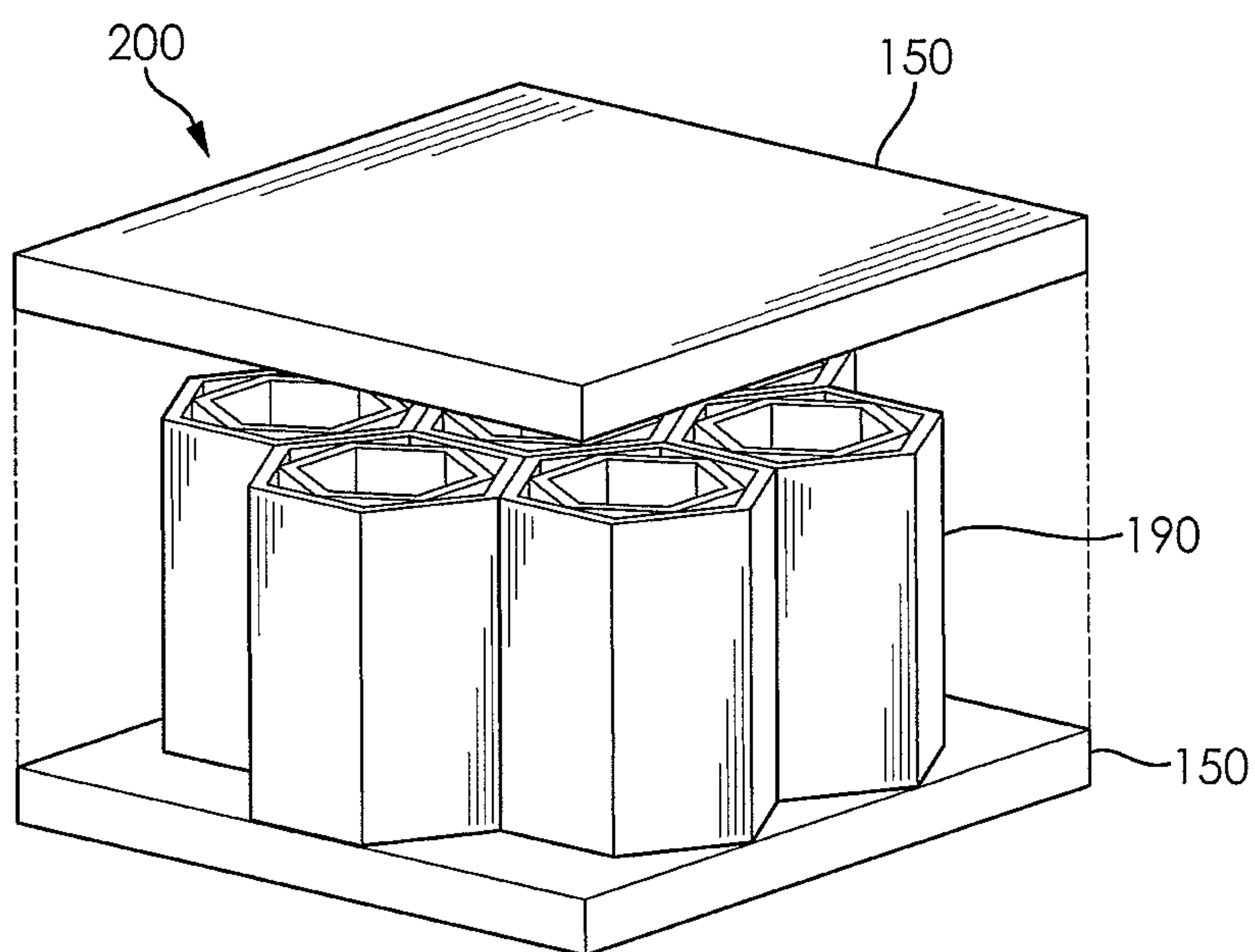
FIG. 9C
