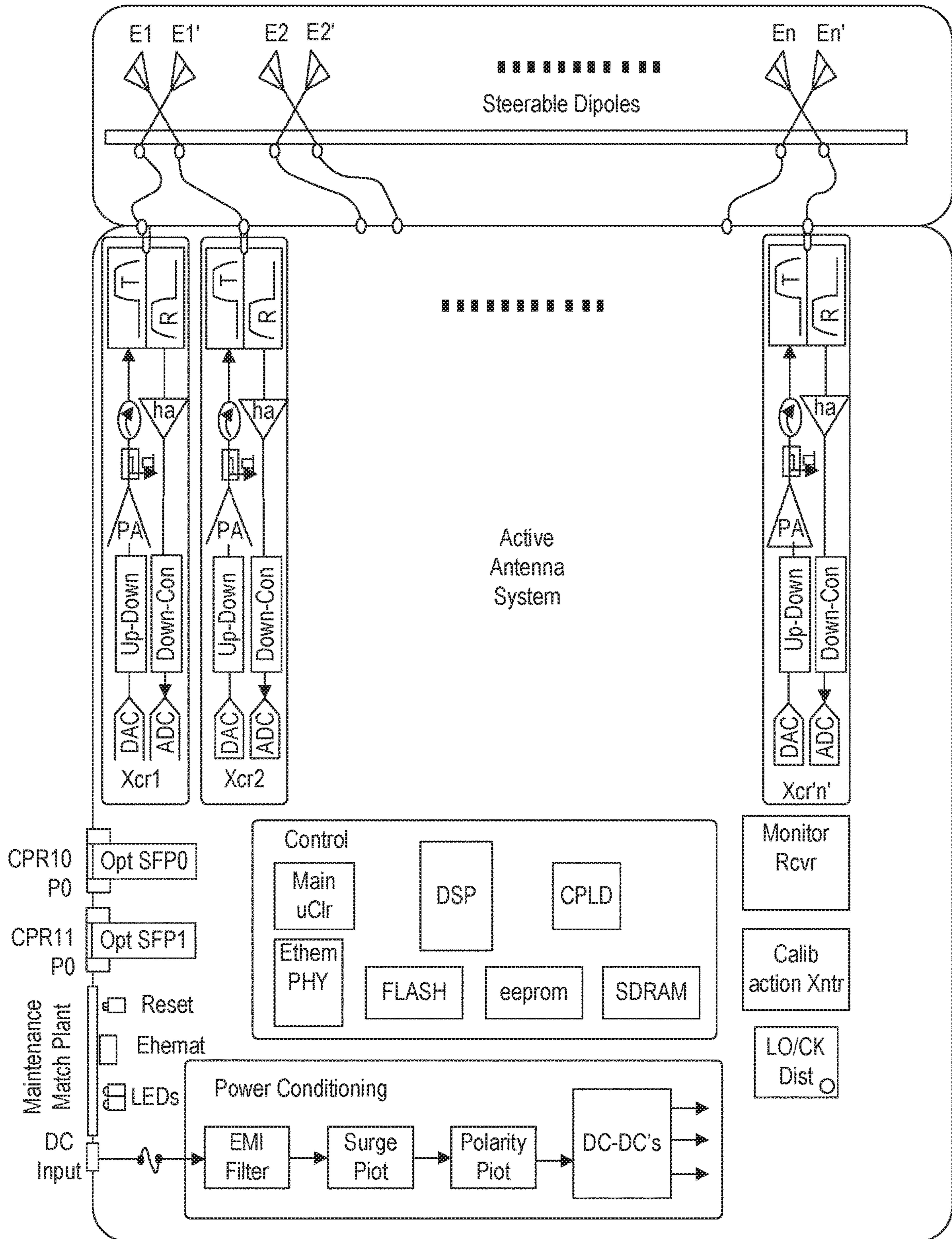
FIG. 2H
